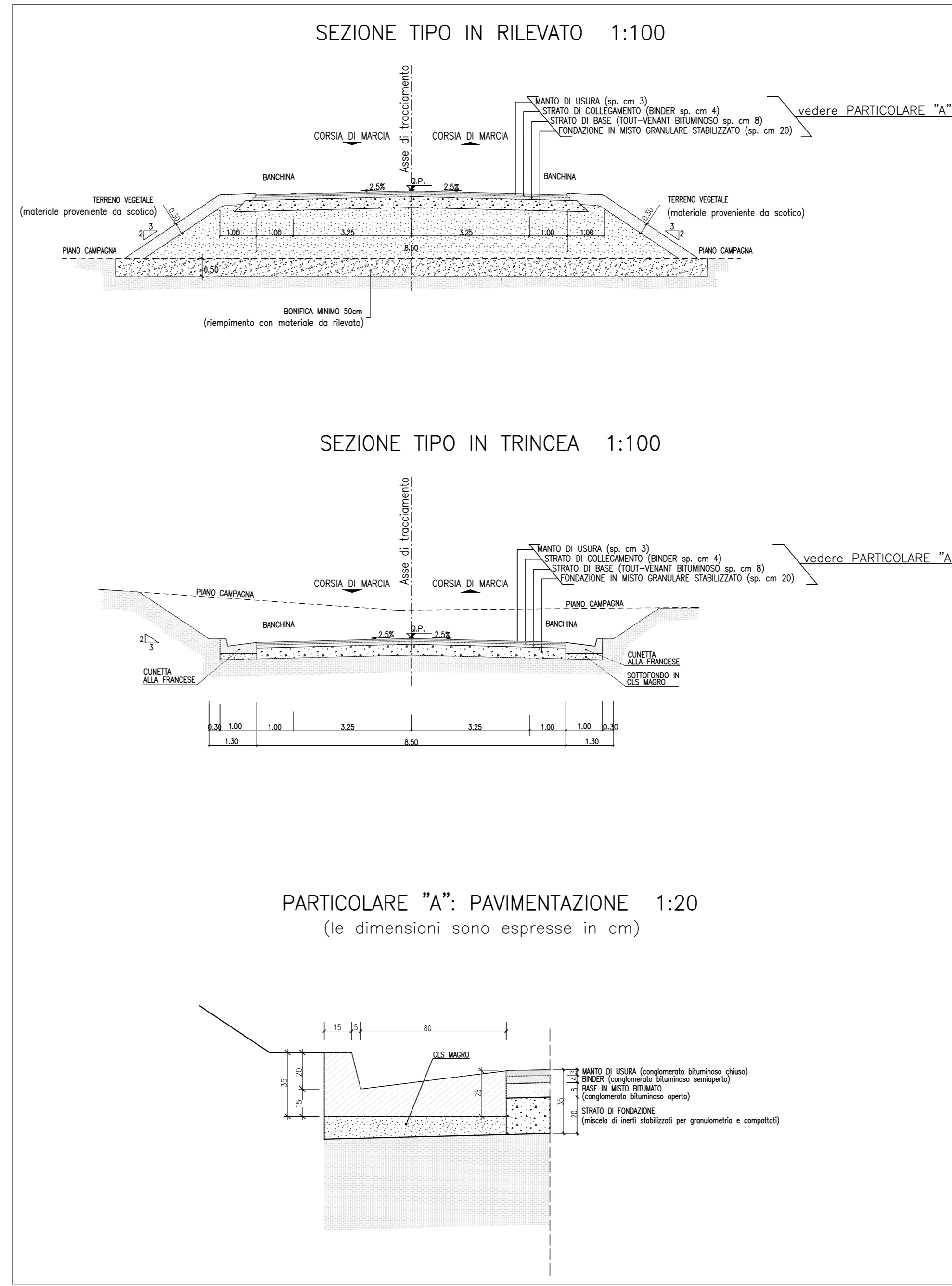
SEZIONE TIPO (Categ. F2) SCALA 1:100
