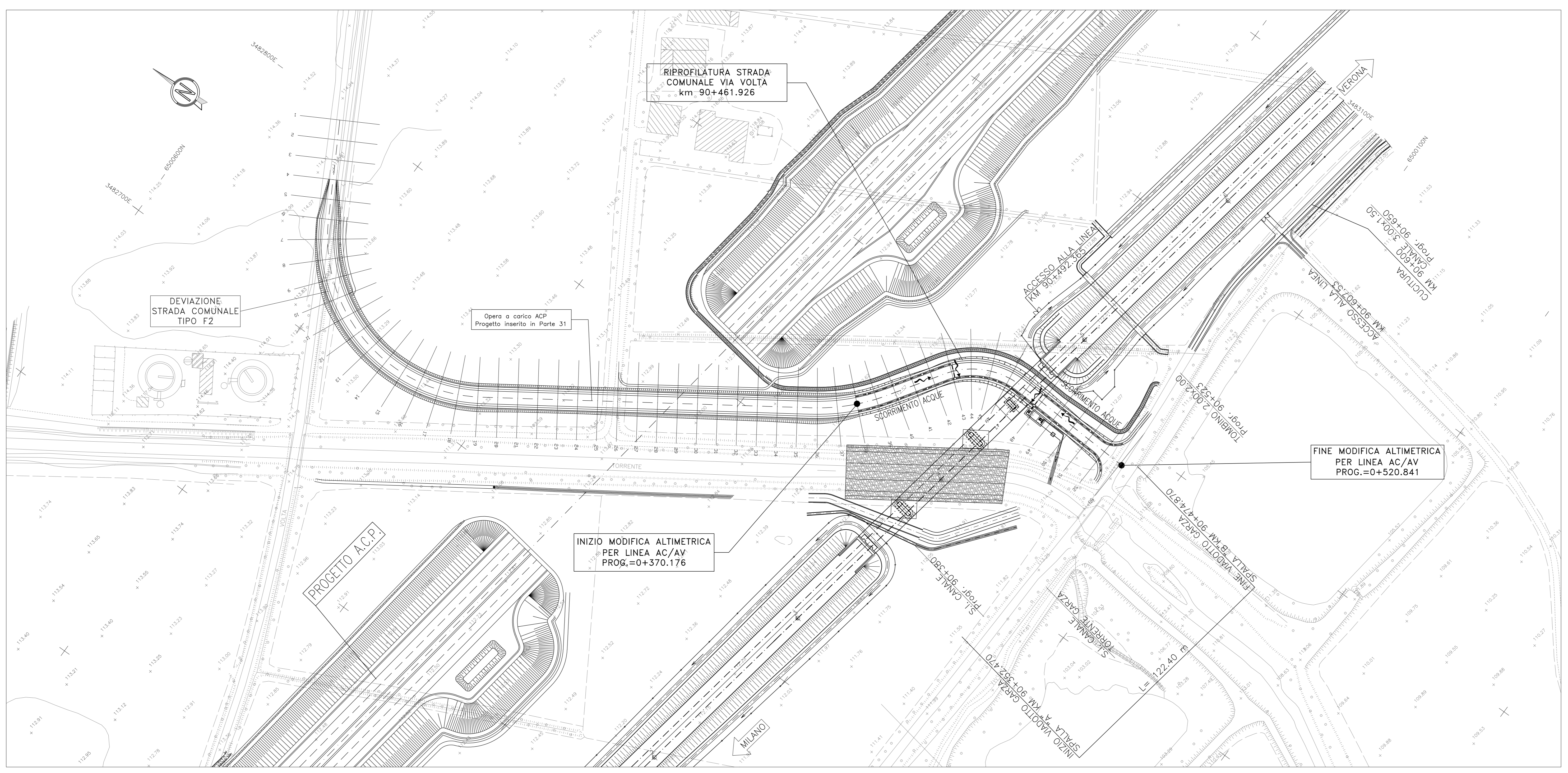
PLANIMETRIA VIA VOLTA SCALA 1:1000
