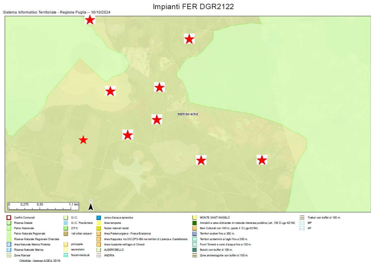
Figura 3 - Ubicazione dell'impianto rispetto alle aree non idonee ex RR 24/2010 (i 9 aerogeneratori sono indicati con una stella rossa)
