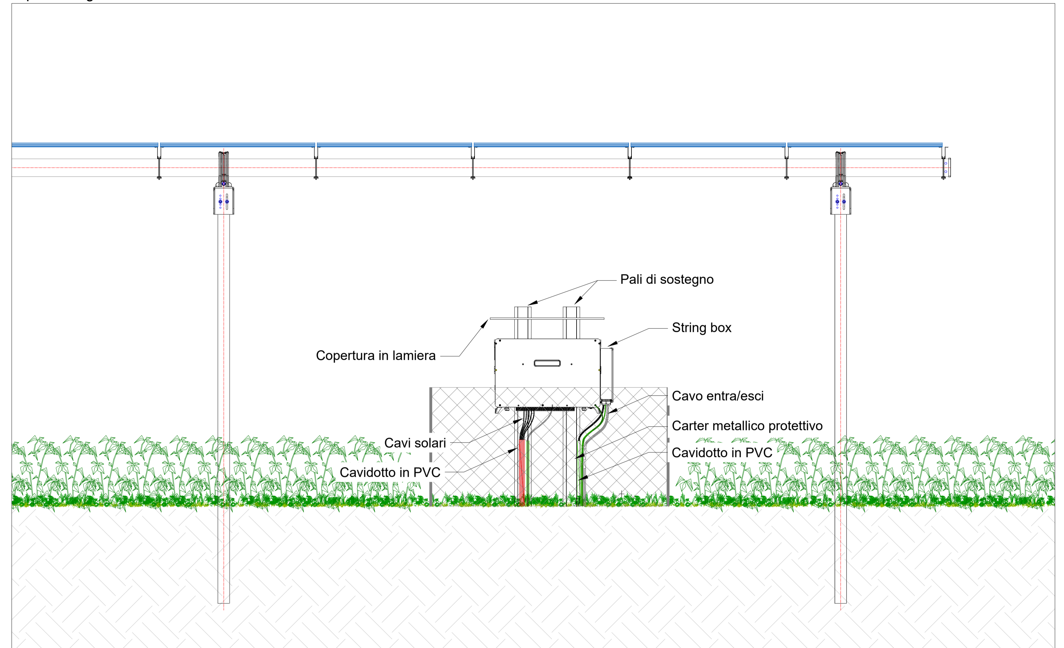
Tipico string box - Vista laterale - Scala 1:20
