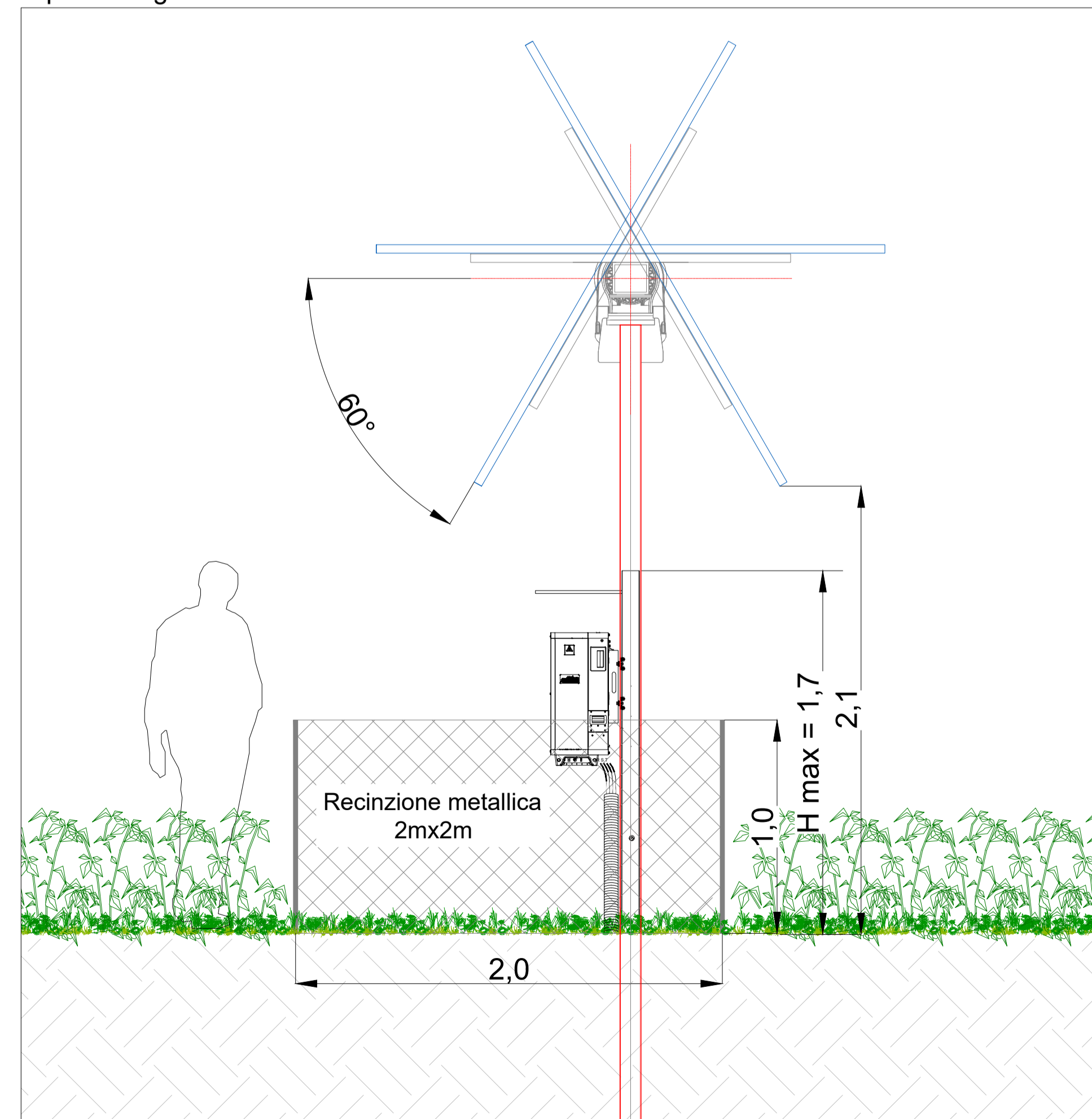
Tipico string box - Vista laterale - Scala 1:20
