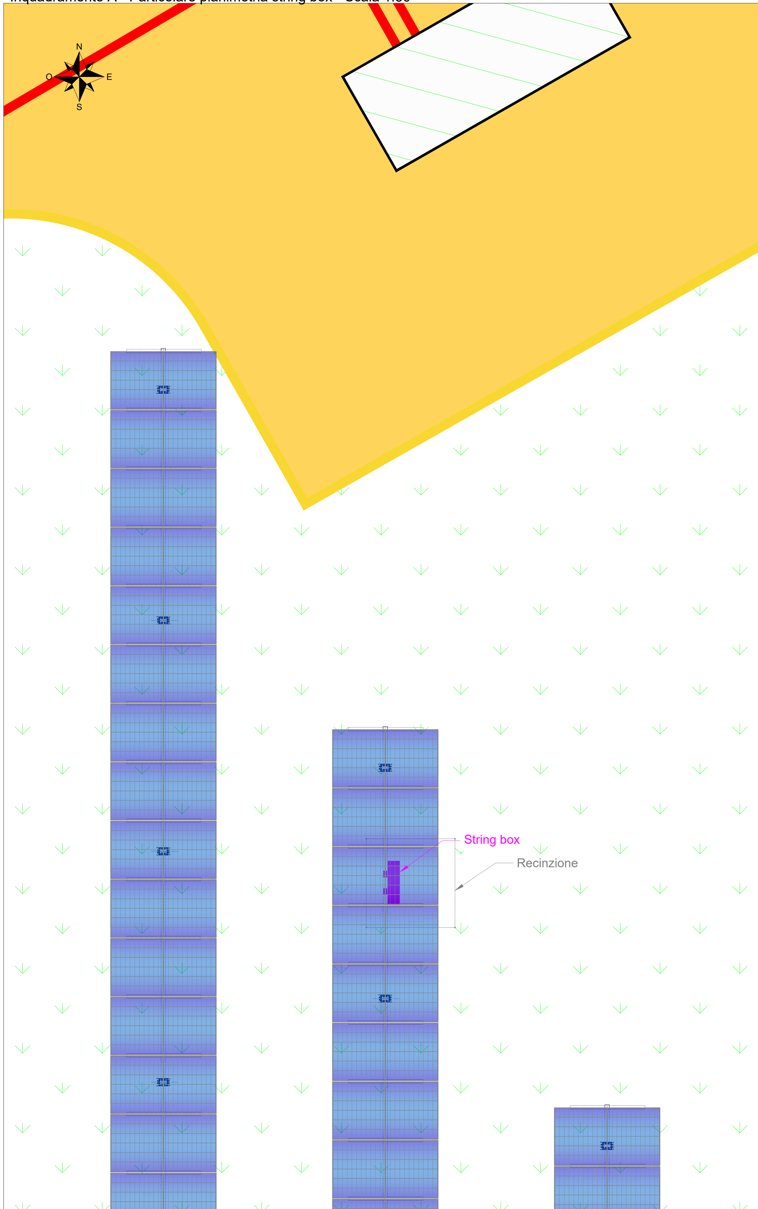
Inquadramento A - Particolare planimetria string box - Scala 1:50
