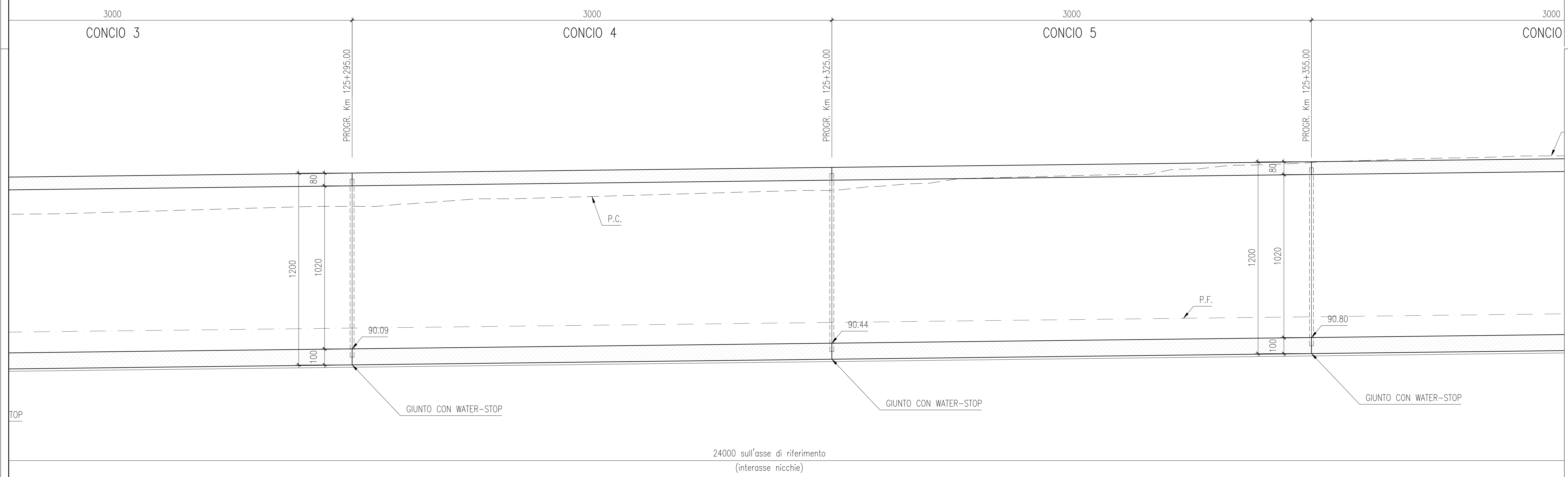
PROFILO LONGITUDINALE SCALA 1:100
