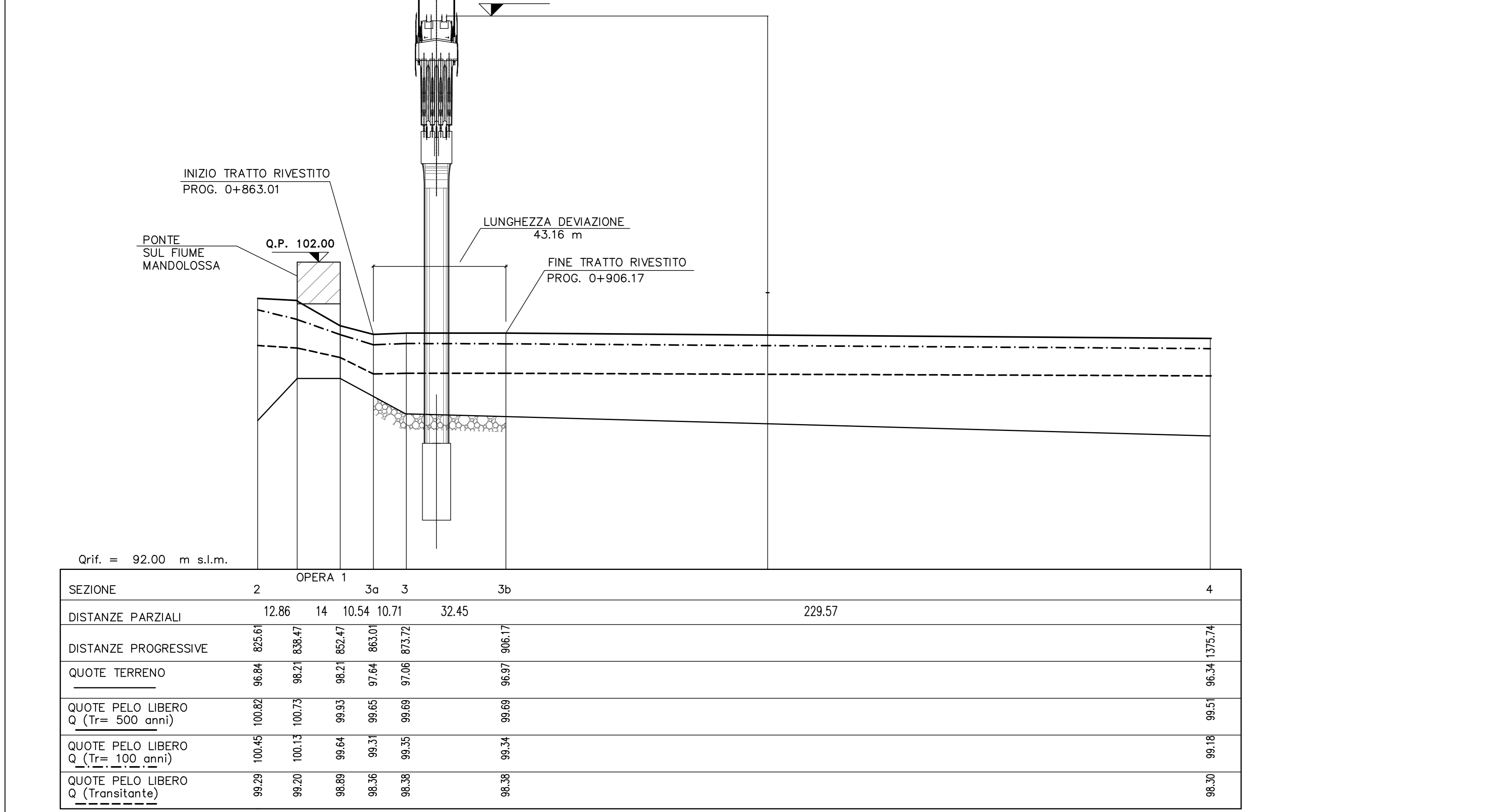
TRATTO 2 PROG. 825.61 - 1375.74
