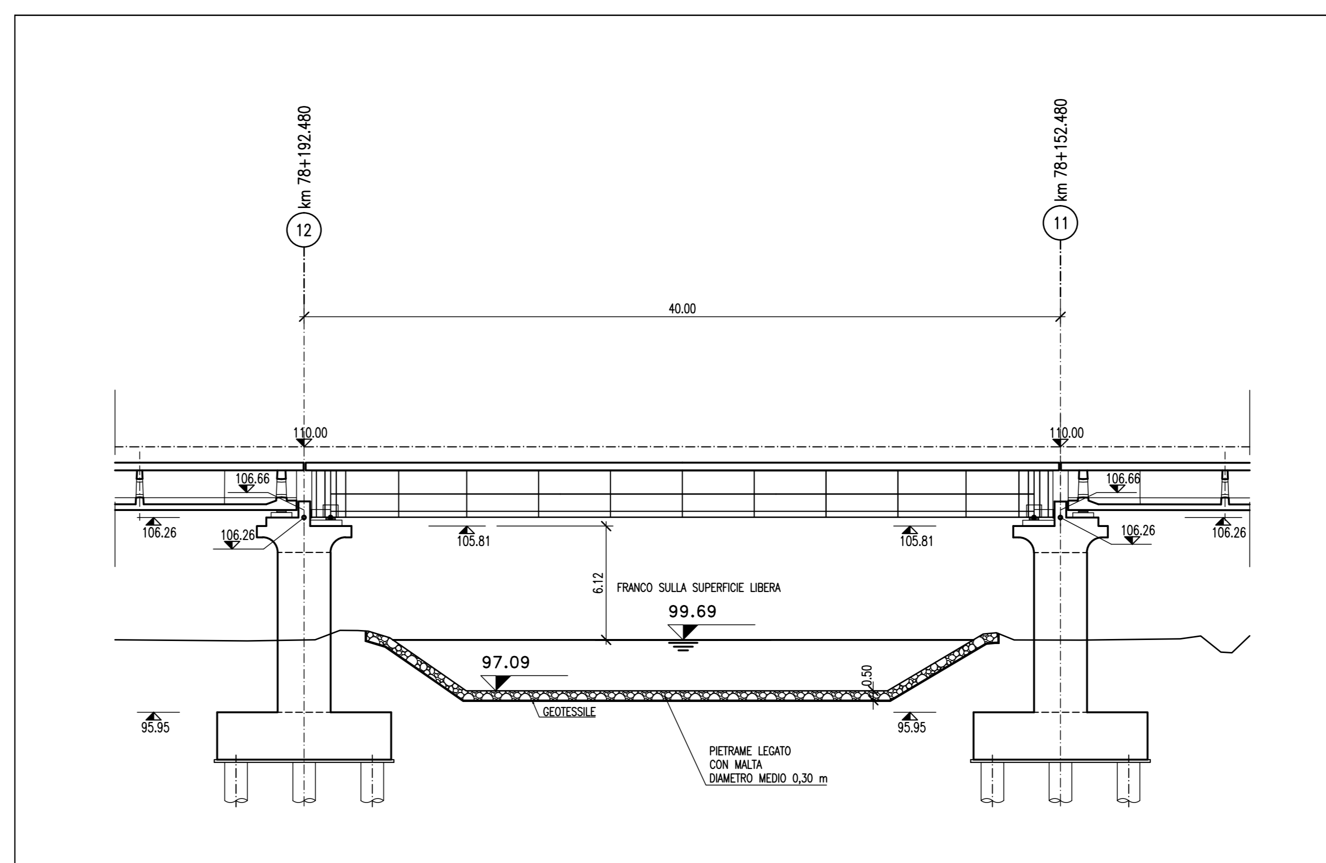
SEZIONE IN ASSE ALL'ATTRAVERSAMENTO scala 1:200
