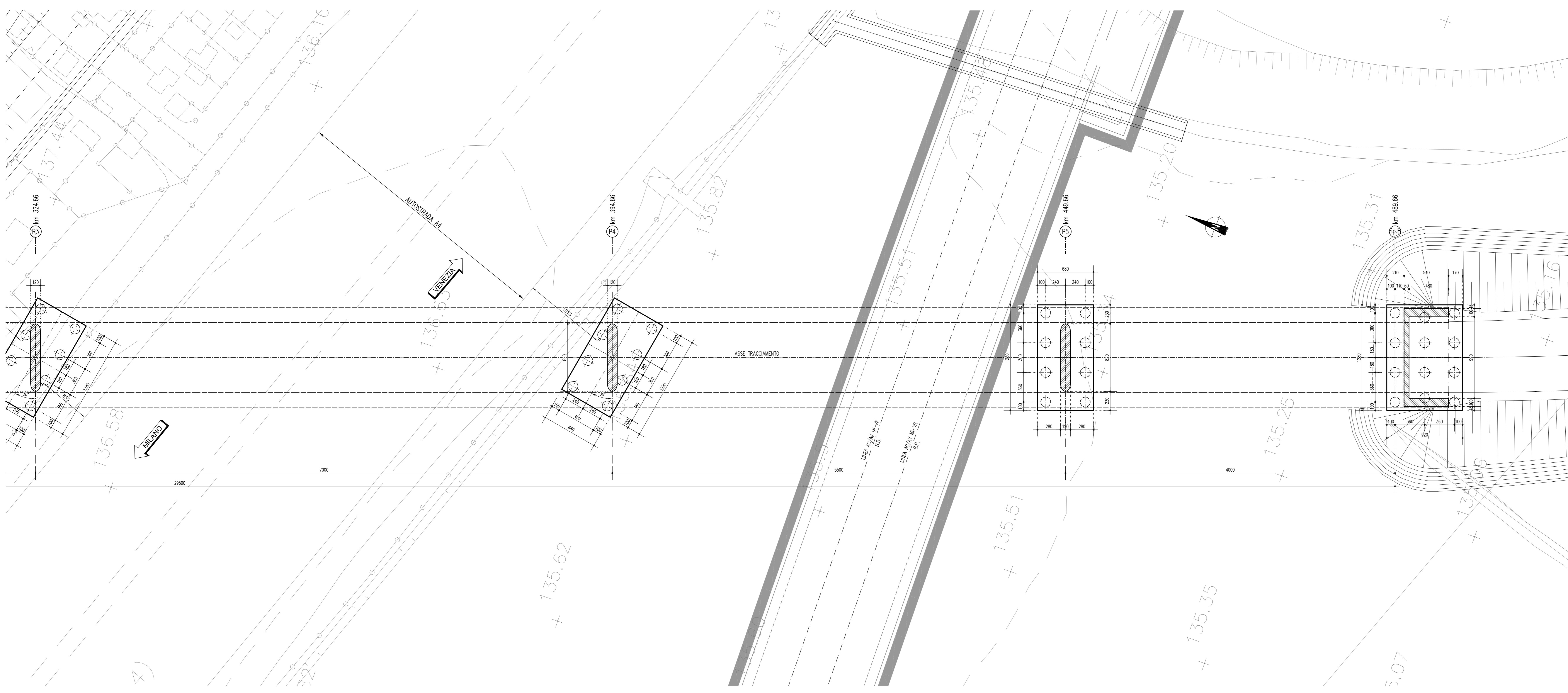
PIANTA FONDAZIONI 1:200
