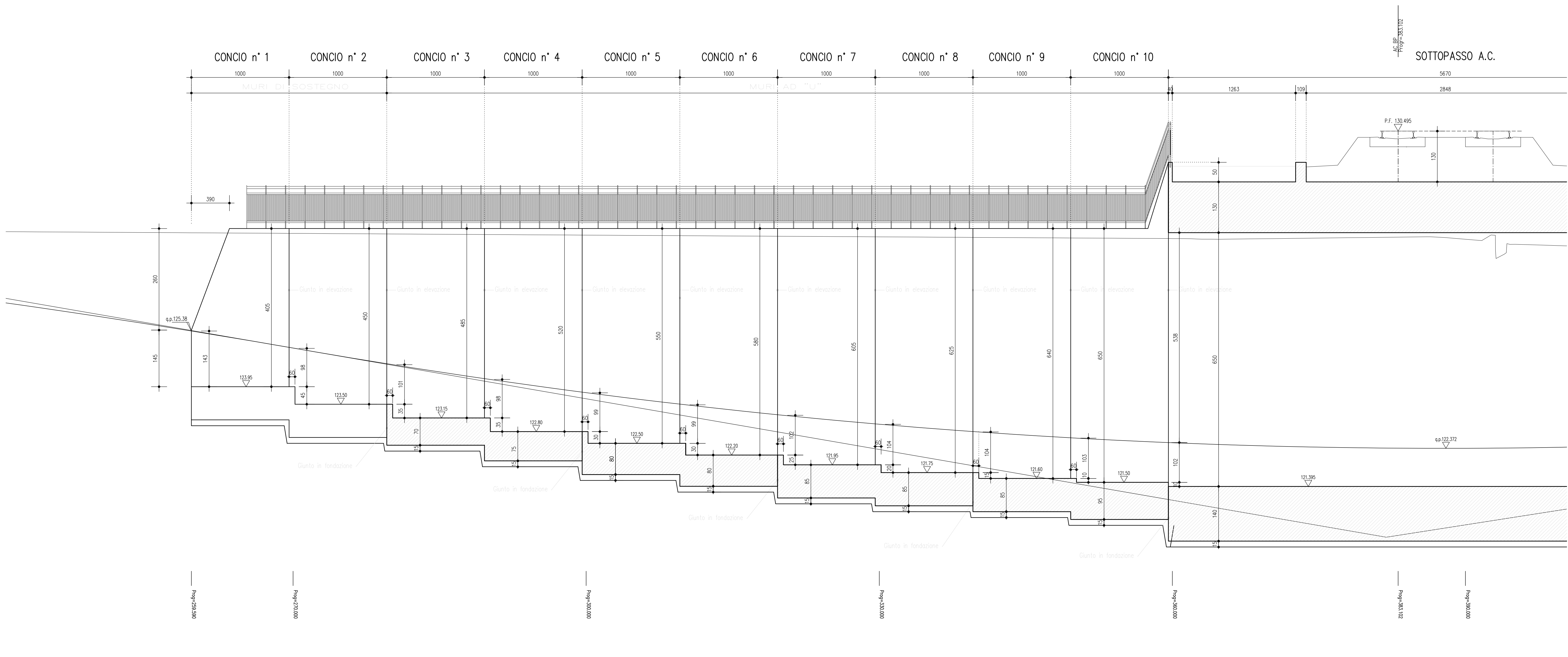
SEZIONE LONGITUDINALE IN CORRISPONDENZA ASSE TRACCIAMENTO 1:200/50
