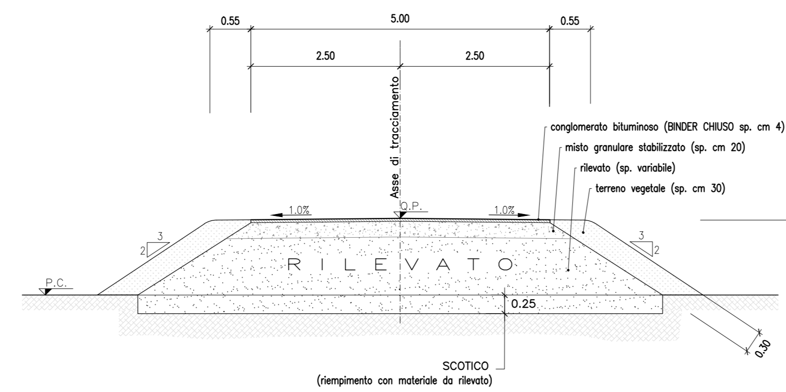
SEZIONE TIPO IN RILEVATO (PAVIMENTAZIONE IN CONGLOMERATO BITUMINOSO) Scala 1:50
