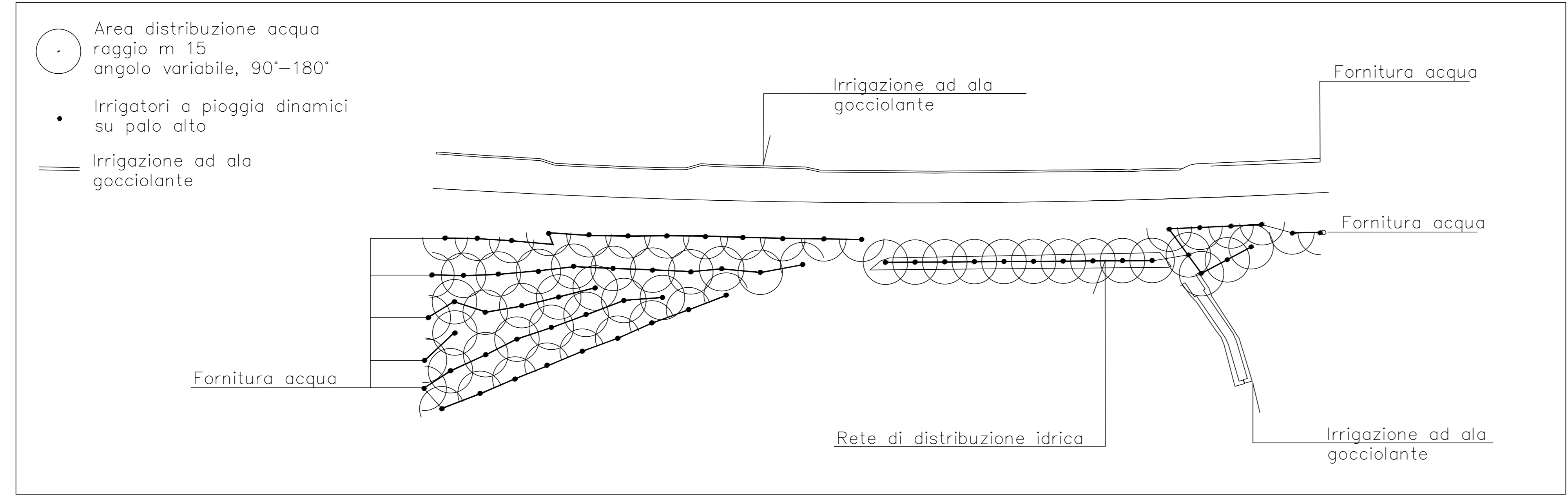
2 Schema d'impianto d'irrigazione: planimetria Scale 1:2000
