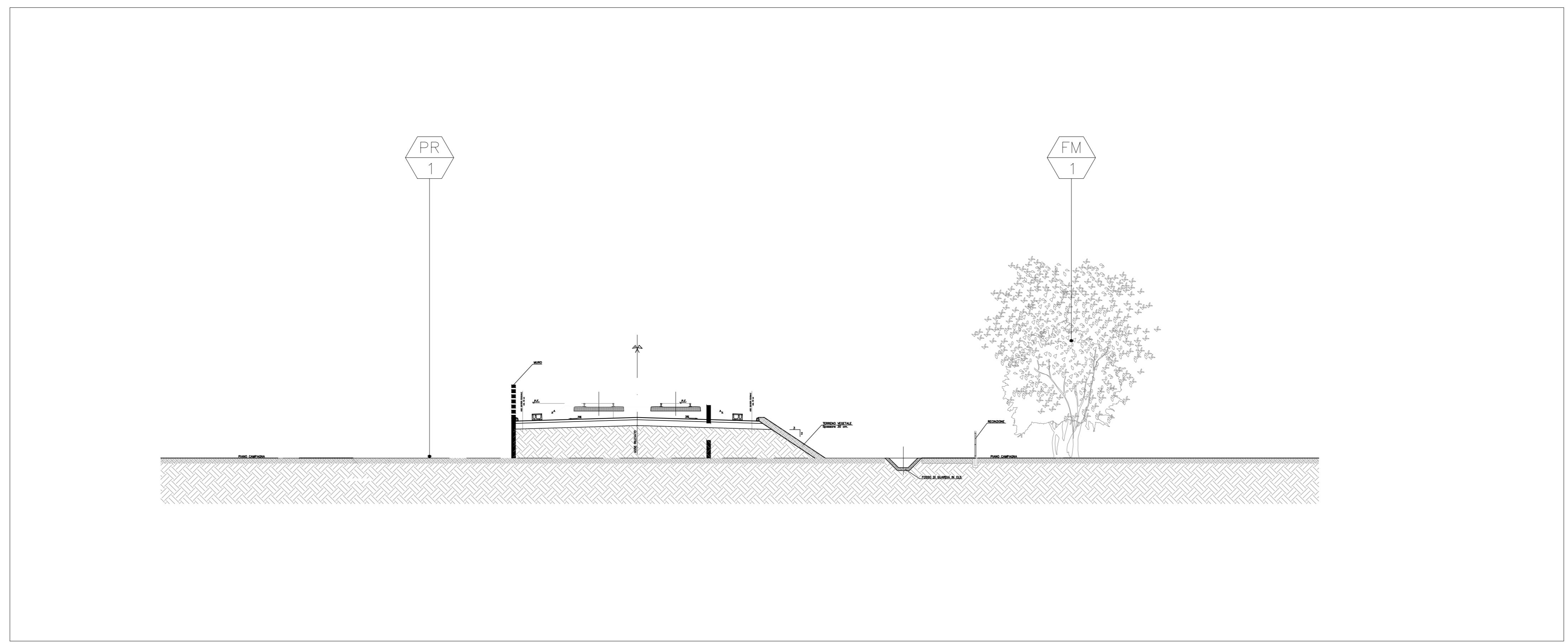
AA Sezione AA Scala 1:200
