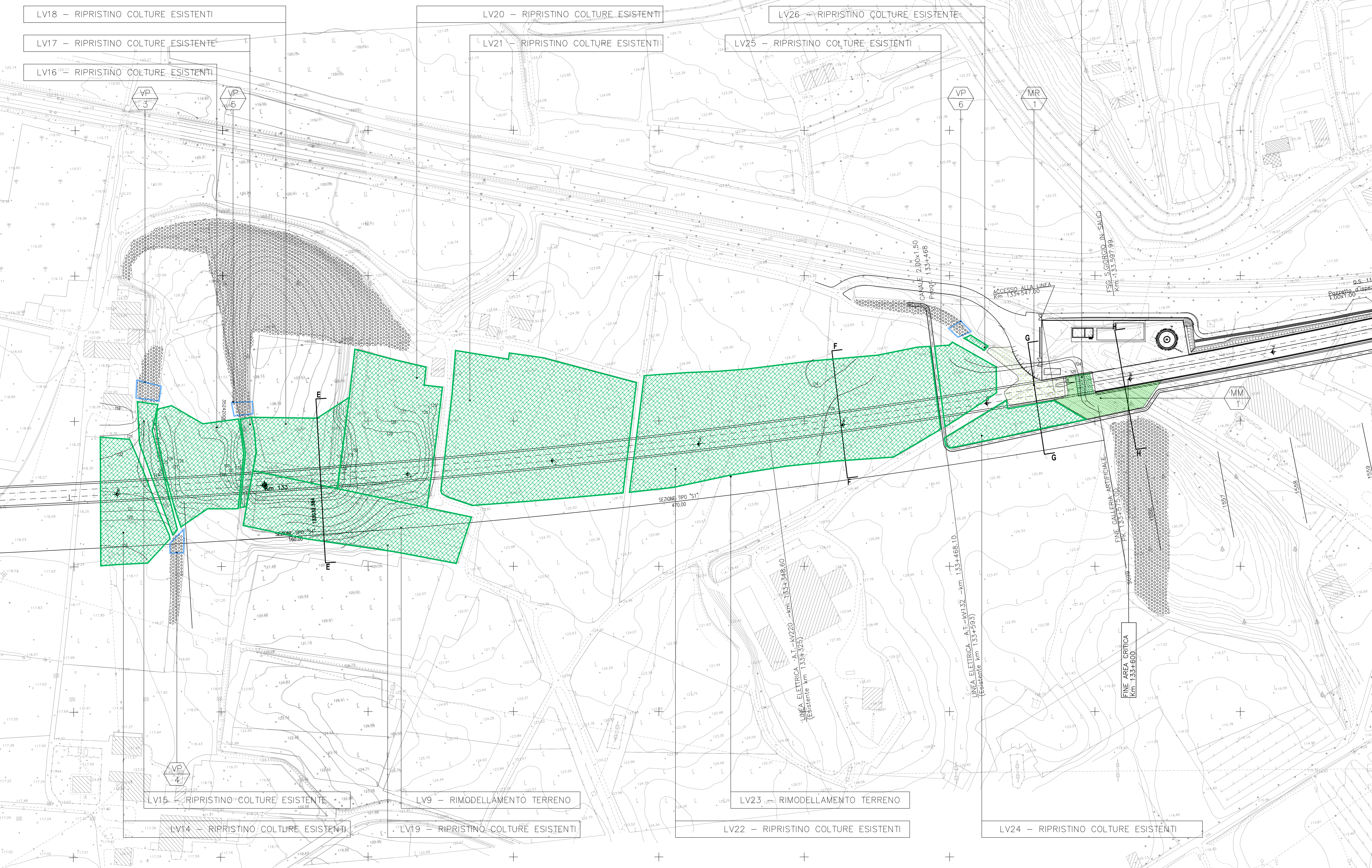
1 Planimetria di progetto Scala 1:1000
