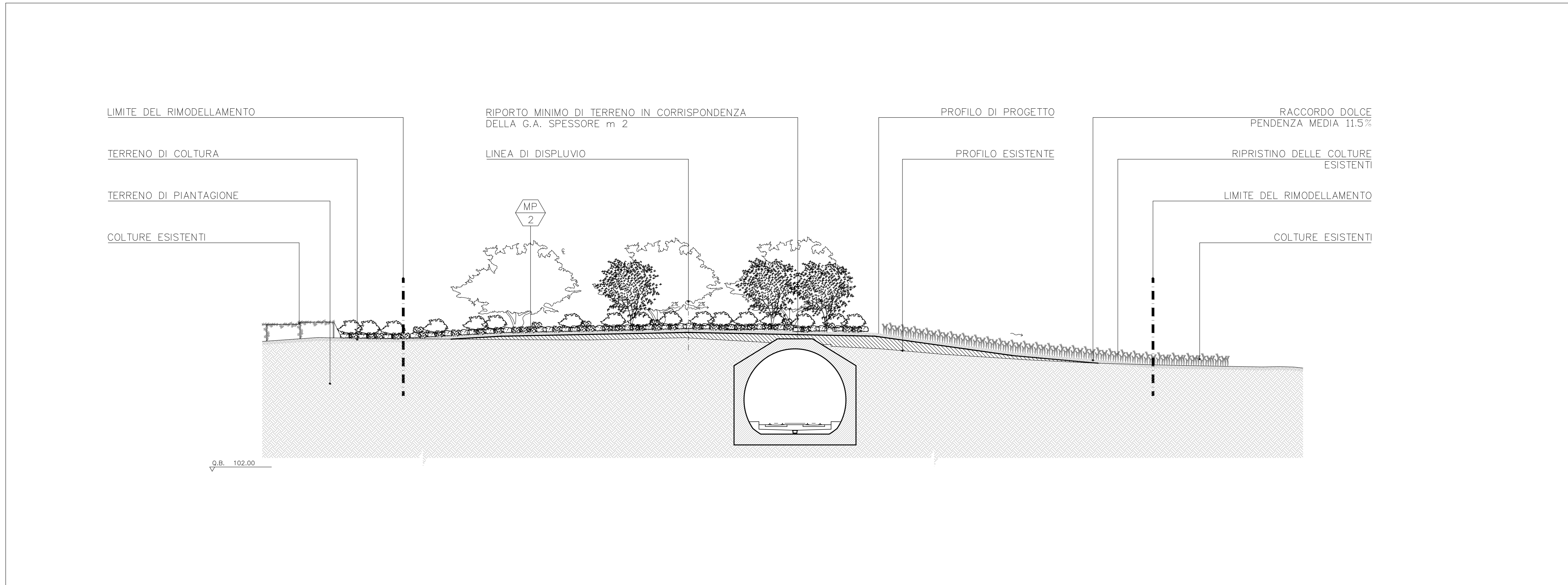
BB Sezione BB Scala 1:200
