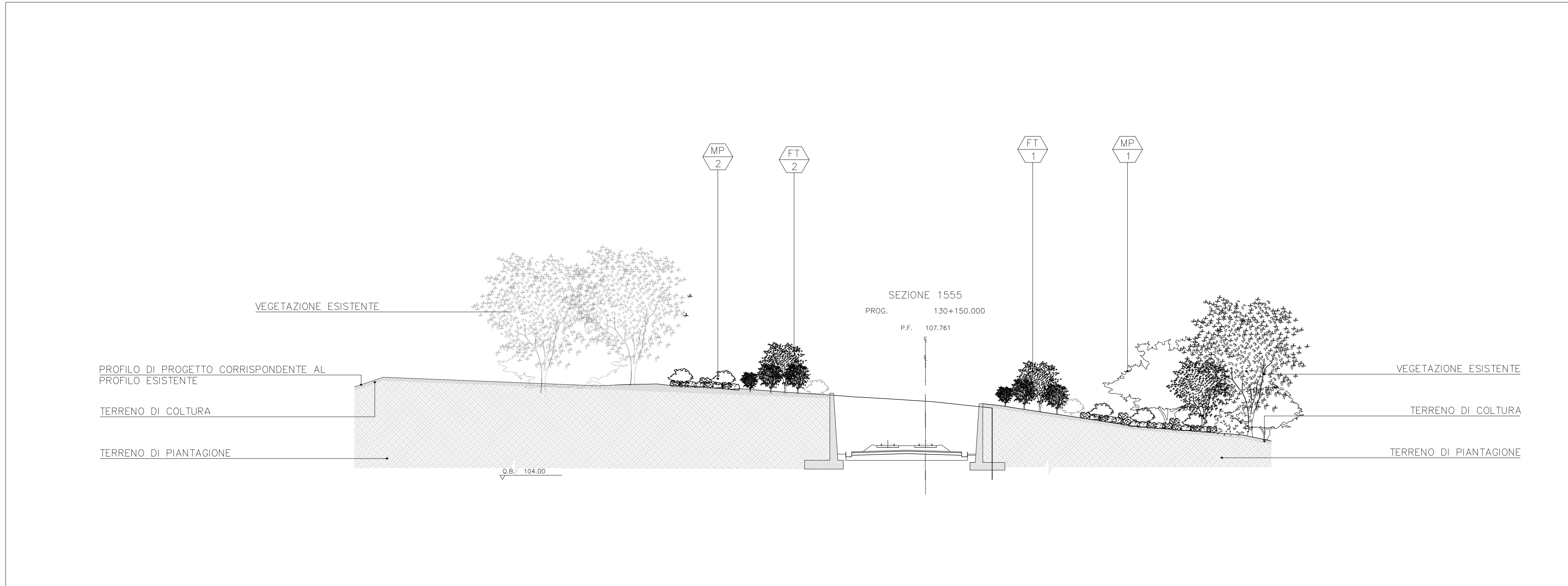
AA Sezione AA Scala 1:200
