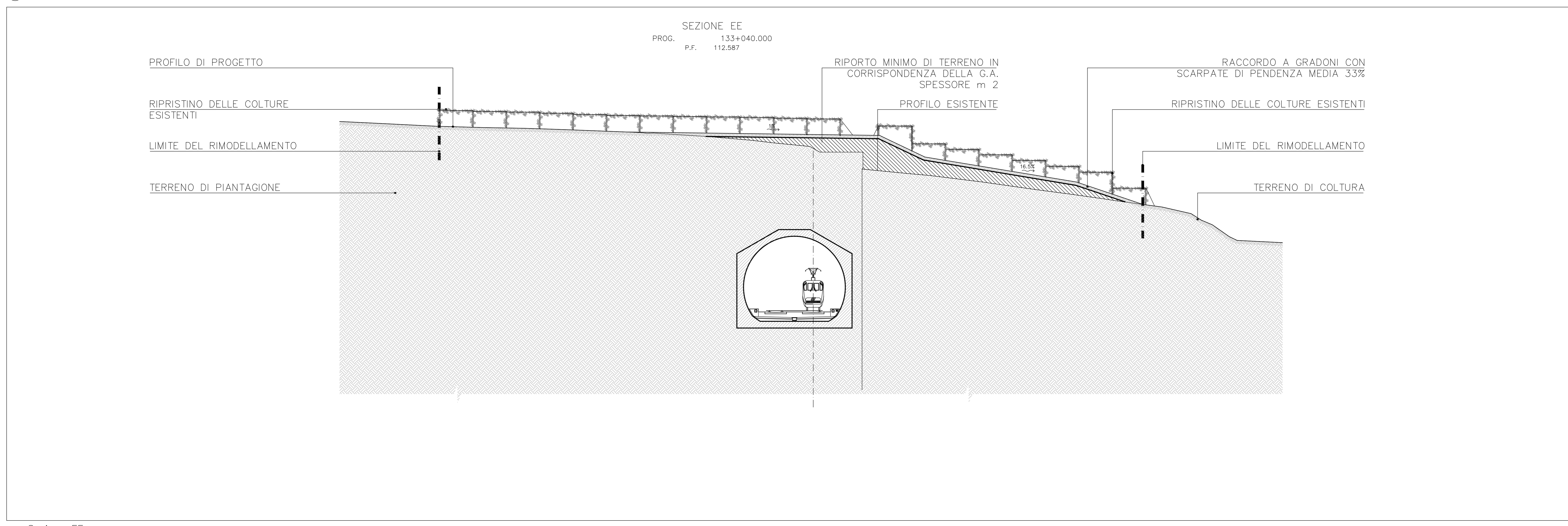
Sezione EE Scala 1:200
