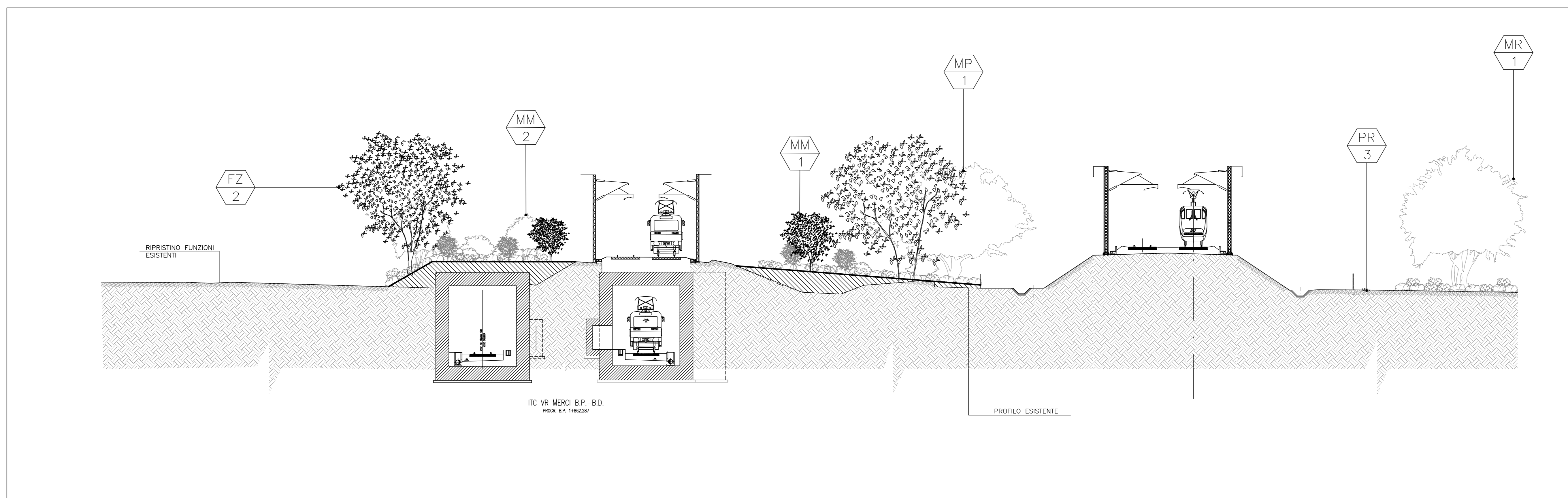
3 Sezione CC Scala 1:200
