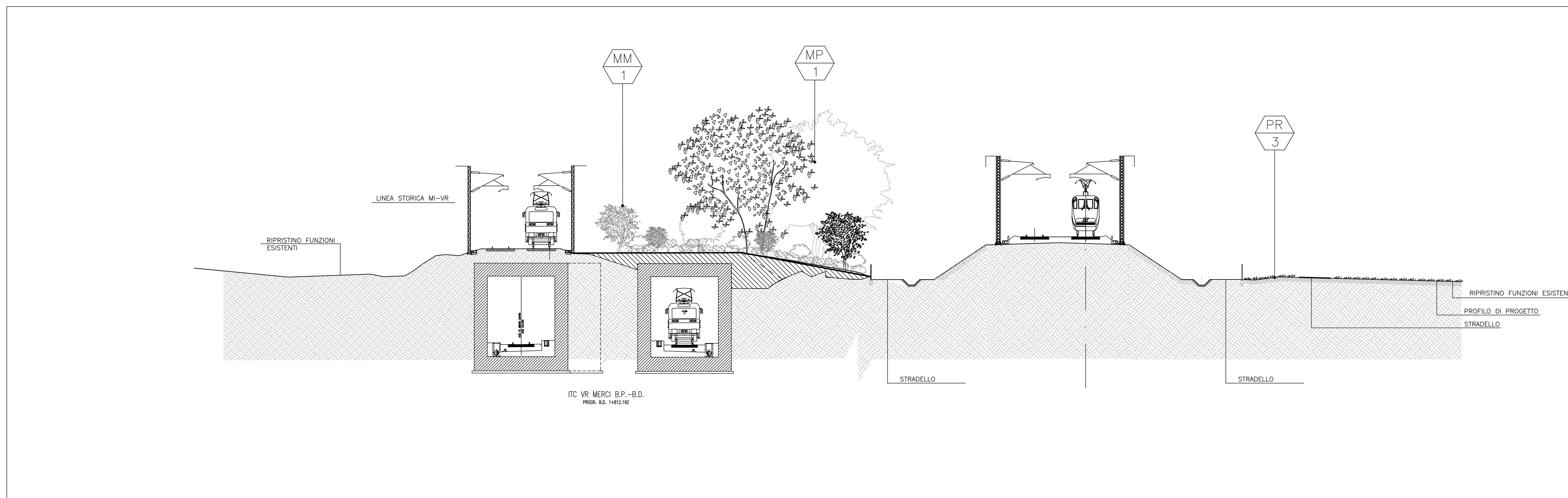
2 Sezione BB Scala 1:200
