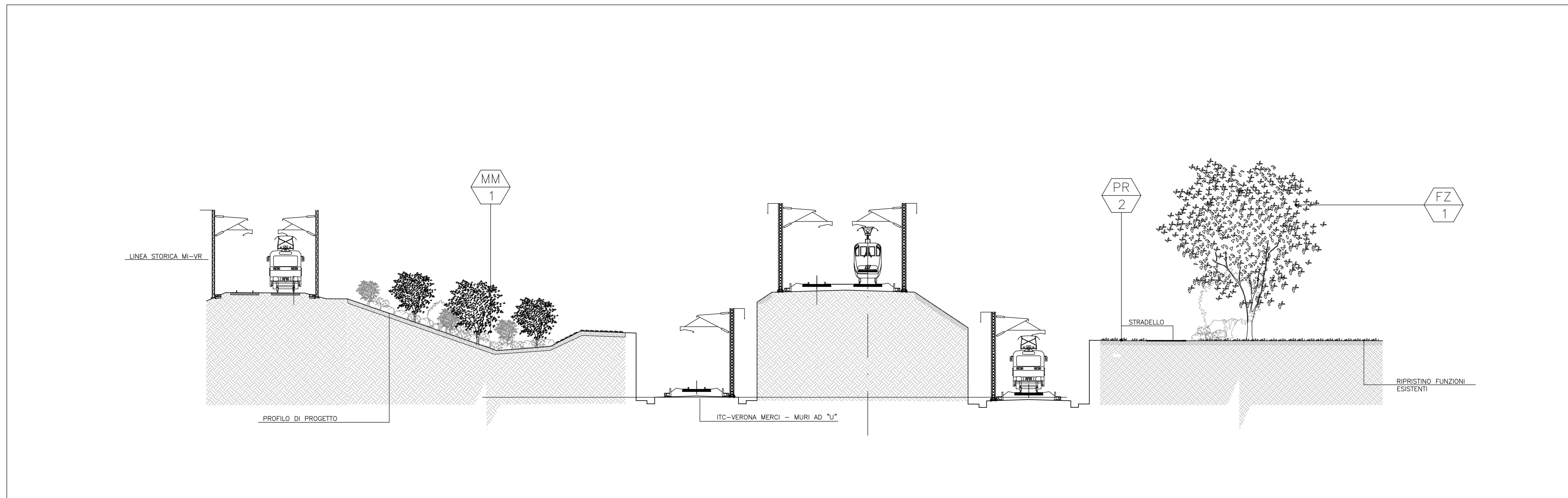
1 Sezione AA Scala 1:200
