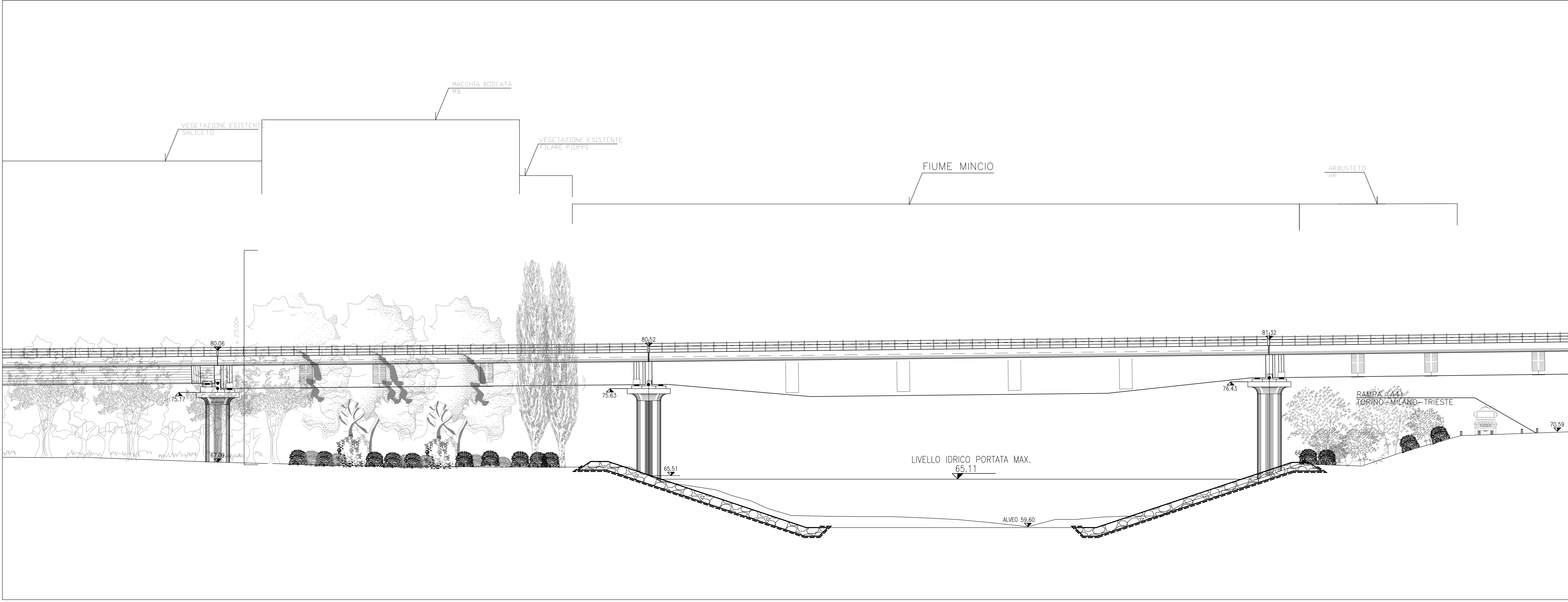
Sezione BB' 1:200
