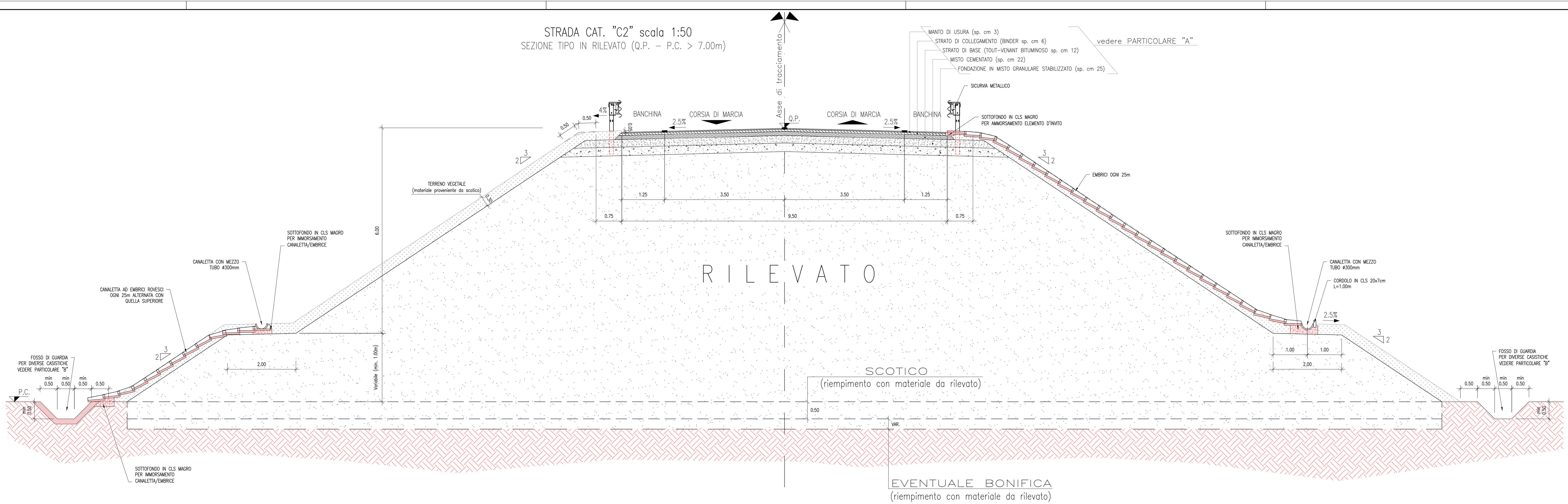
STRADA CAT. "C2" scala 1:50 SEZIONE TIPO IN RILEVATO (1.50m < Q.P. - P.C. ≤ 7.00m)
