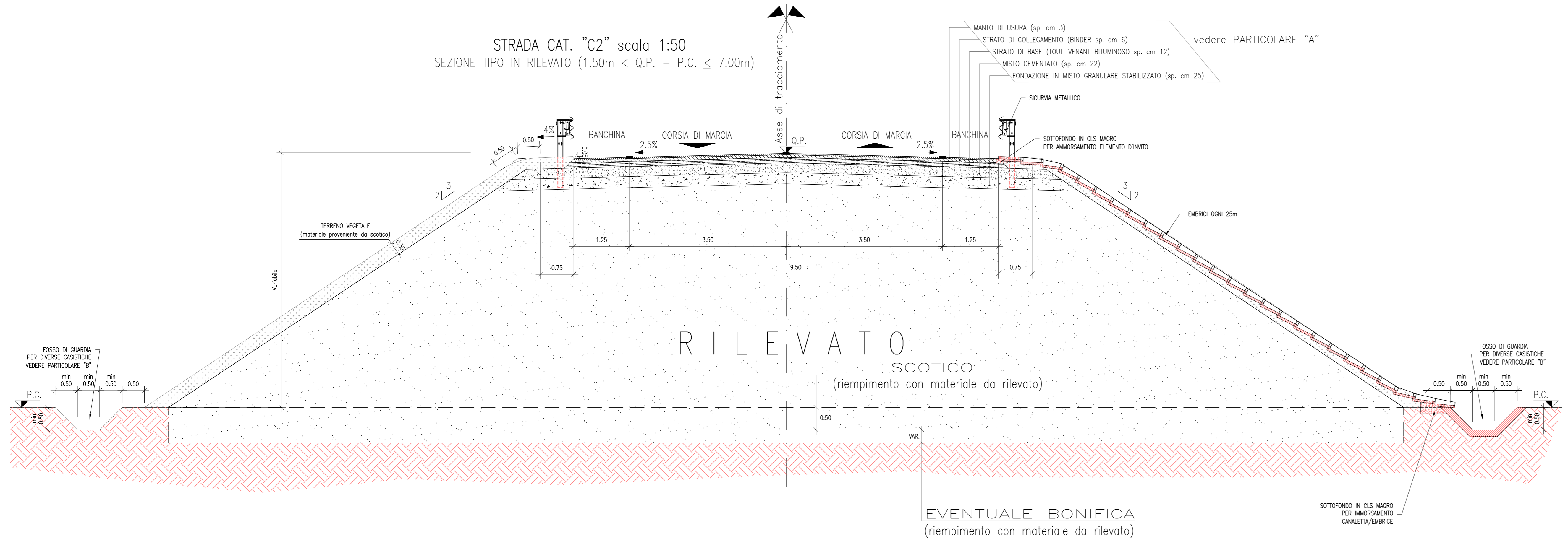
STRADA CAT. "C2" scala 1:50 SEZIONE TIPO IN RILEVATO (0.50m ≤ Q.P. - P.C. ≤ 1.50m)
