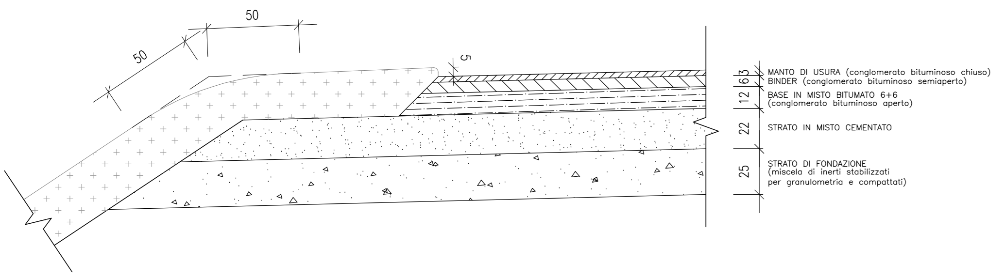
PARTICOLARE "A": PAVIMENTAZIONE scala 1:20 (Le dimensioni sono espresse in cm)
