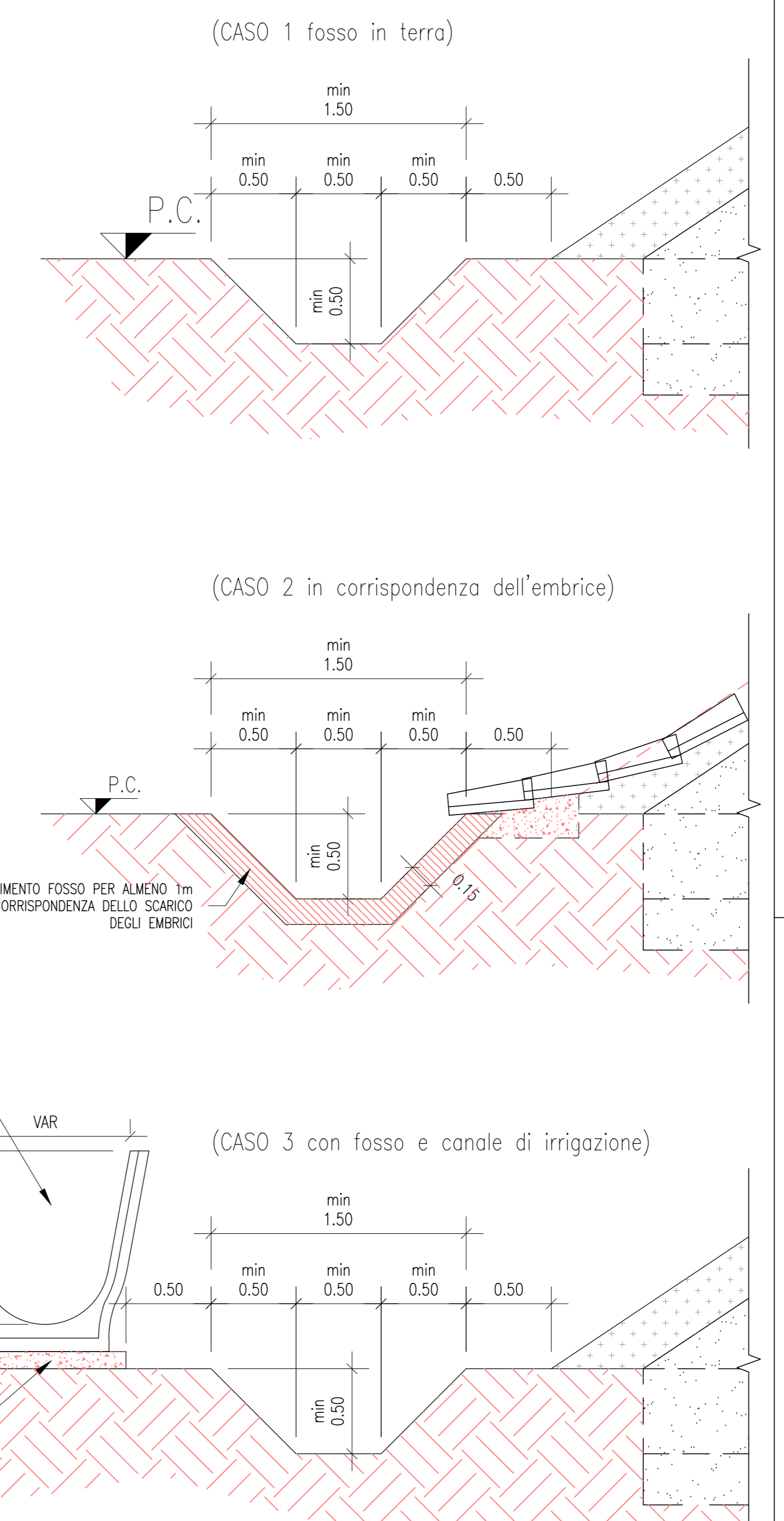
PARTICOLARE "B": FOSSO DI GUARDIA scala 1:25
