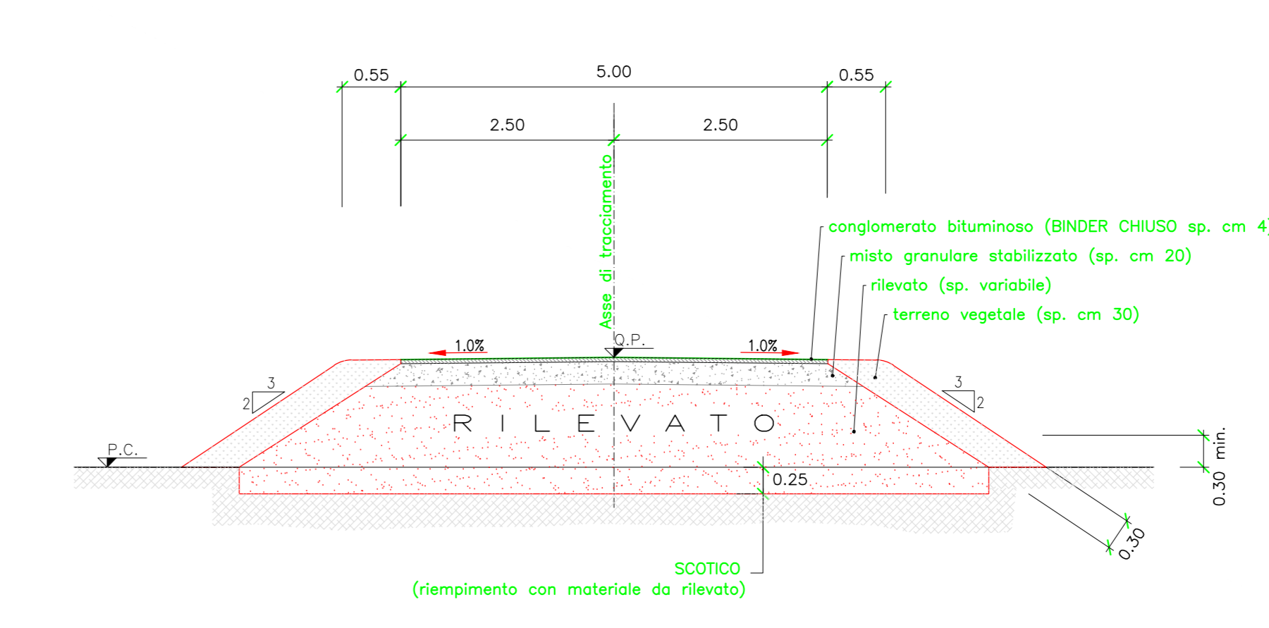
VIABILITA' DI CUCITURA SEZIONE TIPO IN RILEVATO (PAVIMENTAZIONE IN CONGLOMERATO BITUMINOSO) Scala 1:50
