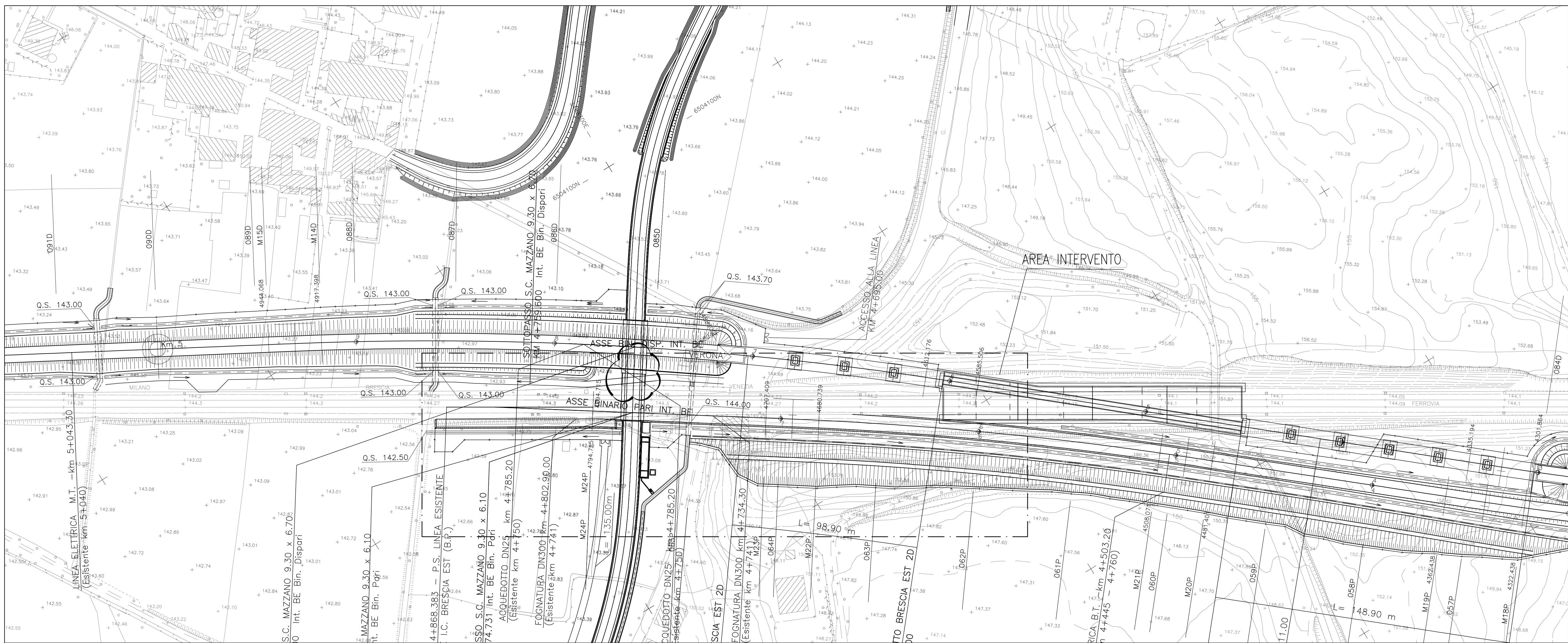
STRALCIO PLANIMETRICO 1 SCALA 1:1000
