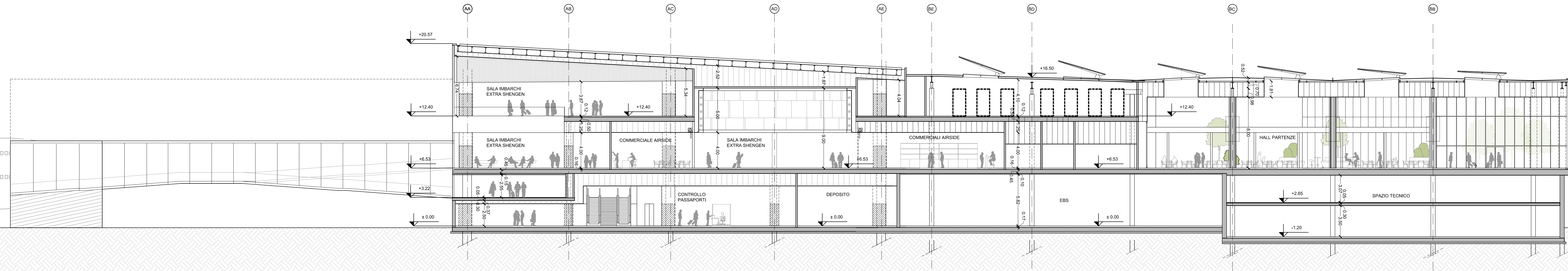
01 Sezione Trasversale Extra Schengen DD 1:200
