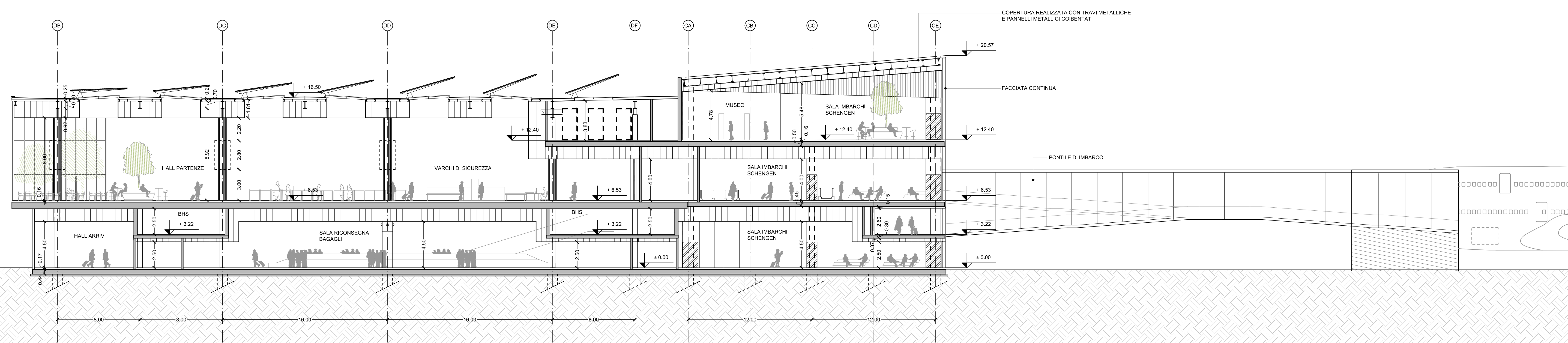
02 Sezione Trasversale Schengen CC 1:200
