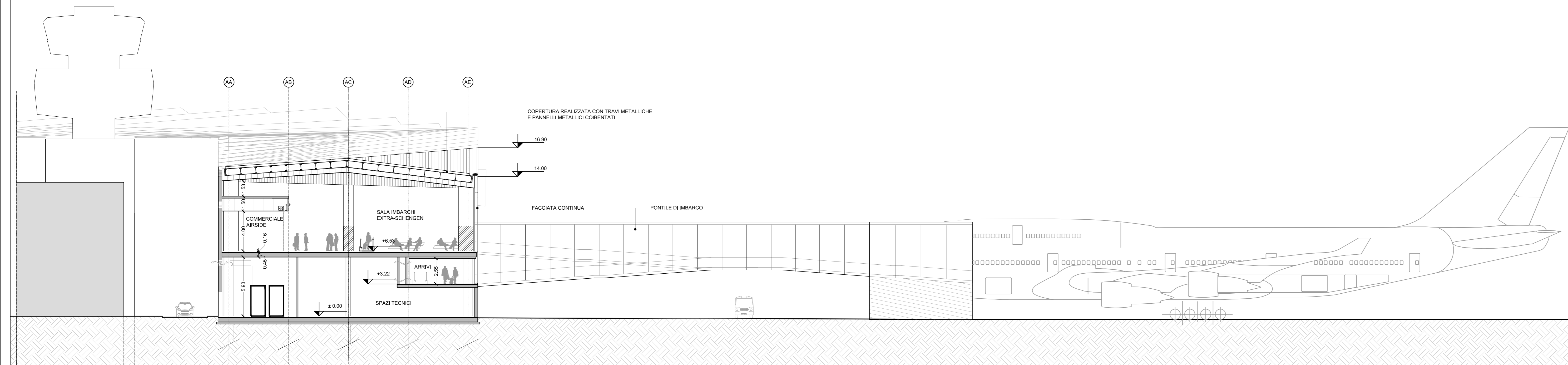
02 Sezione Trasversale Airside FF 1:200
