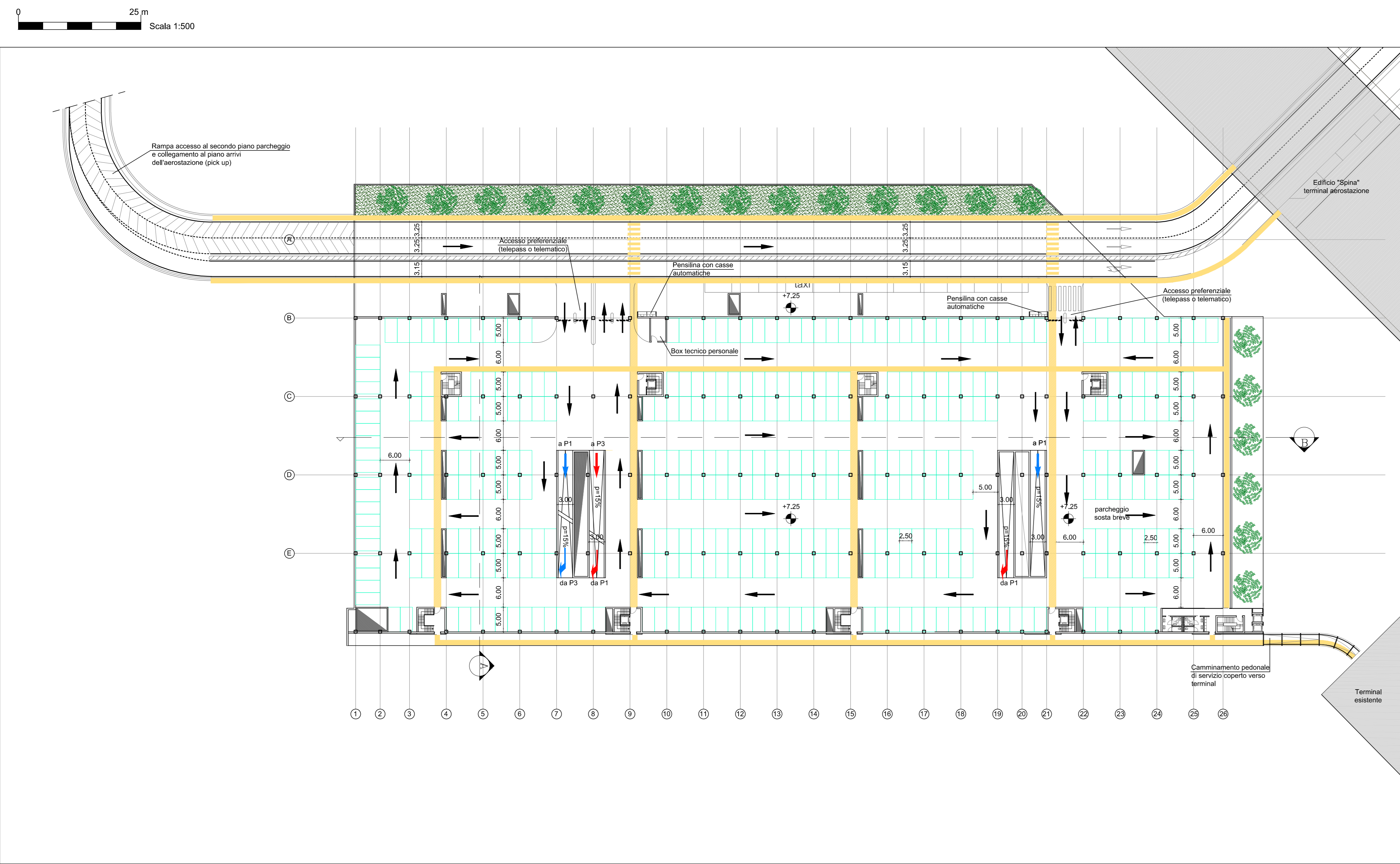
Pianta secondo piano (quota +7.25)
