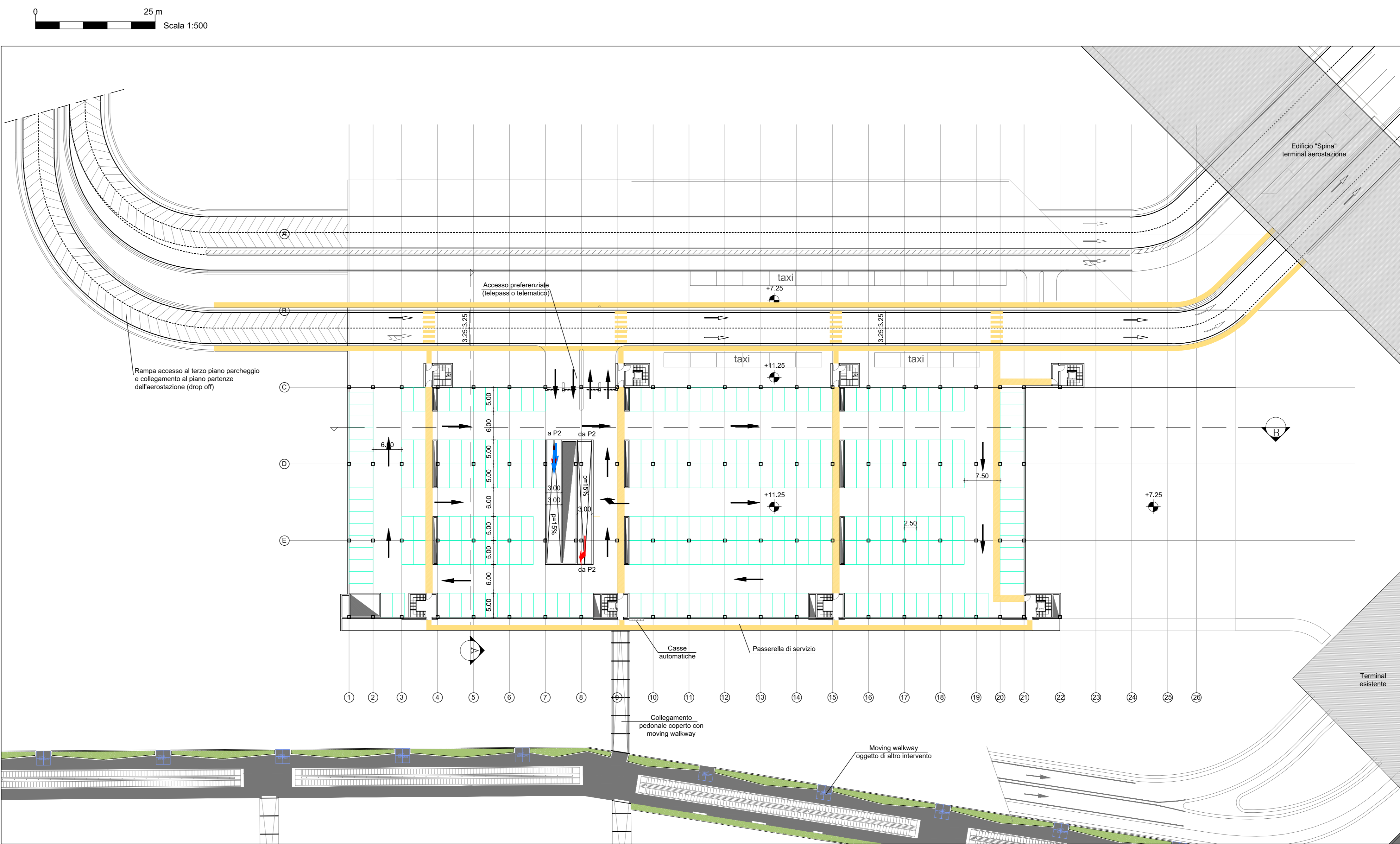
Pianta terzo piano (quota +11.25)
