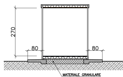
SEZIONE A-A
