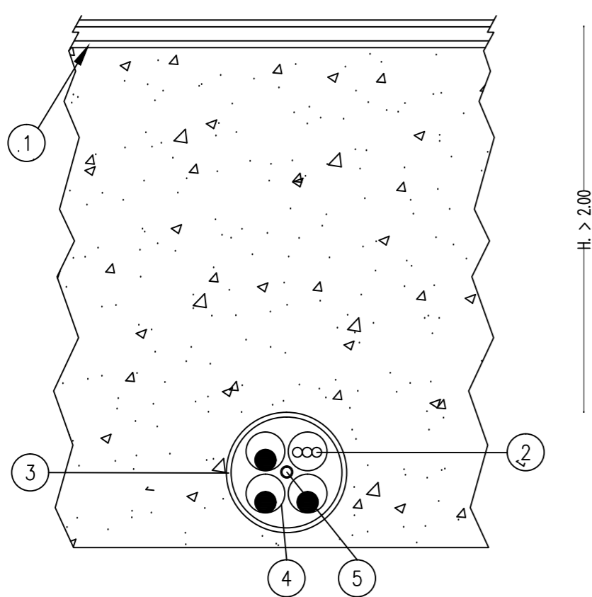
SEZIONE TIPO ATTRAVERSAMENTO CON SPINGITUBO
