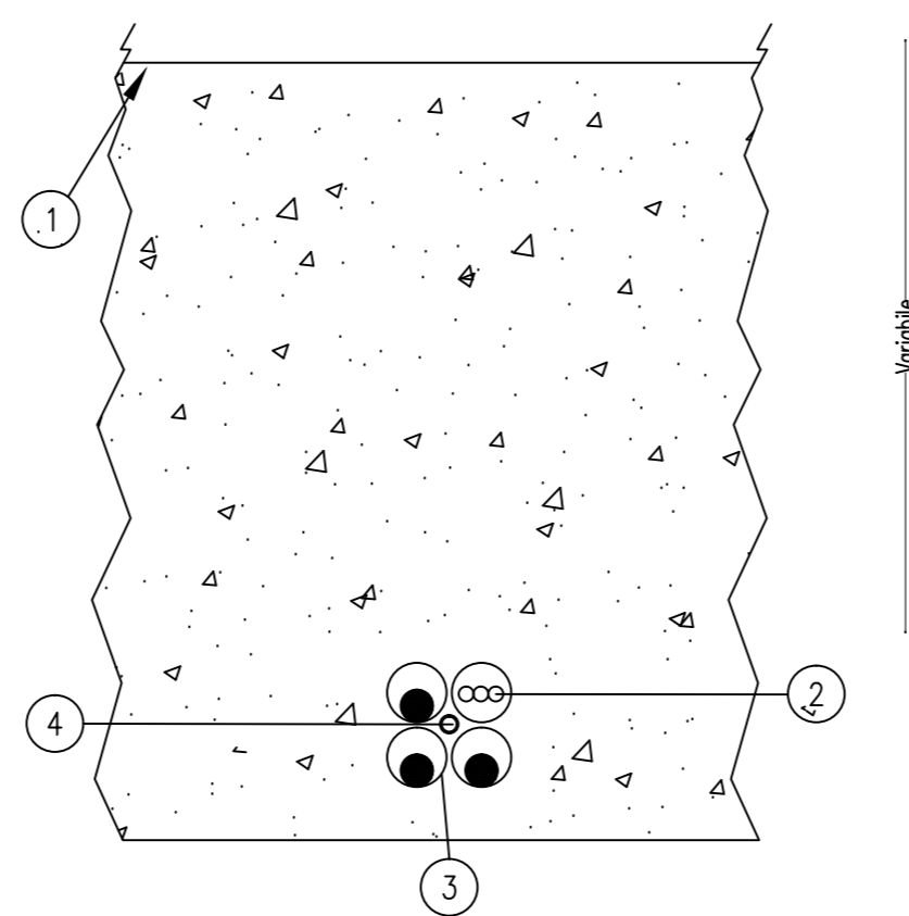
SEZIONE TIPO ATTRAVERSAMENTO T.O.C.
