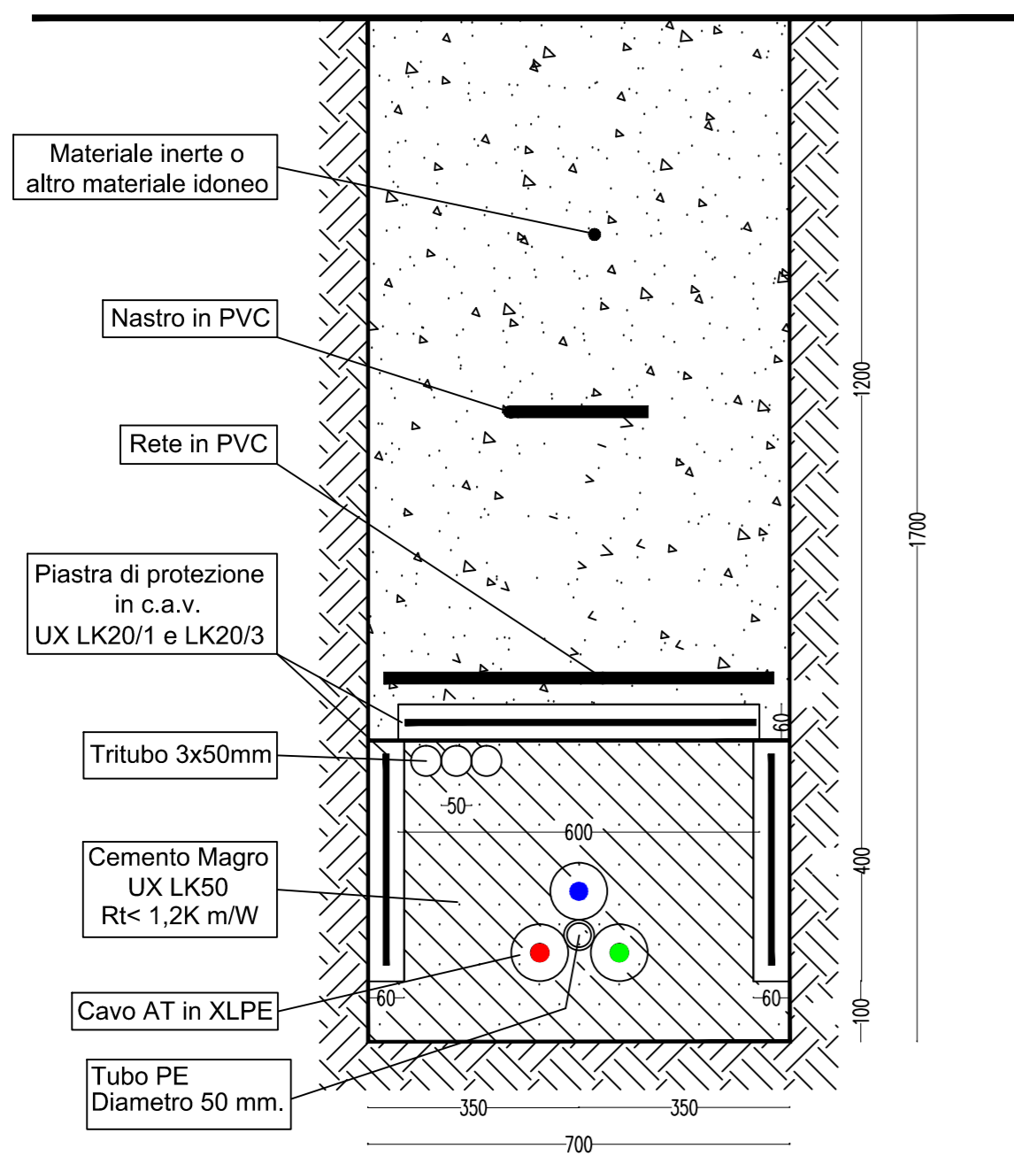
SEZIONE TIPO ATTRAVERSAMENTO CON SPINGITUBO
