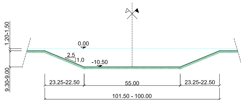
SEZIONE TRASVERSALE TIPO DEL CANALE
