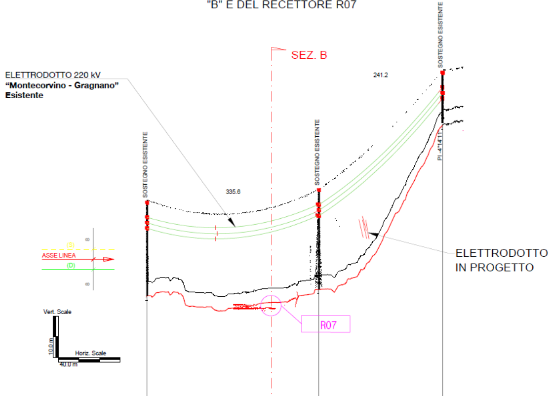
PROFILO E PLANIMETRIA CON INDIVIDUAZIONE DELLA SEZIONE "B" E DEL RECETTORE R07
