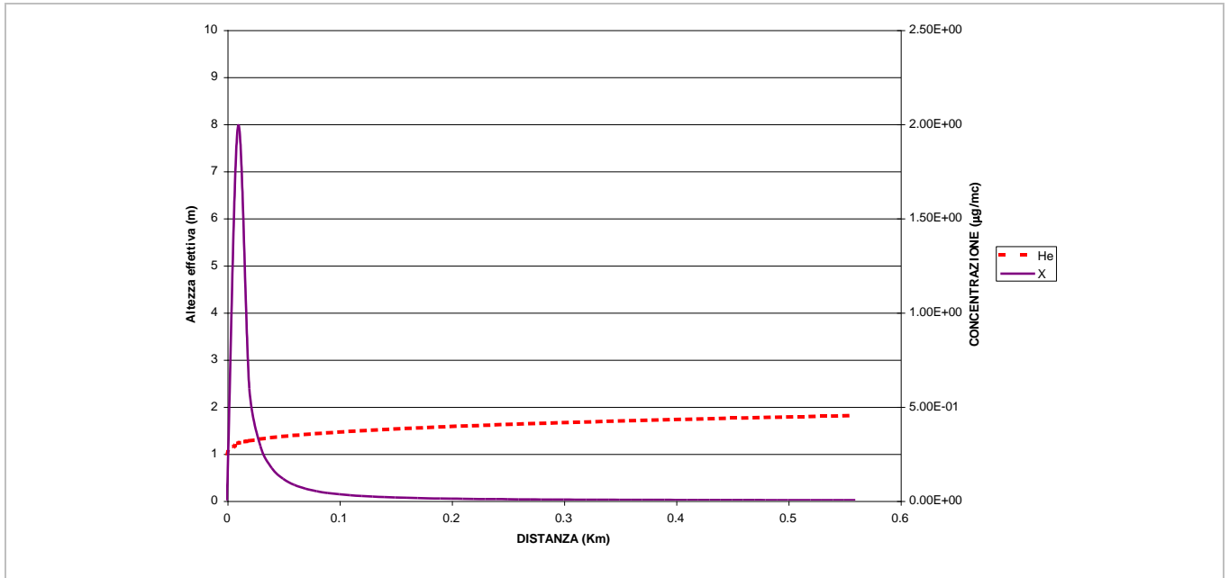
Figura 15 - ricadute al suolo per atmosfera instabile (He = elevation (distanza dal suolo delle particelle emesse) X = funzione di concentrazione del particolato)
