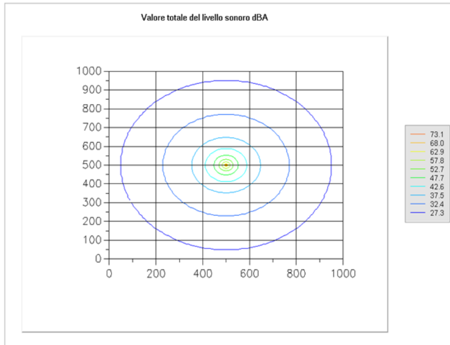
Figura 18 - diffusione della rumorosità ambientale relativamente alla fase di cantiere per la realizzazione di un sostegno tipo
