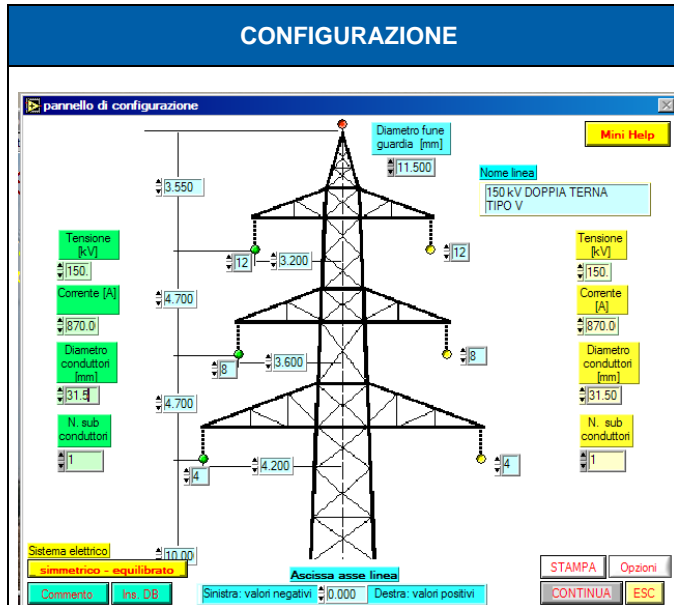
Configurazione 150 DT – Tipo V
