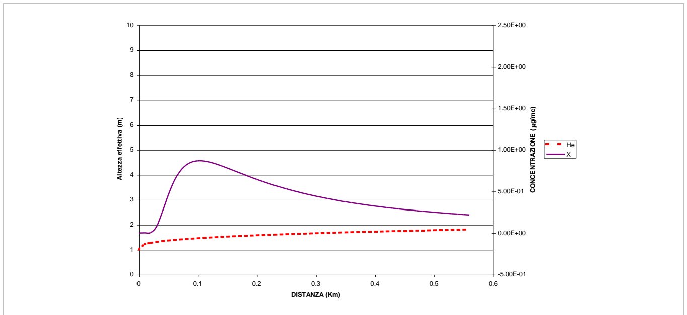
Figura 16 - ricadute al suolo per atmosfera stabile (He = elevation (distanza dal suolo delle particelle emesse) X = funzione di concentrazione del particolato)
