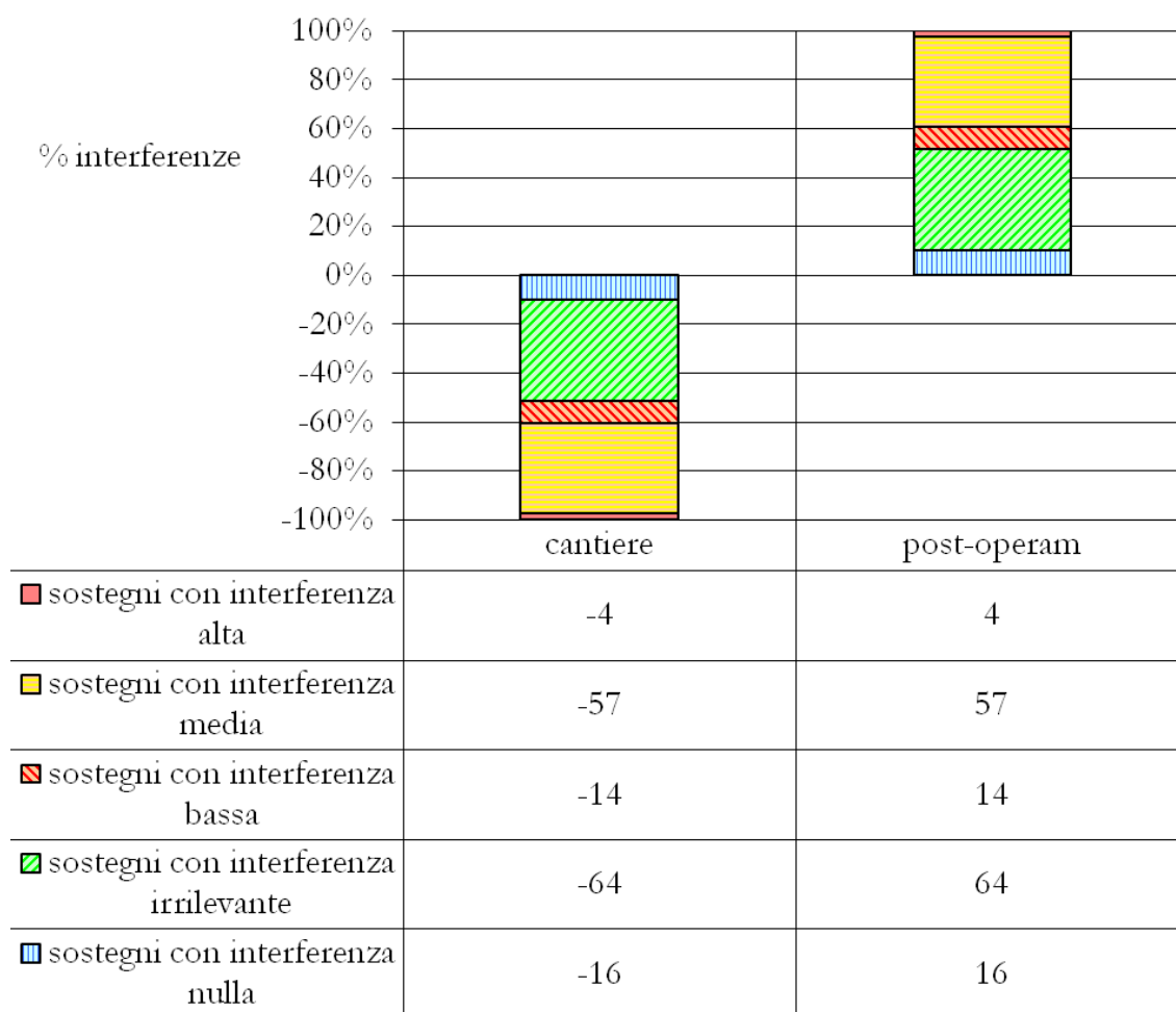
Figura 20 - quantificazione delle interferenze sulle componenti biotiche a seguito della demolizione dei sostegni esistenti da non sostituire
