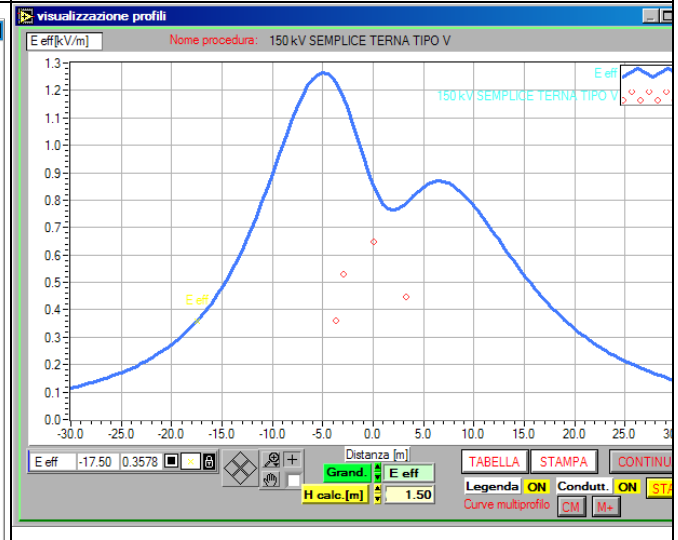
Campo elettrico inferiore a 3.4kV/m
