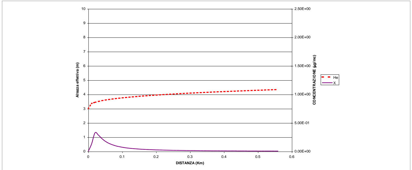
Figura 17 - ricadute al suolo per atmosfera neutra (He = elevation (distanza dal suolo delle particelle emesse) X = funzione di concentrazione del particolato)
