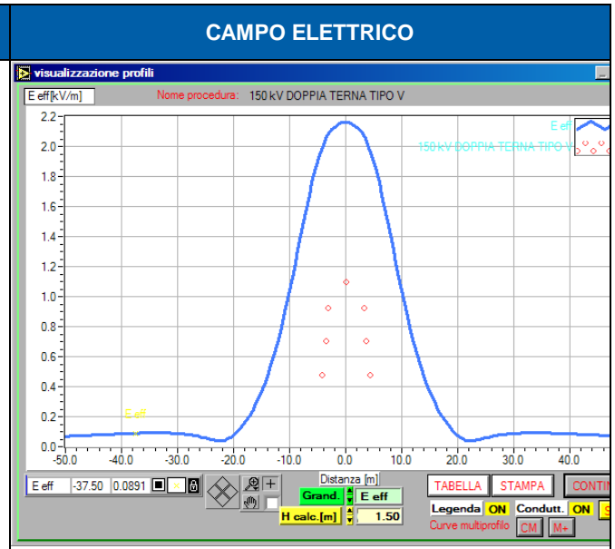
Campo elettrico inferiore a 3.4kV/m
