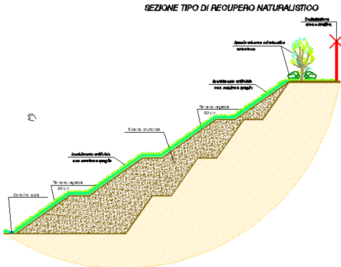
Figura 1-2 Sezione tipo scarpate di recupero agronomico-naturalistico.
