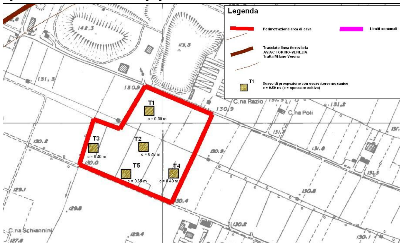
Figura 1-30: Localizzazione delle trincee geognostiche.
