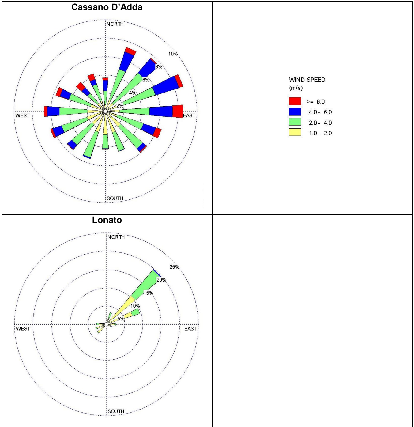
Figura 1-11 Rose dei venti annuali relative alle stazioni meteorologiche – serie storica.
