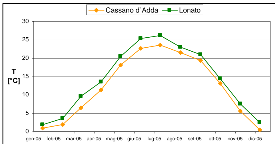
Figura 1-14 Andamento delle temperature medie mensili relative alle stazioni di Cassano d'Adda e Lonato – serie 2005.
