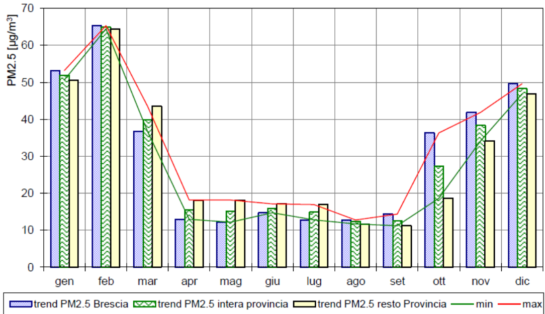
Figura 1-25 Trend mensile PM2.5 Brescia e Provincia 2012
