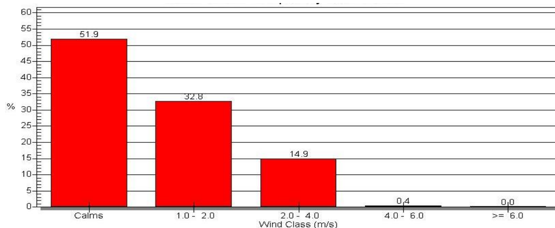
Figura 1-10 Distribuzione delle classi di velocità relativa ai dati meteorologici di Lonato – serie storica.
