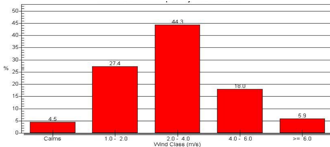
Figura 1-9 Distribuzione delle classi di velocità relativa ai dati meteorologici di Cassano d'Adda – serie storica.
