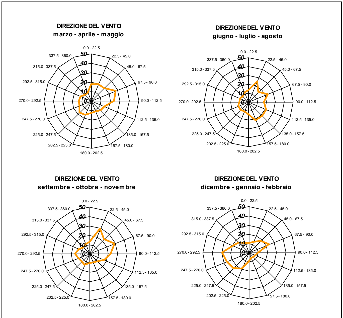
Figura 1-12 Rose dei venti stagionali – Stazione di Cassano d’Adda (frequenze %) – serie storica.
