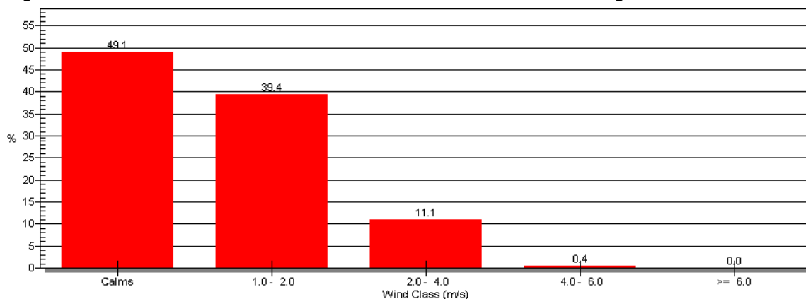
Figura 1-17 Distribuzione delle classi di velocità relativa ai dati meteorologici di Lonato – serie 2005.
