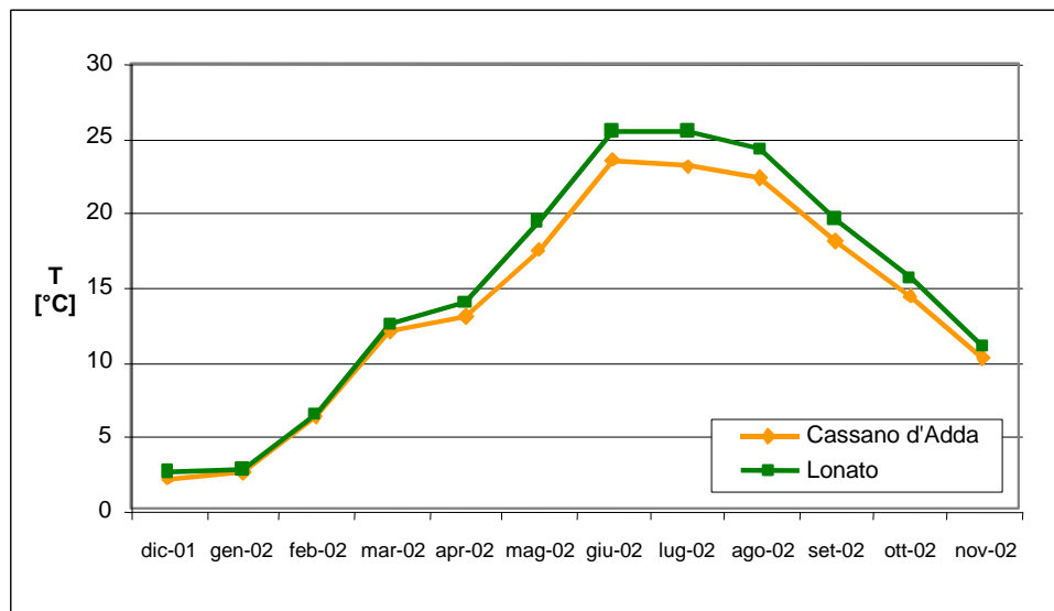
Figura 1-7 Andamento delle temperature medie mensili relative alle stazioni di Cassano d'Adda e Lonato – 1 dicembre 2001 – 30 novembre 2002.
