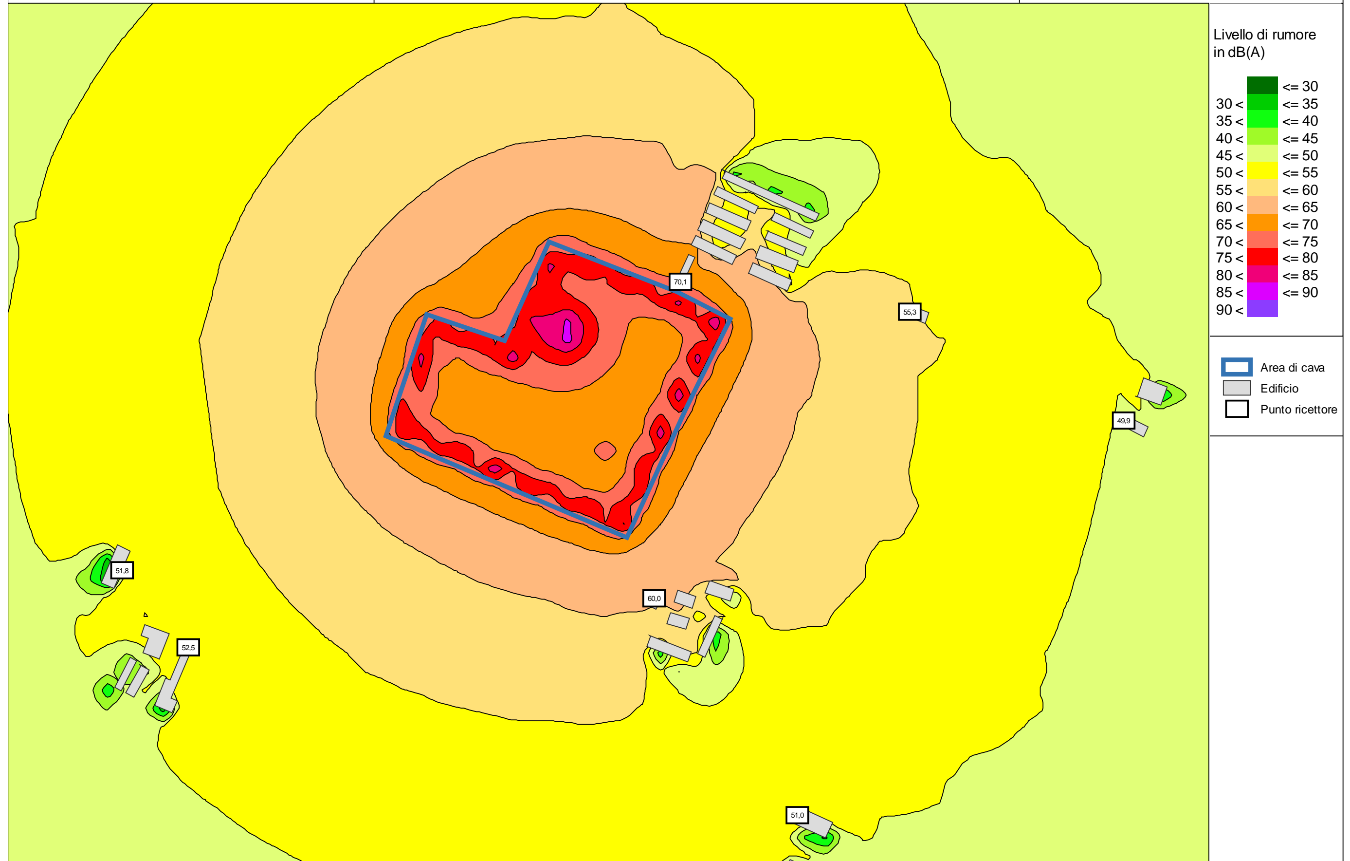
Figura 2-a: Livelli isofonici
