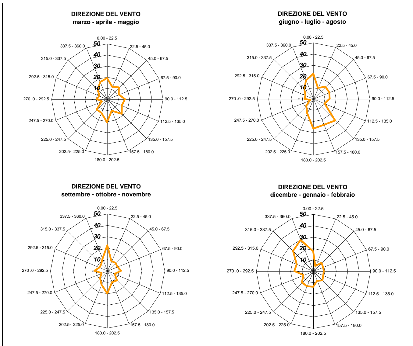
Figura 1-19 Rose dei venti stagionali – Stazione di Cassano d’Adda (frequenze %) – serie 2005.
