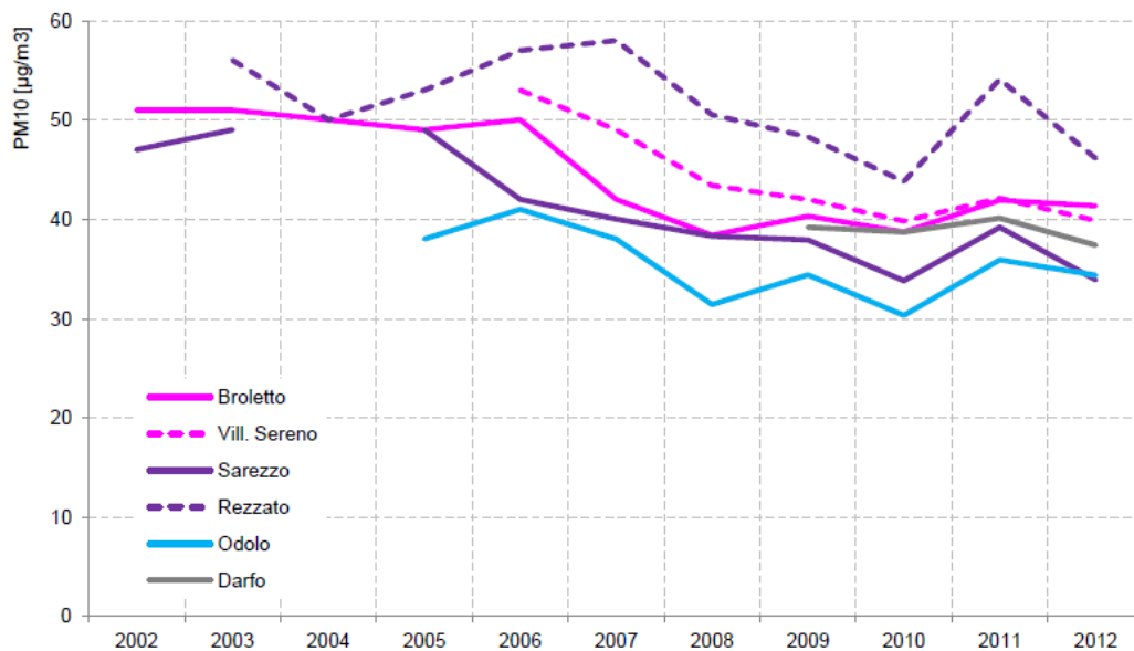
Figura 1-24 Trend PM10 Brescia e Provincia.
