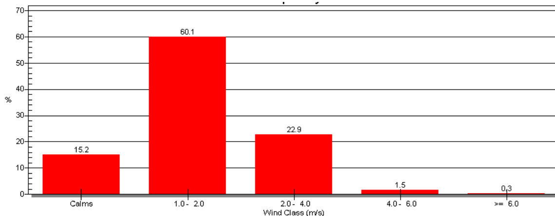
Figura 1-16 Distribuzione delle classi di velocità relativa ai dati meteorologici di Cassano d'Adda – serie 2005.
