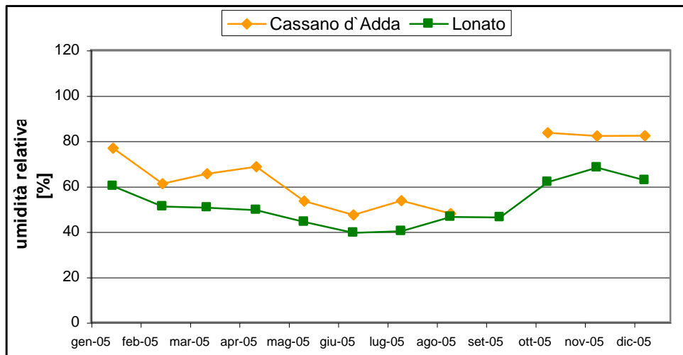
Figura 1-15 Andamento dell'umidità media mensile relativa alle stazioni di Cassano d'Adda e Lonato – serie 2005.
