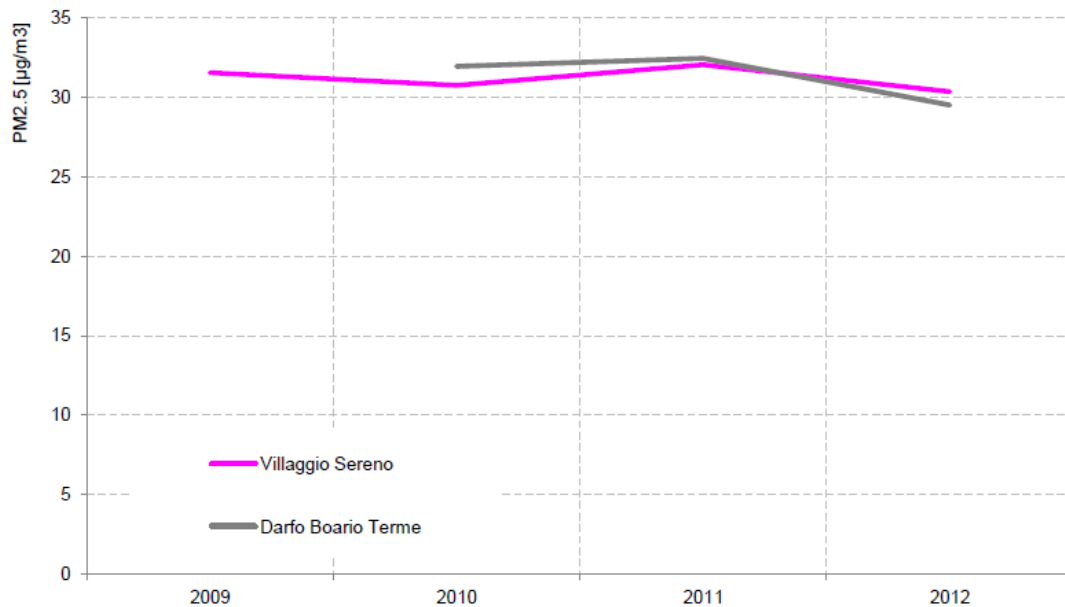
Figura 1-26 Trend PM2.5 Brescia e Provincia.
