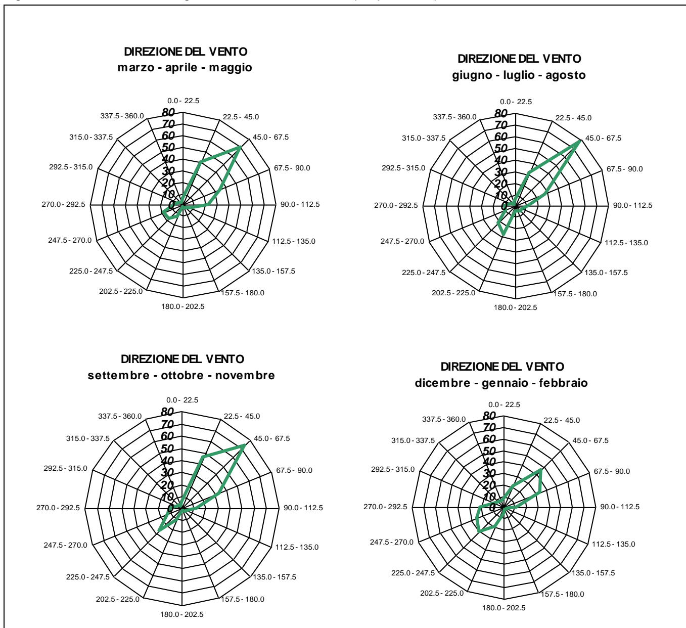
Figura 1-13 Rose dei venti stagionali – Stazione di Lonato (frequenze %) – serie storica.
