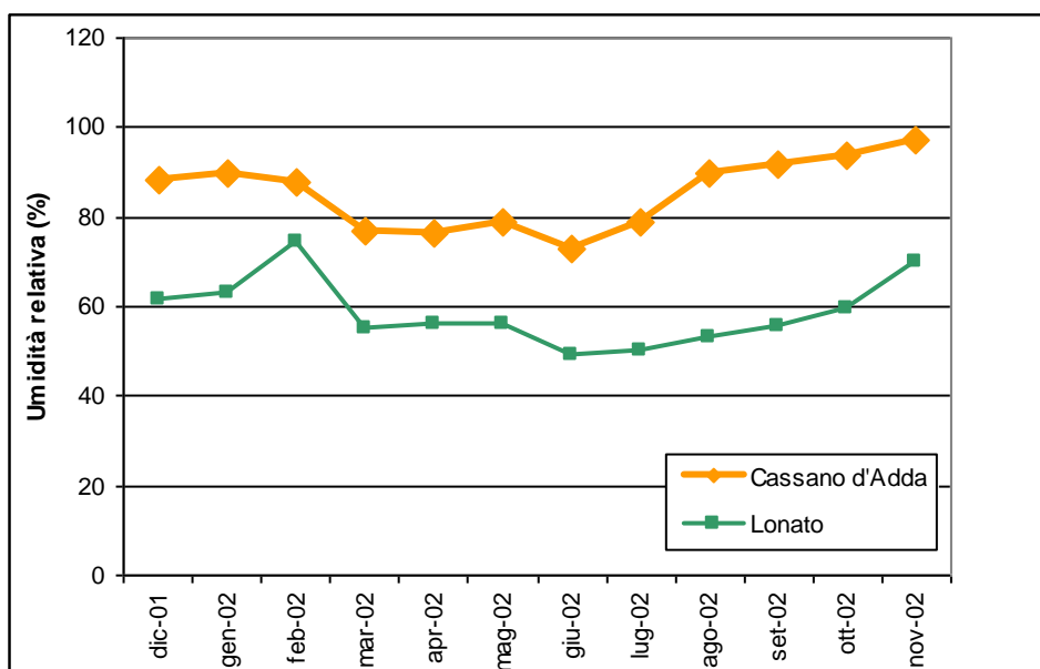
Figura 1-8 Andamento dell'umidità media mensile relativa alle stazioni di Cassano d'Adda e Lonato – 1 dicembre 2001 – 30 novembre 2002.
