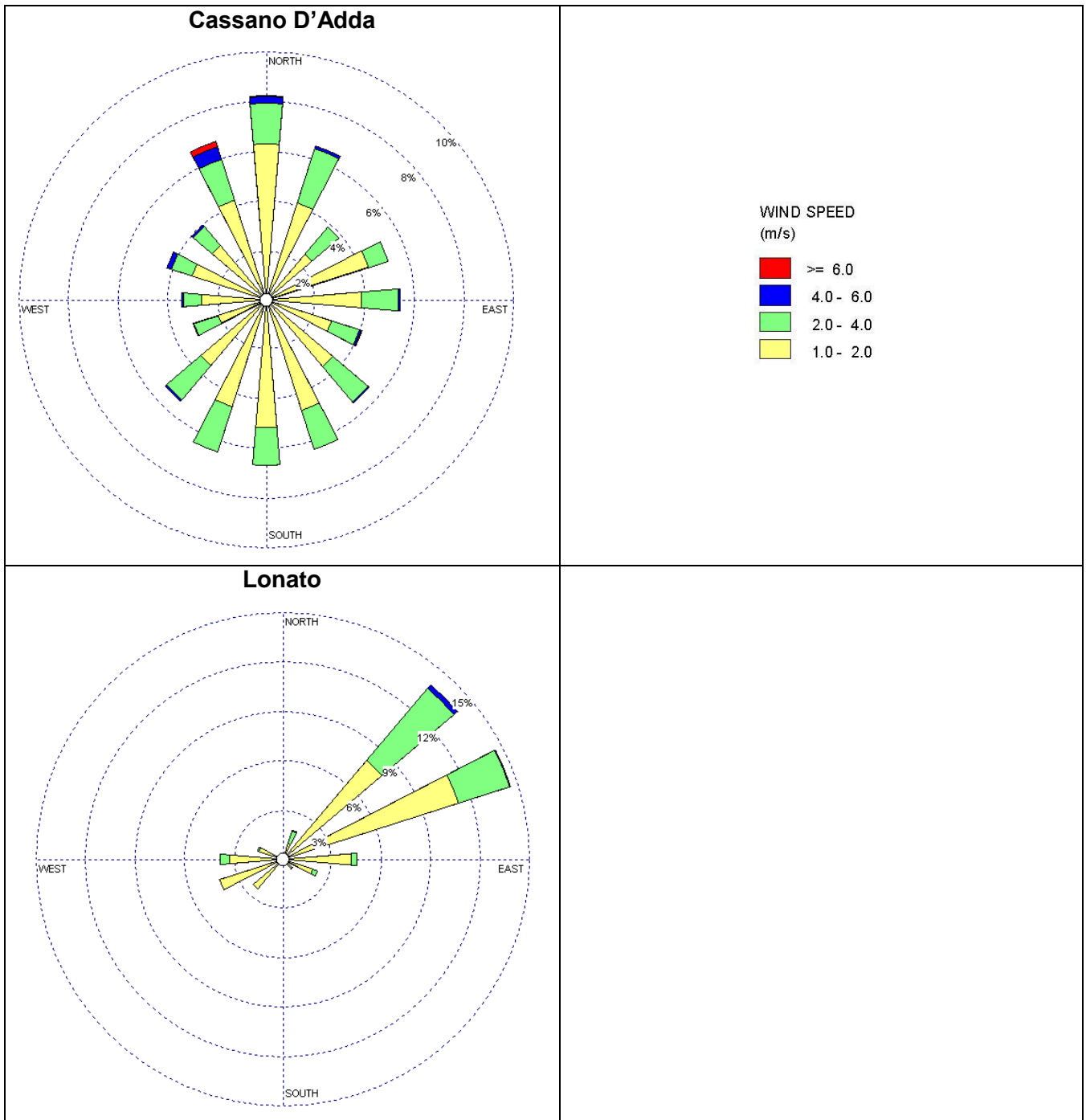
Figura 1-18 Rose dei venti annuali relative alle stazioni meteorologiche – serie 2005.
