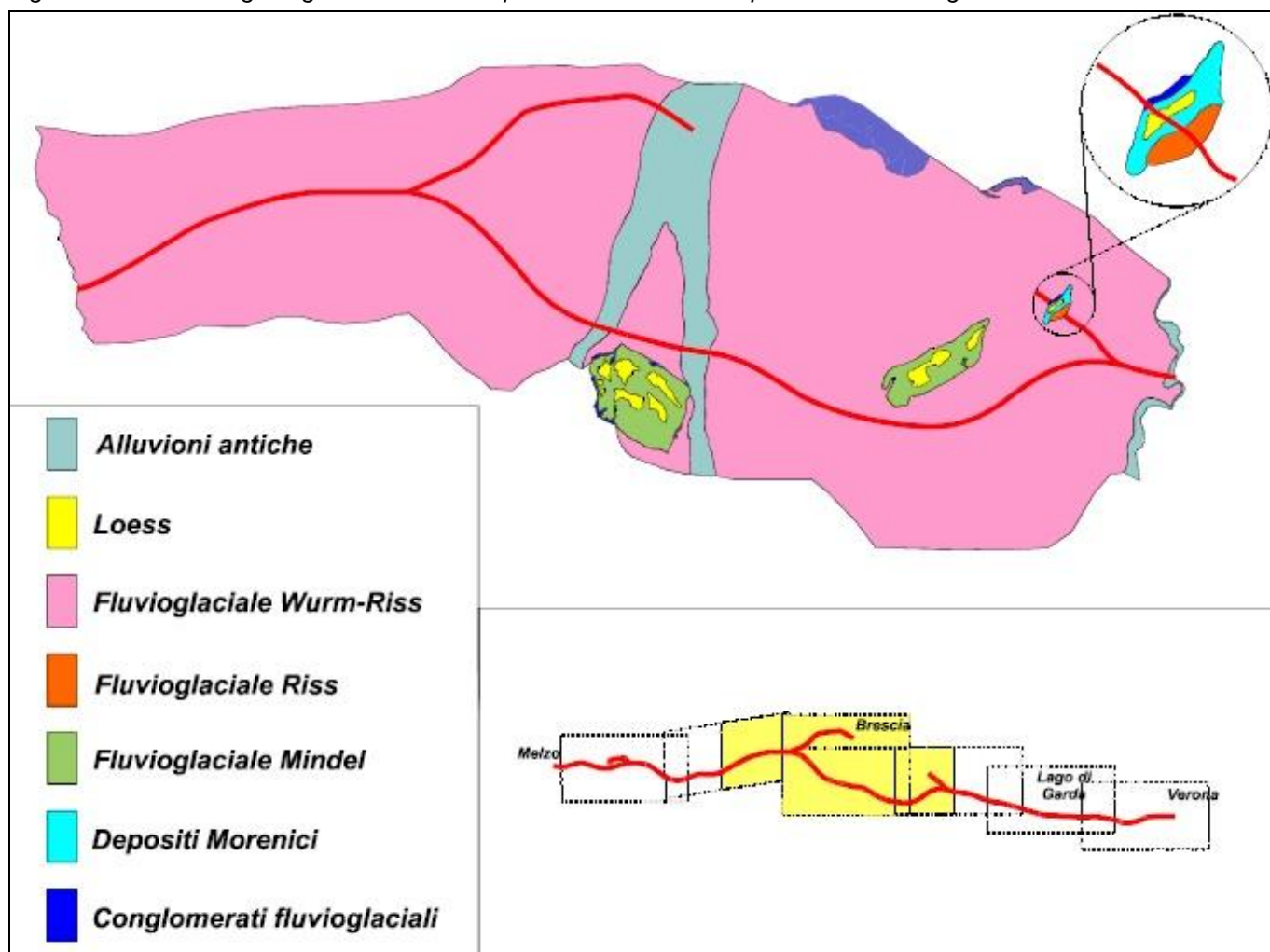
Figura 1-29 Schema geologico del settore di pianura lombarda compreso tra i fiumi Oglio e Chiese.
