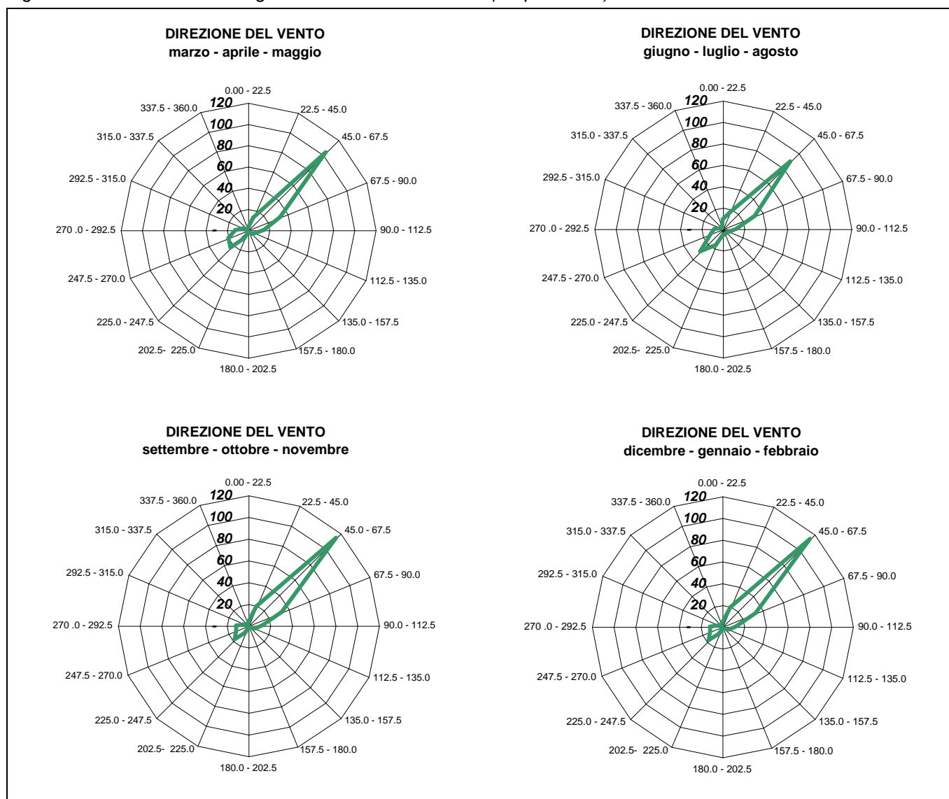
Figura 1-20 Rose dei venti stagionali – Stazione di Lonato (frequenze %) - serie 2005.
