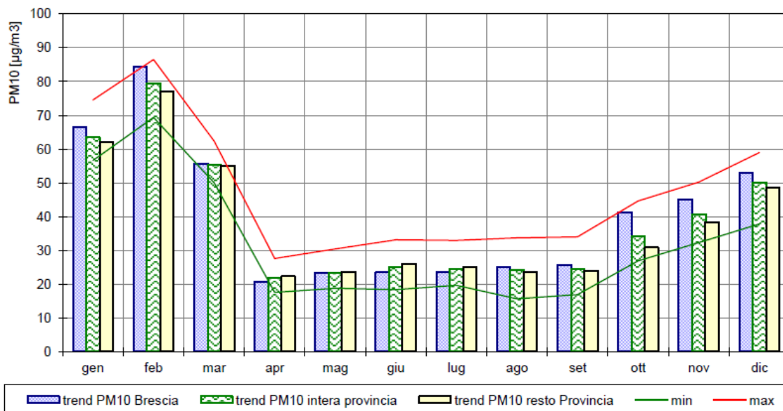
Figura 1-23 Trend mensile PM10 Brescia e Provincia 2012
