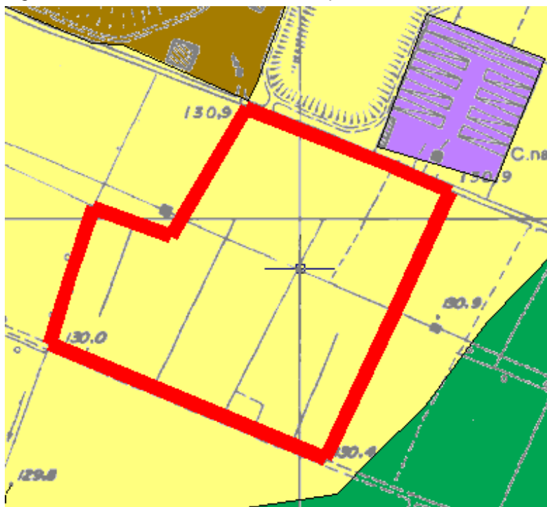
Figura 1-32: Estratto della carta della capacità d'uso dei suoli 04 – IP – C – 32040-01.
