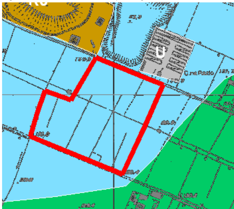
Figura 1-31: Estratto della carta pedologica 04 – IP – C – 32039-01.
