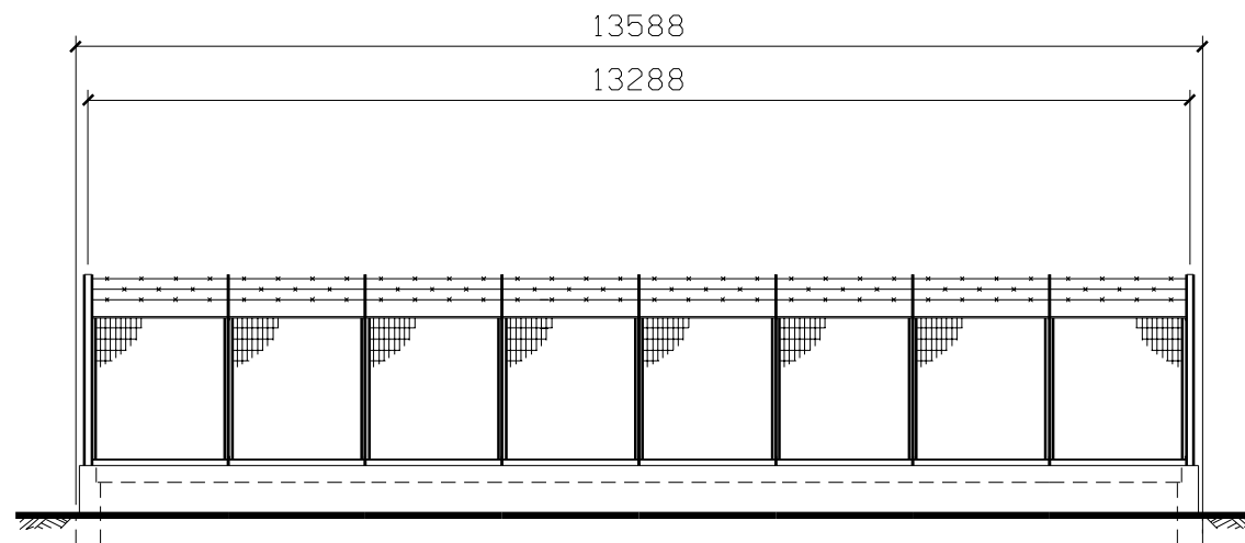
PROSPETTO B
