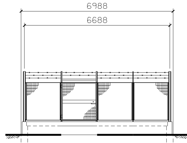
PROSPETTO A
