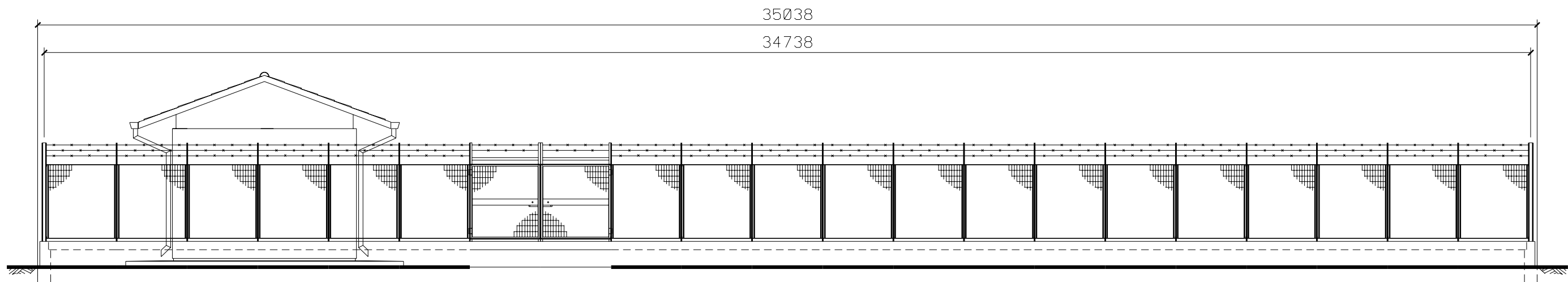
PROSPETTO A
