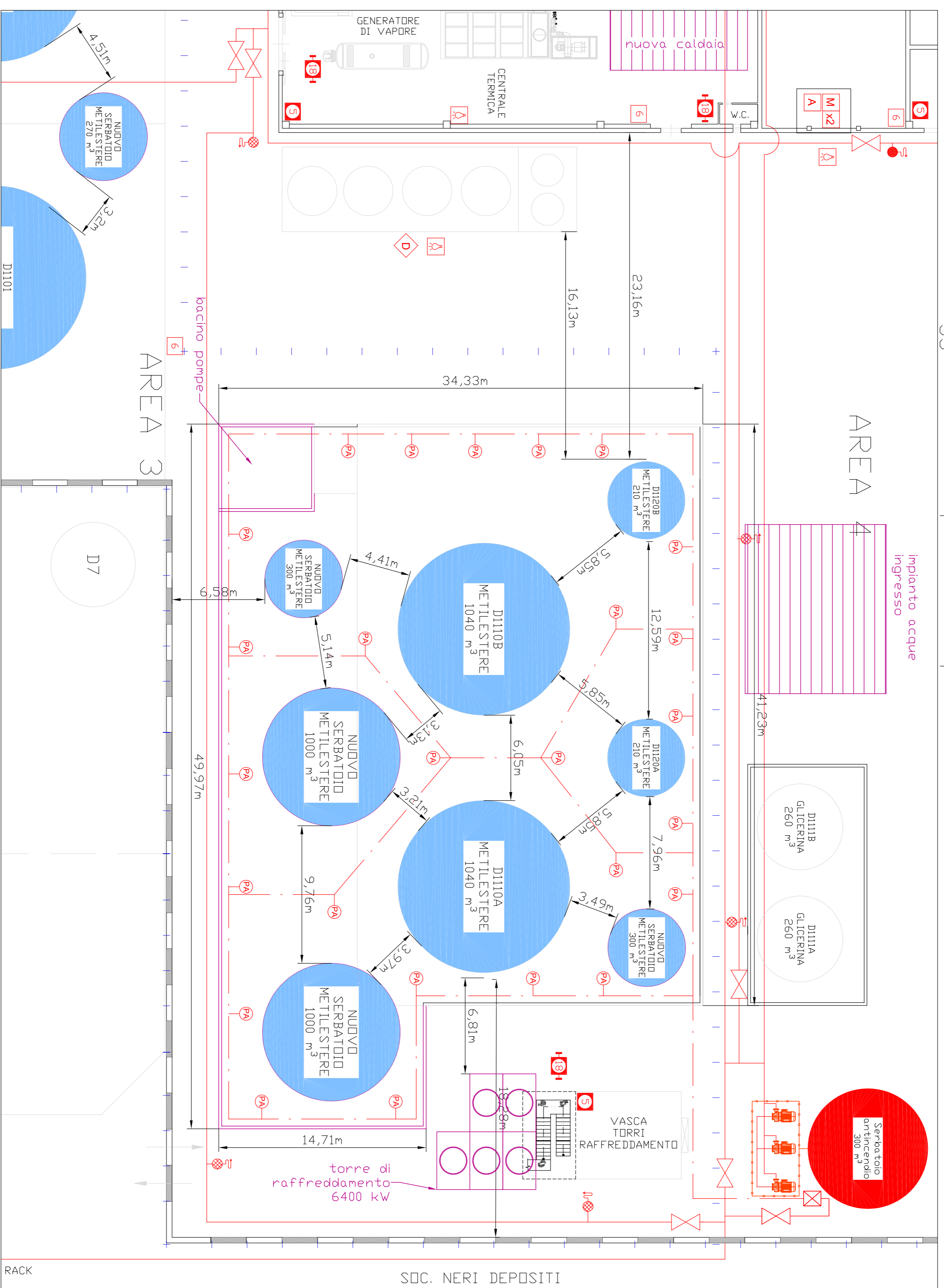
Area 3 - Area di stoccaggio Biodiesel (ipotesi di ampliamento)
