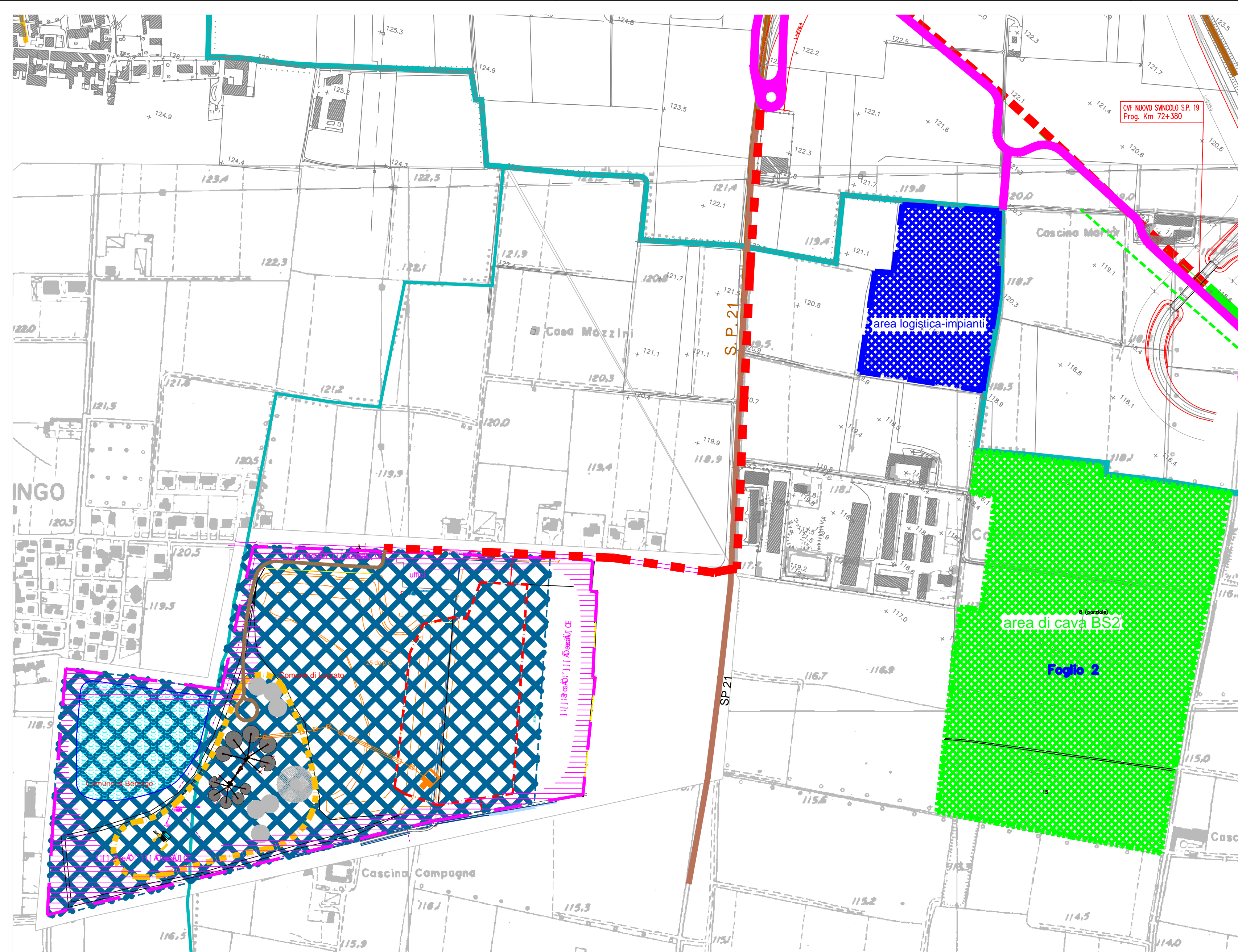
ESTRATTO DALLA CARTA GEOLOGICA
