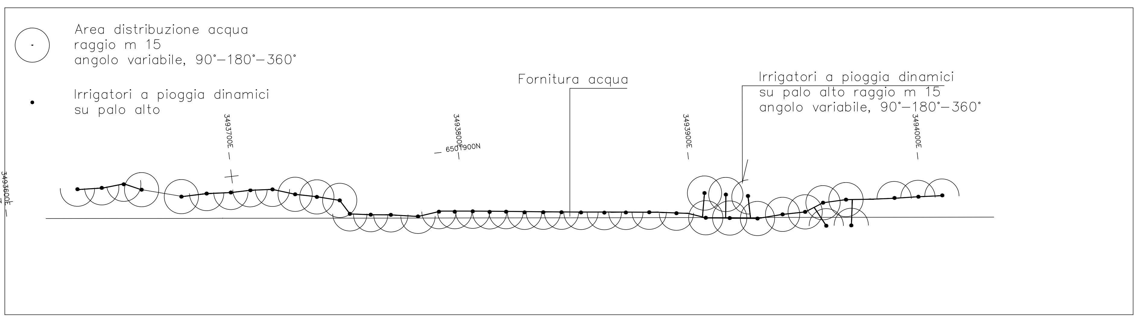
2 Schema d'impianto d'irrigazione: planimetria Scala 1:2000
