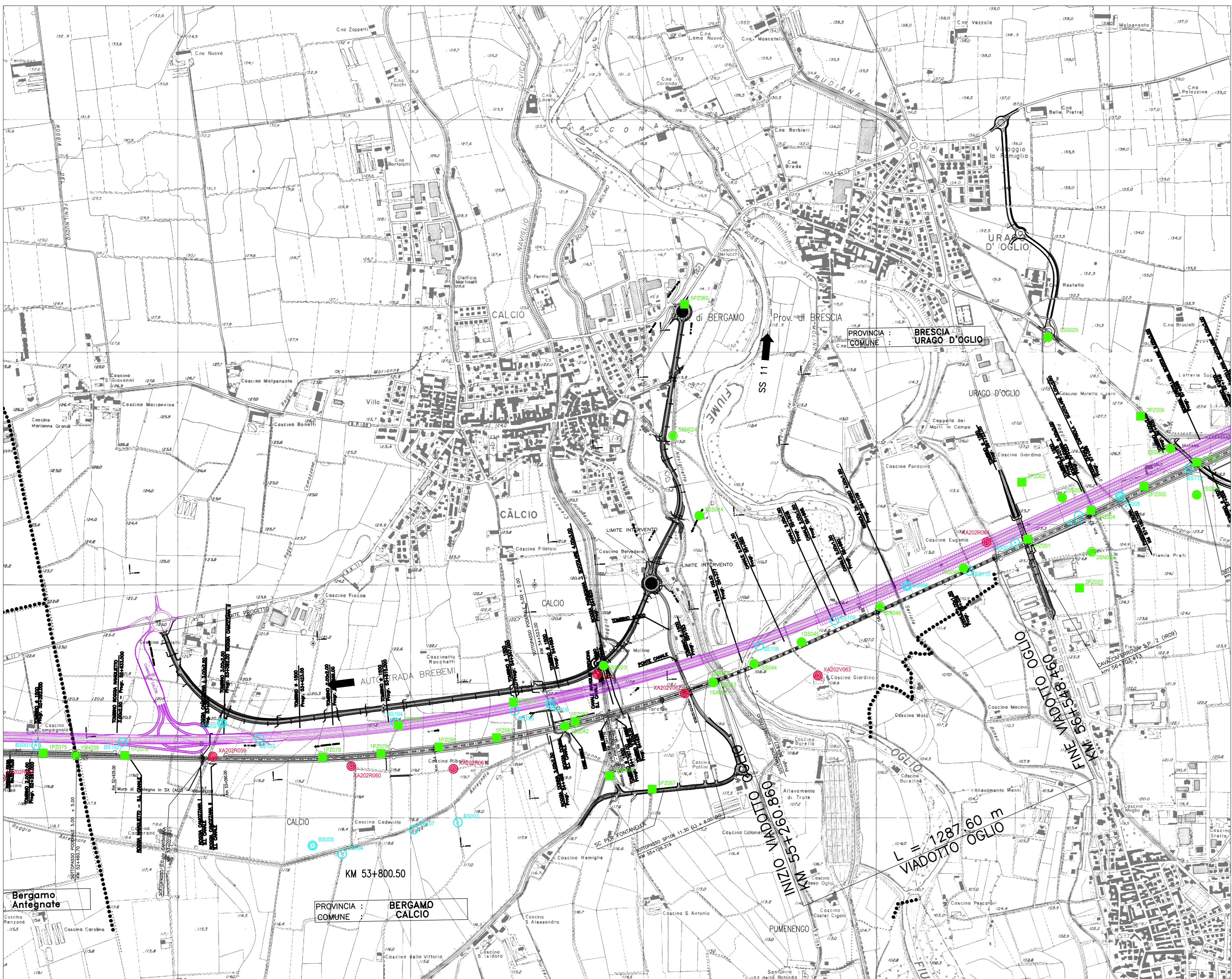
VIABILITA' DALLA PK 52+000 ALLA PK 58+000 DELLA LINEA AV/AC
