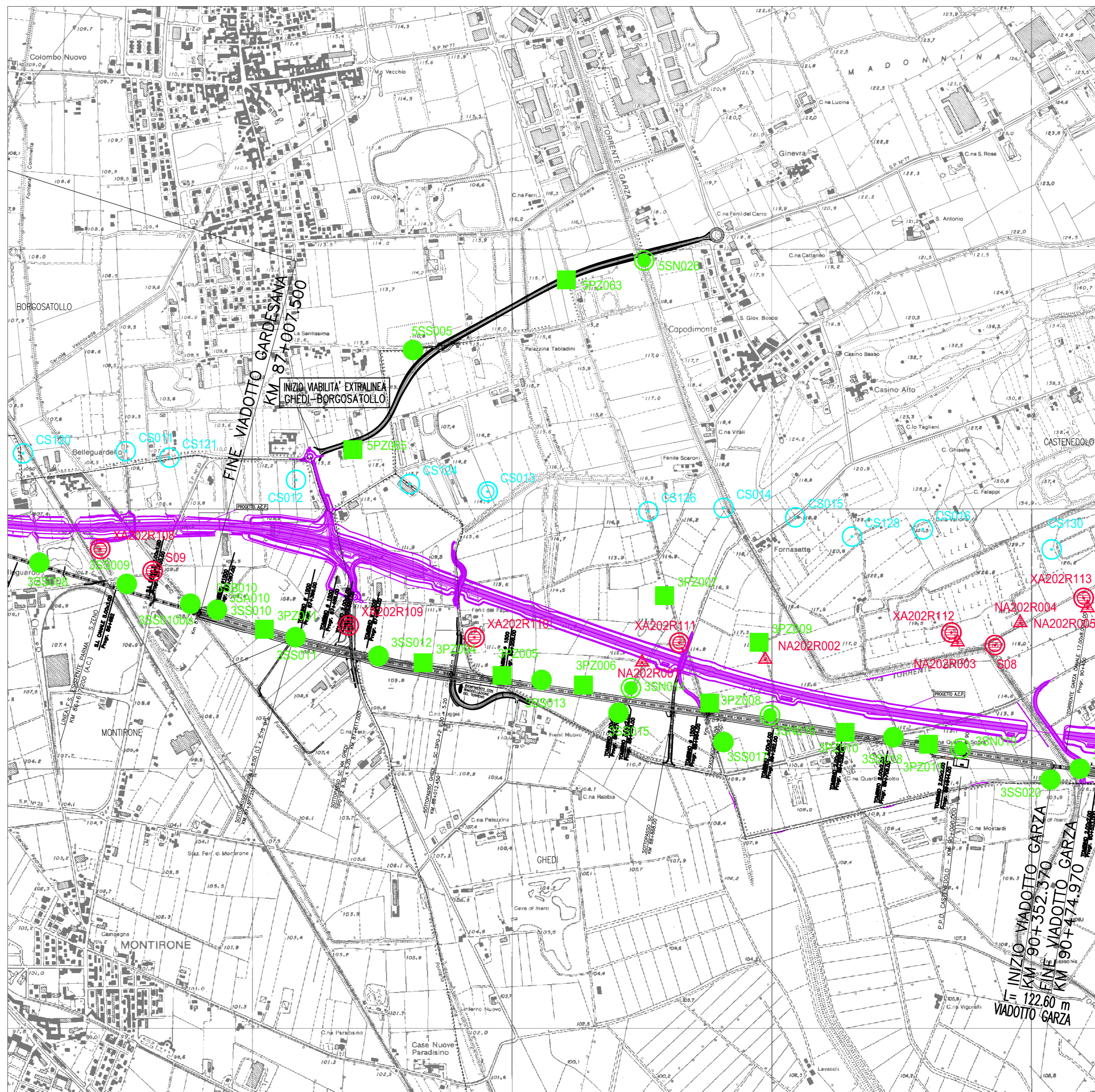
VIABILITA' DALLA PK 87+000 ALLA PK 90+000 DELLA LINEA AV/AC
