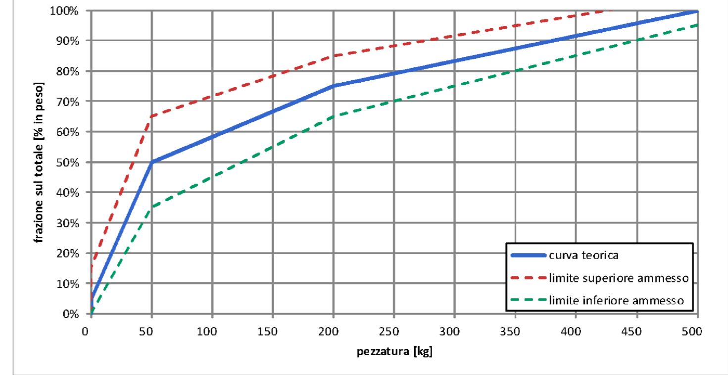
Fuso di distribuzione del peso
