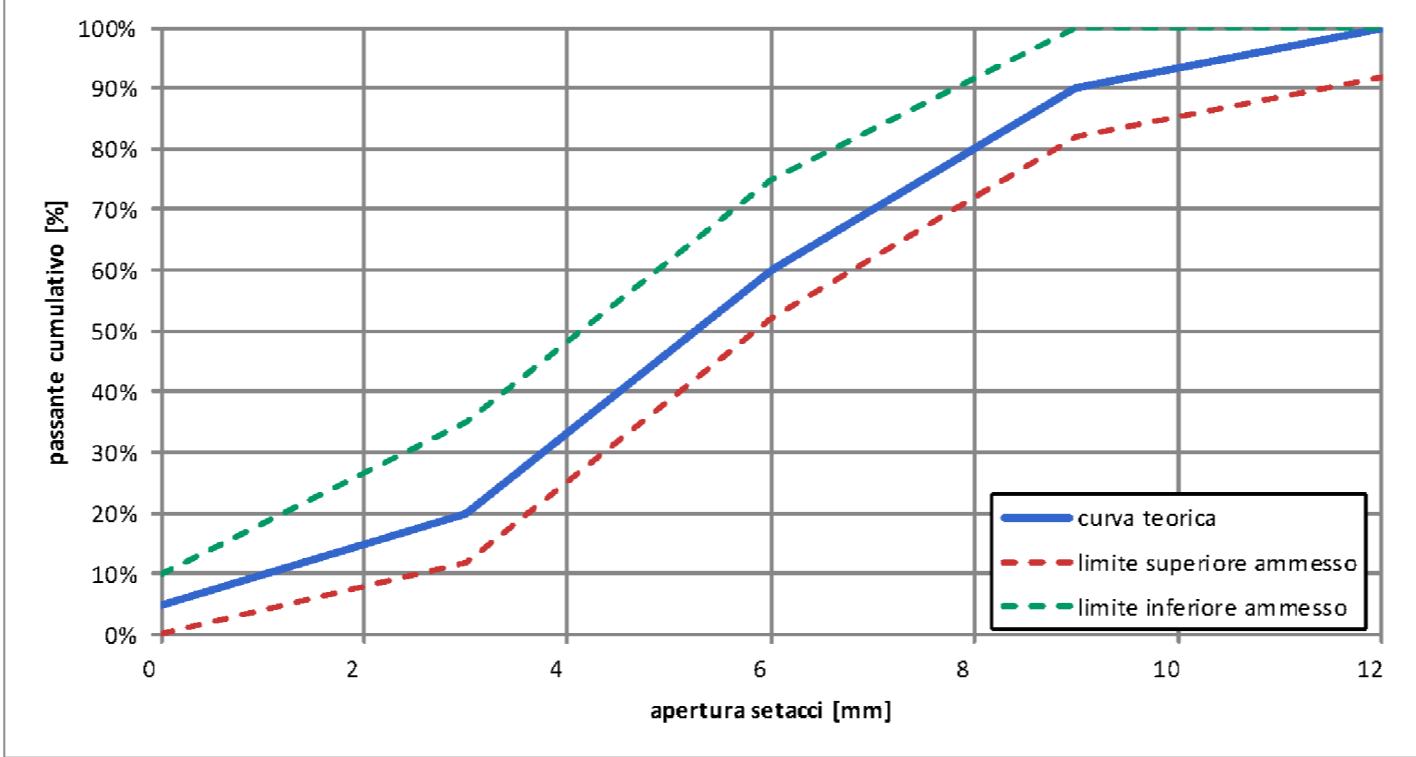
Fuso di distribuzione del diametro dei grani
