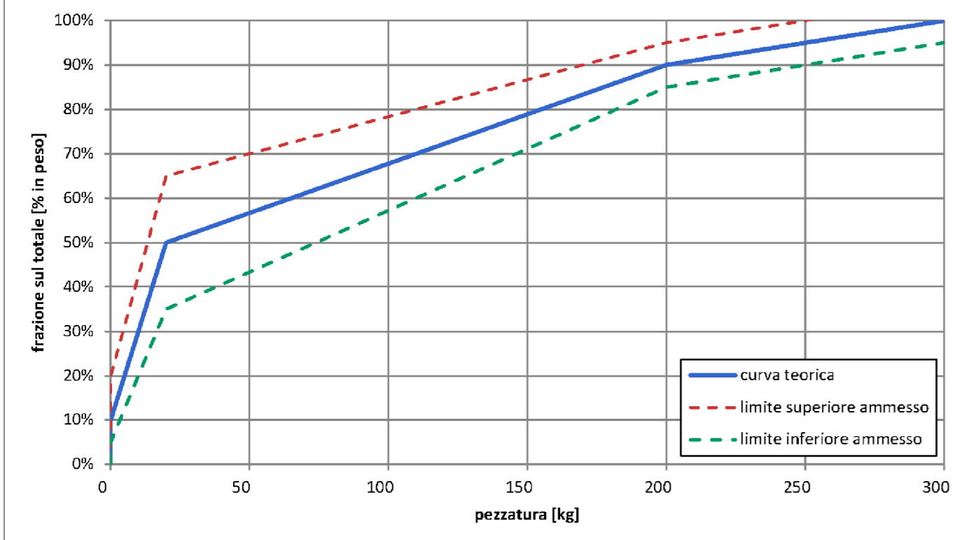
Fuso di distribuzione del peso
