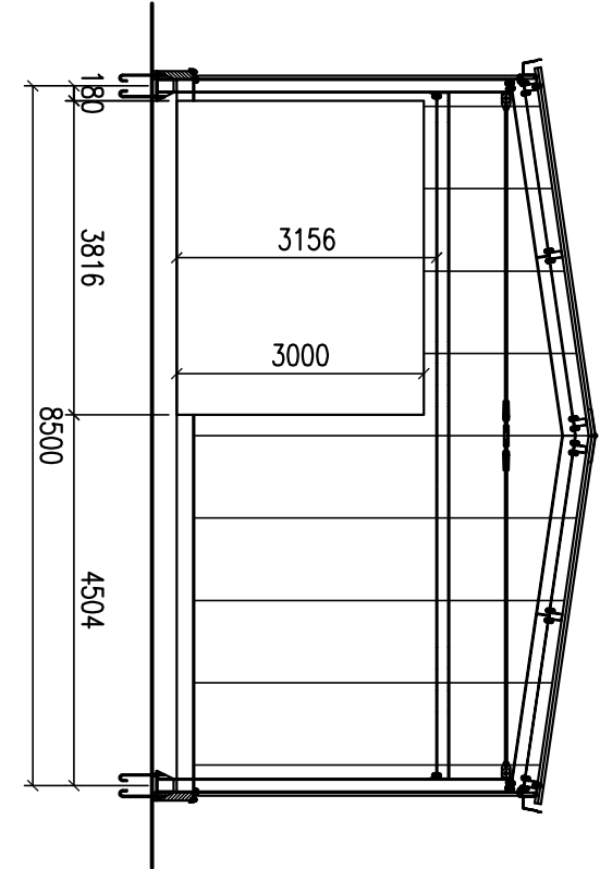
PROSPETTO LATO B
