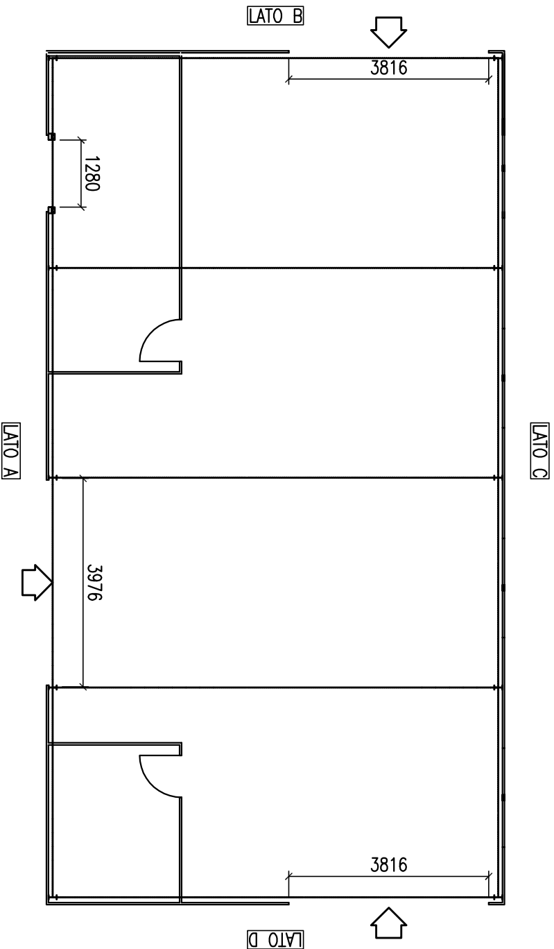
PIANTA DISTRIBUZIONE INTERNA
