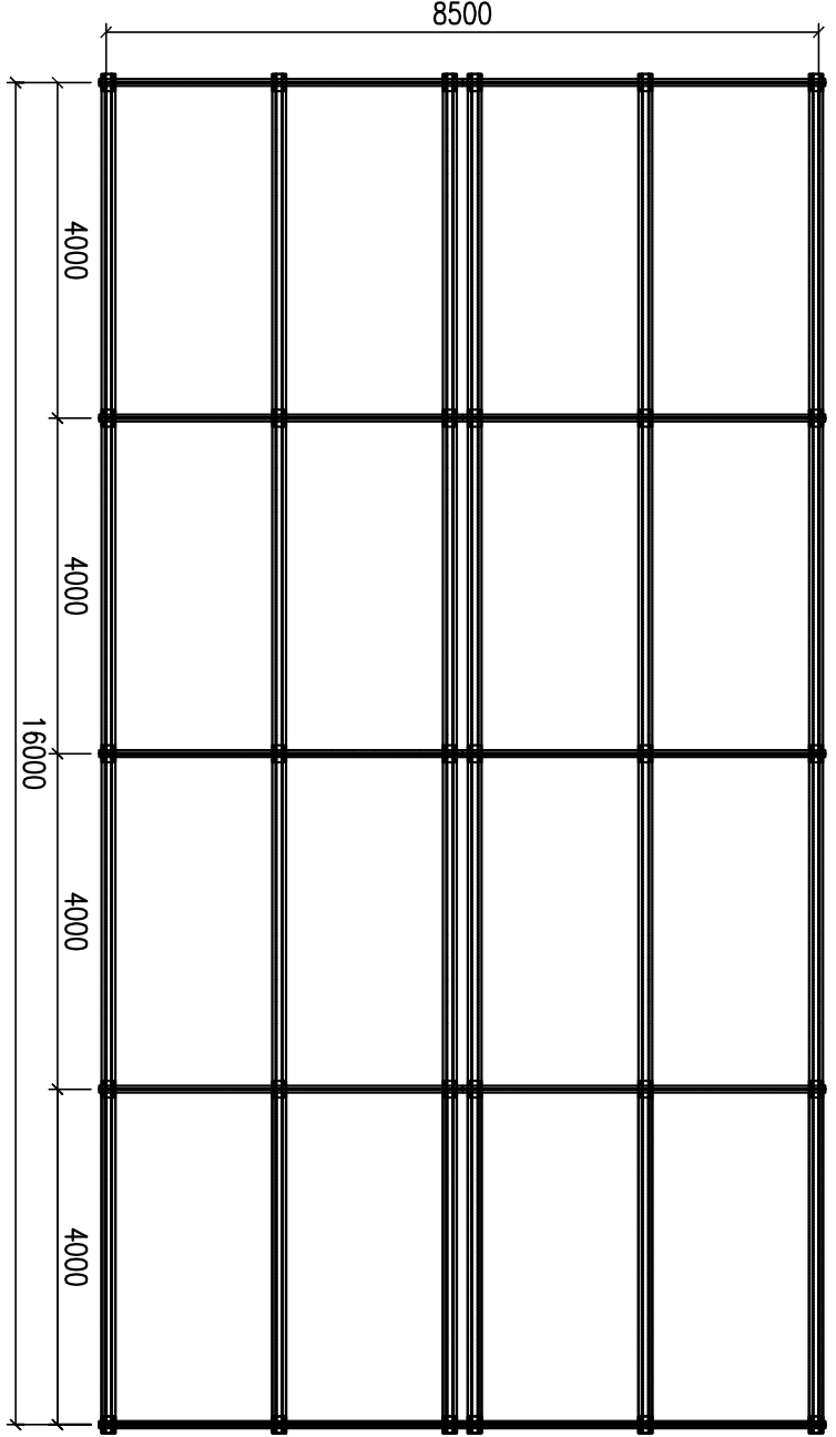
PIANTA CARPENTERIA COPERTURA
