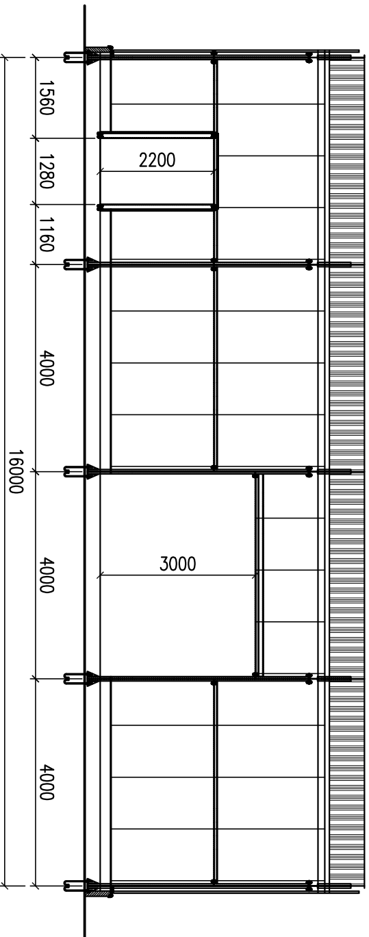
PROSPETTO LATO A
