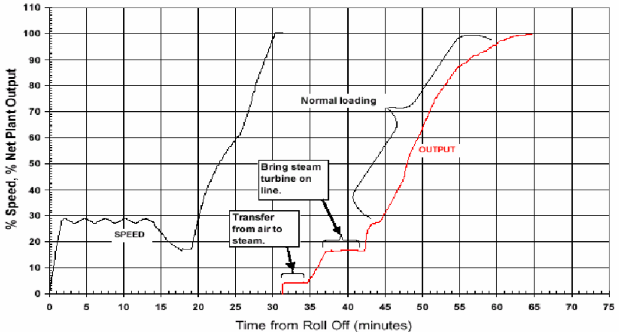
Fig. 3.4 Transitori di avviamento da “freddo”
