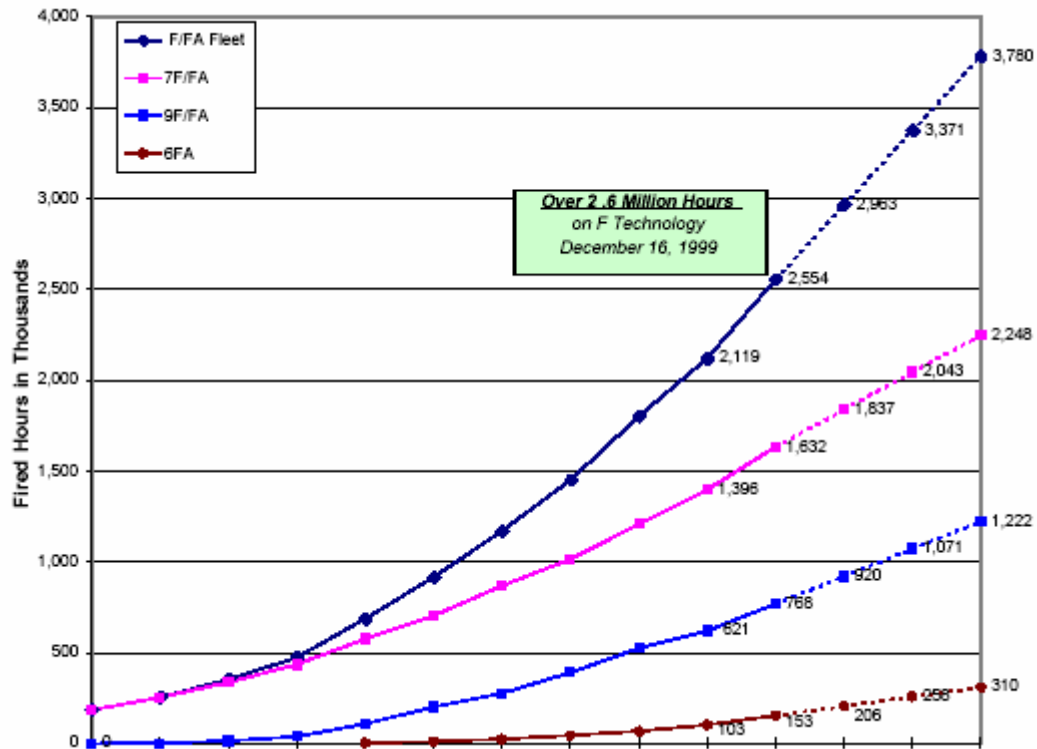
Fig. 3.11 Ore di funzionamento Turbine della classe F di GE
