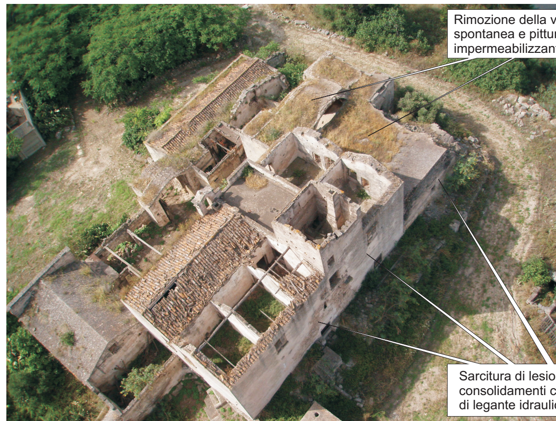
Ripristino coperture in coppi.
