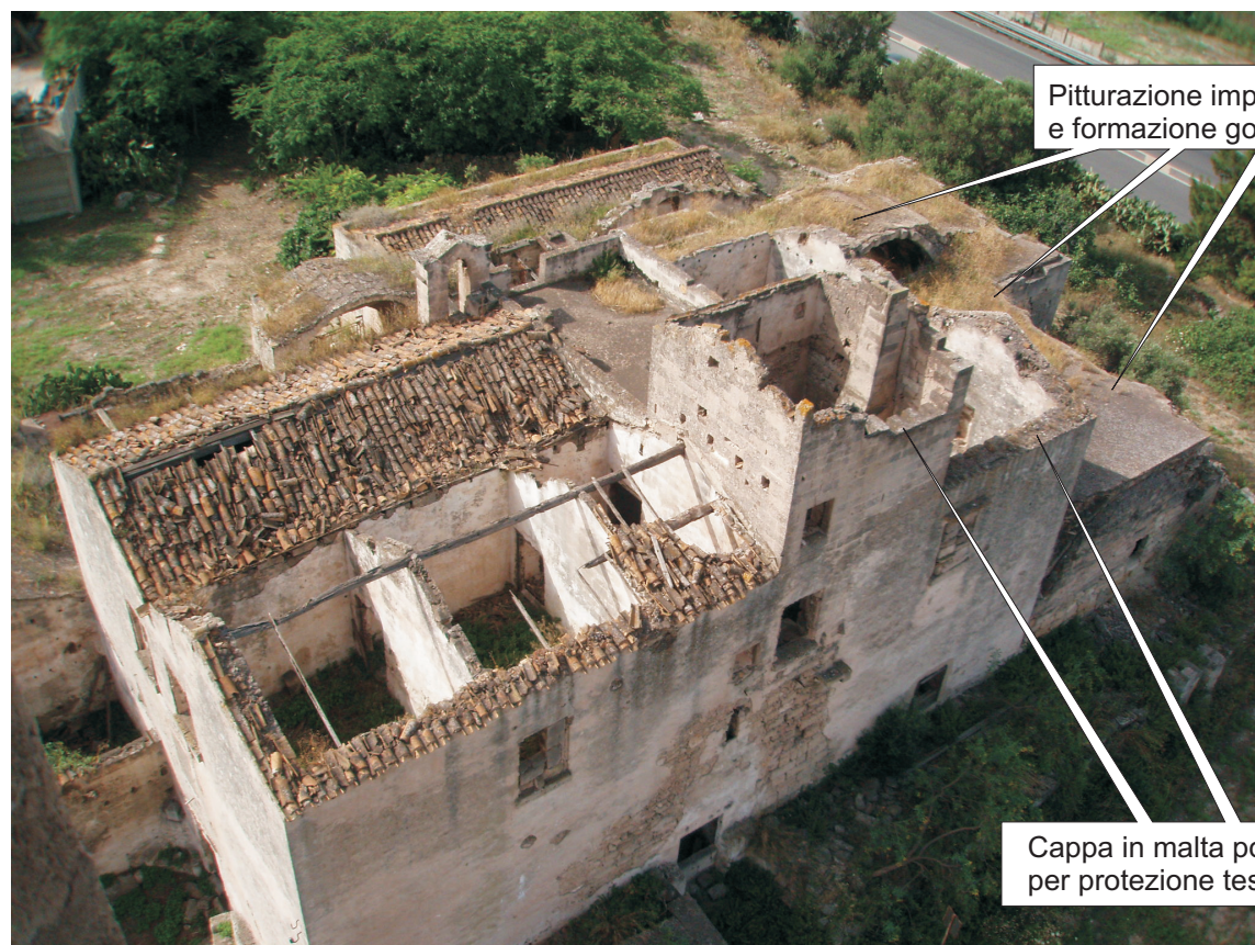
Chiusura con murature in tufo di aperture con piattabanda lesionata o in legno.
