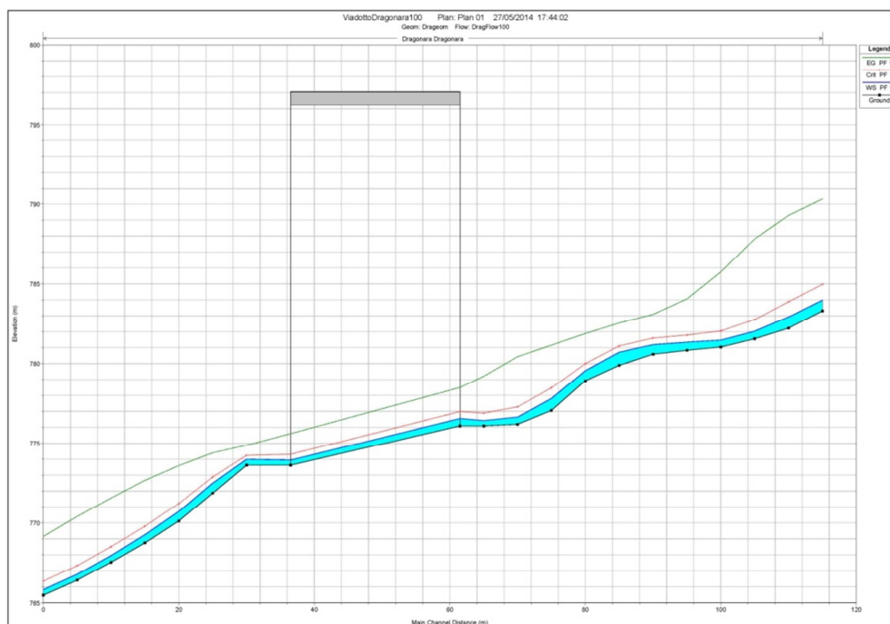
FIGURA 3 - PROFILO Q100
