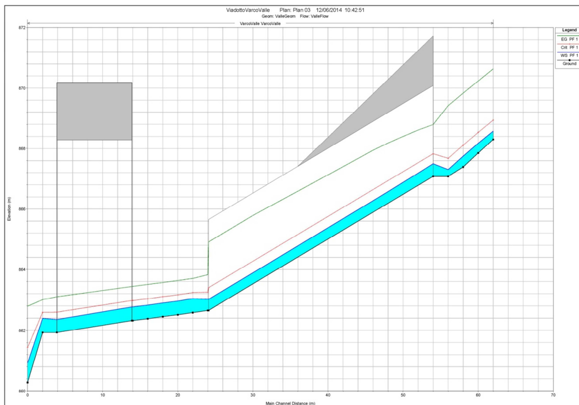
FIGURA 3 - PROFILO Q100
