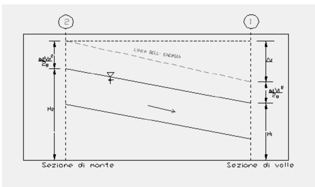
FIGURA 2 - GRANDEZZE PRESENTI NELL'EQUAZIONE DELL'ENERGIA.
