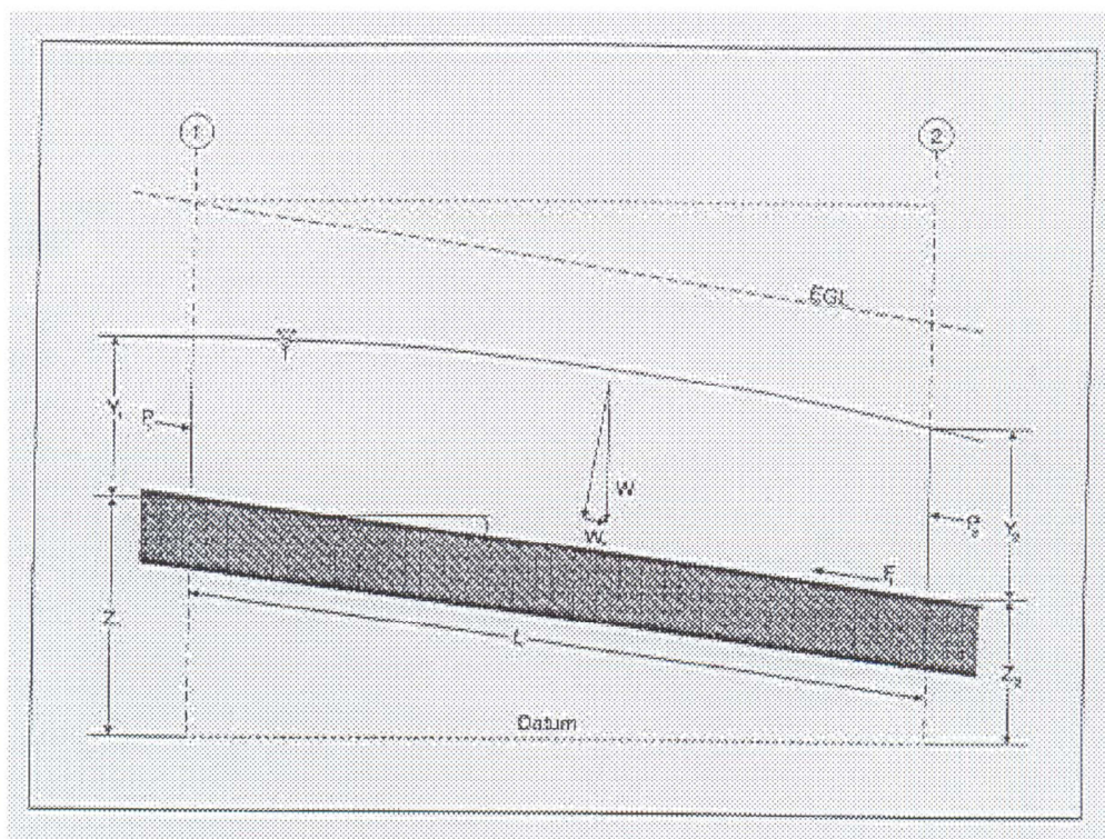
FIGURA 3 - ELEMENTI CARATTERISTICI DELL'EQUAZIONE DEL MOMENTO
