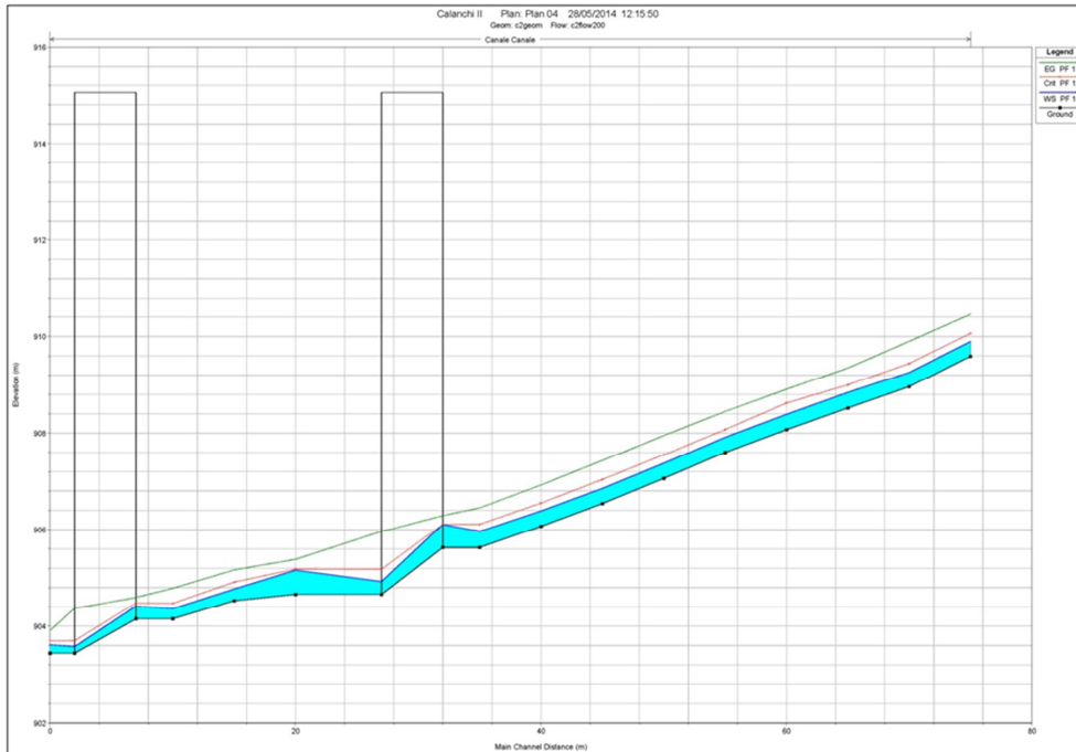
FIGURA 4 - PROFILO Q100
