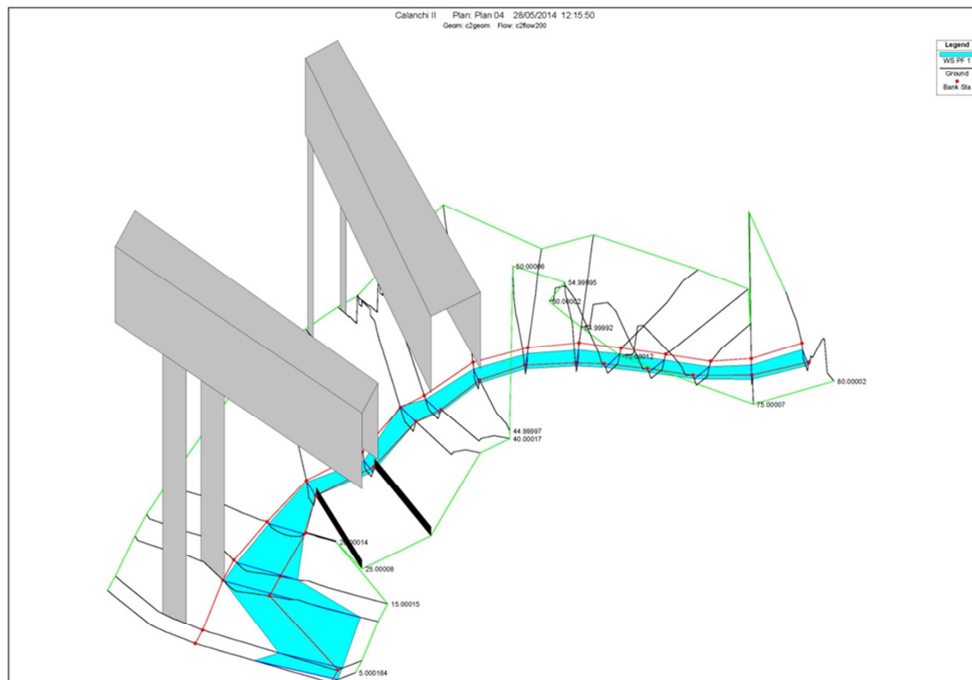
FIGURA 5 - VISTA 3D DEL MODELLO IDRAULICO CORRISPONDENZA DELL'ATTRAVERSAMENTO
