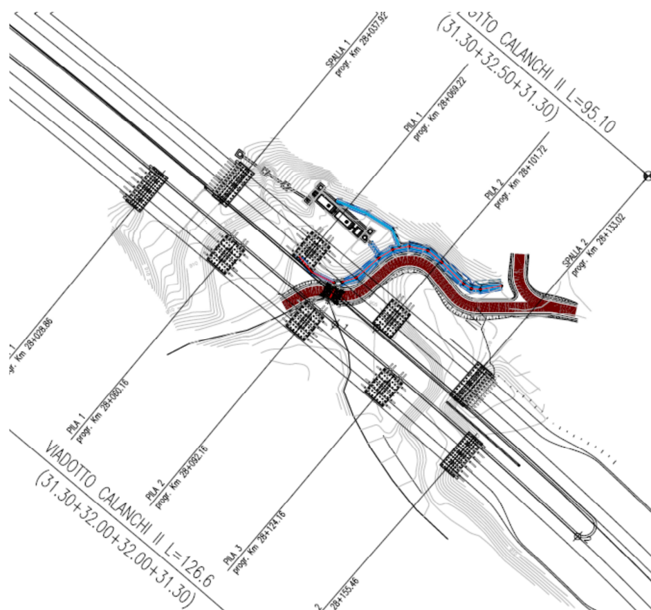
FIGURA 6 – INQUADRAMENTO DELL'INTERVENTO
