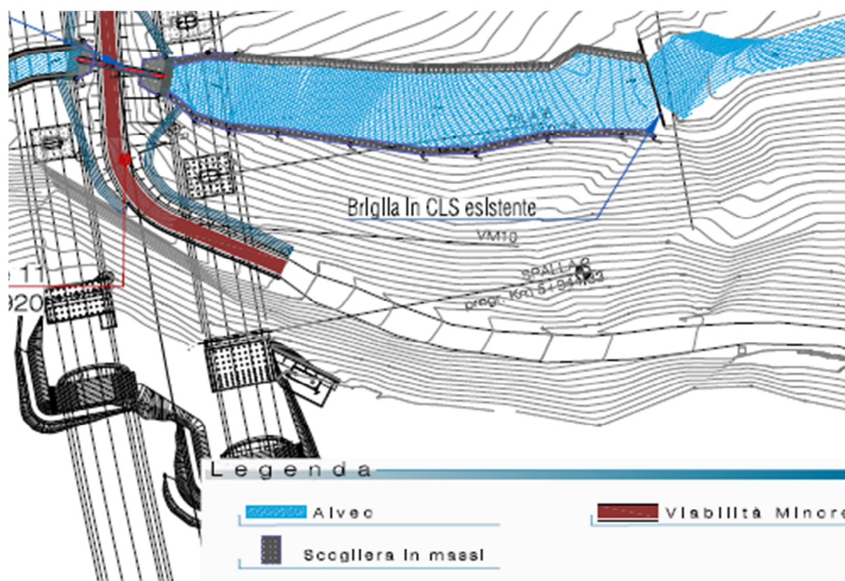
FIGURA 5 – OPERE DI PROTEZIONE SPONDE E DI STRAVERSAMENTO IDRAULICO
