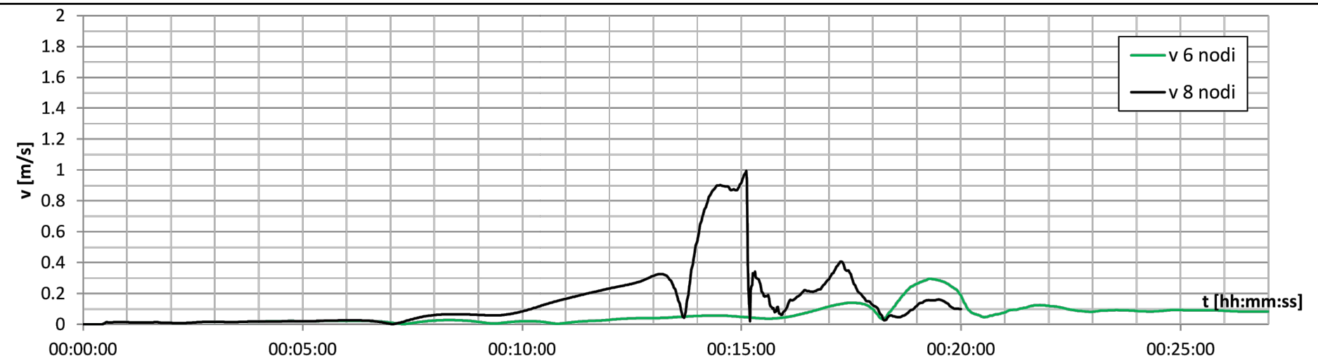
VELOCITA' [m/s]
