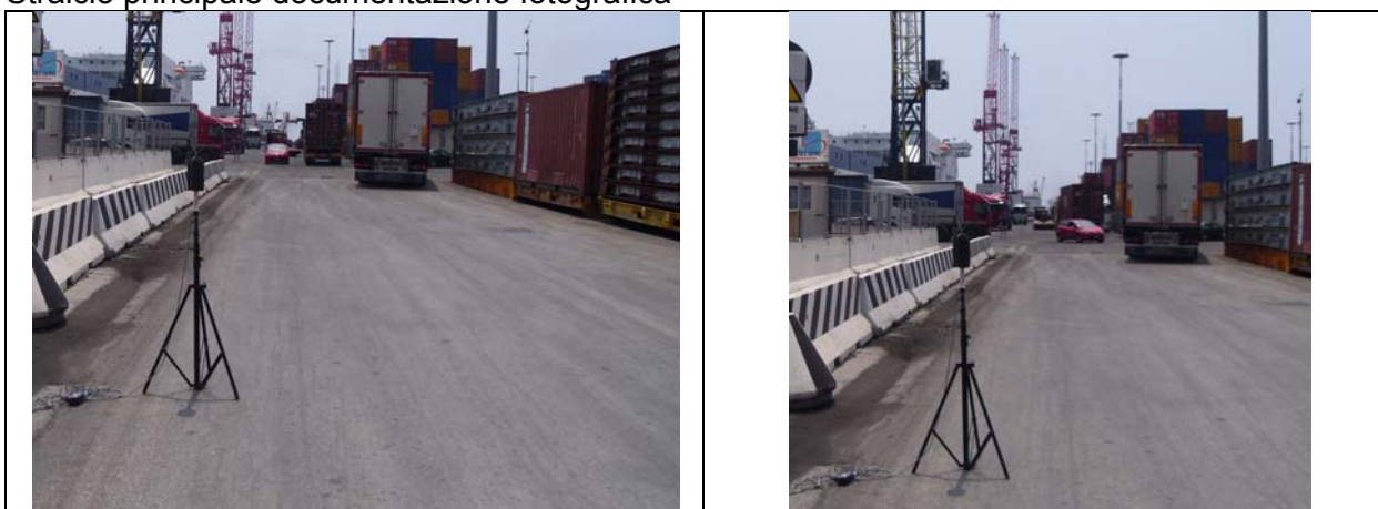
Figura 5.14 – Posizionamento della strumentazione impiegata nel punto R03 (campagna di luglio)
