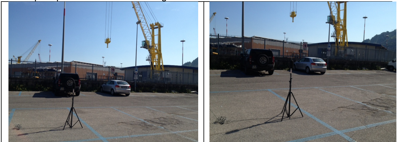
Figura 5.6 - Posizionamento della strumentazione impiegata nel punto R04 (campagna di giugno)
