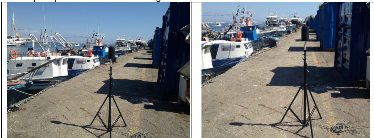
Figura 5.4 – Posizionamento della strumentazione impiegata nel punto R02 (campagna di giugno)
