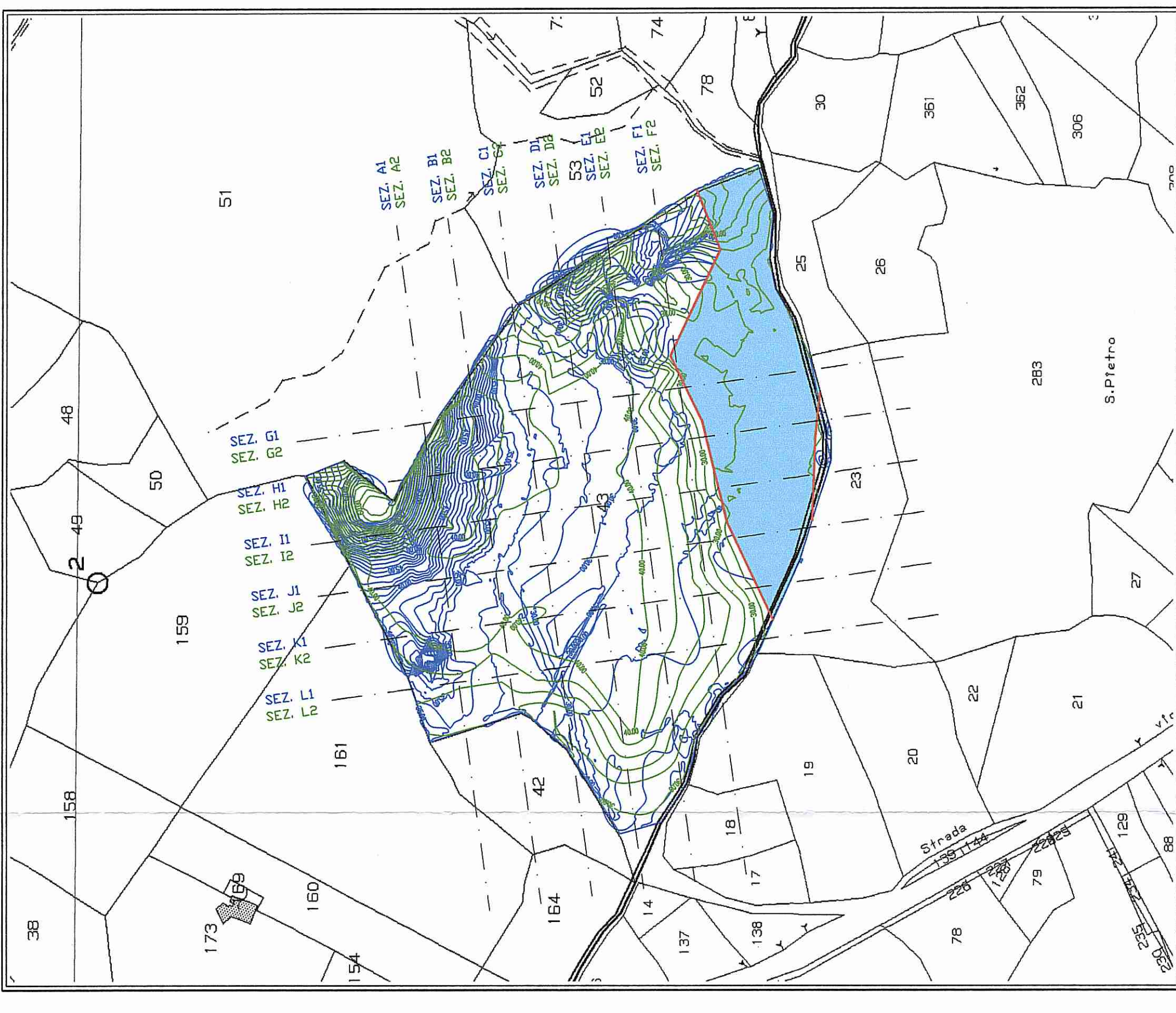
Schema delle sezioni Repp 1:2000
