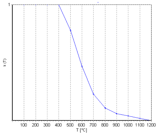
Figure 6: Fattore di riduzione del valore di resistenza f_{yk} per le barre d'armatura (EN 1992-1-2 p.4.2.4.3 – fig.4.2a)
