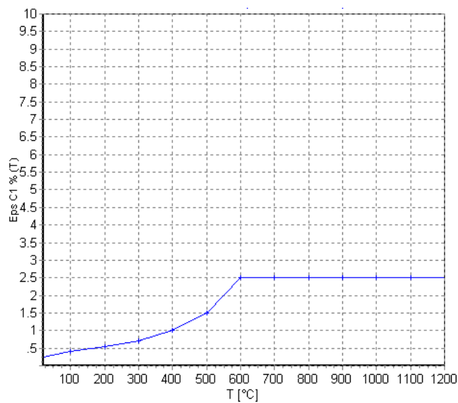
Figure 4: Fattore di riduzione del valore \epsilon_{sc1} per il calcestruzzo (EN 1992-1-2 p.3.2.2.1 – tab.3.1)
