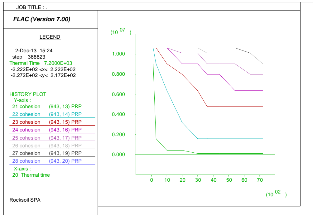
Figura 51 – Evoluzione del valore di coesione c'nel rivestimento – Curva EUREKA
