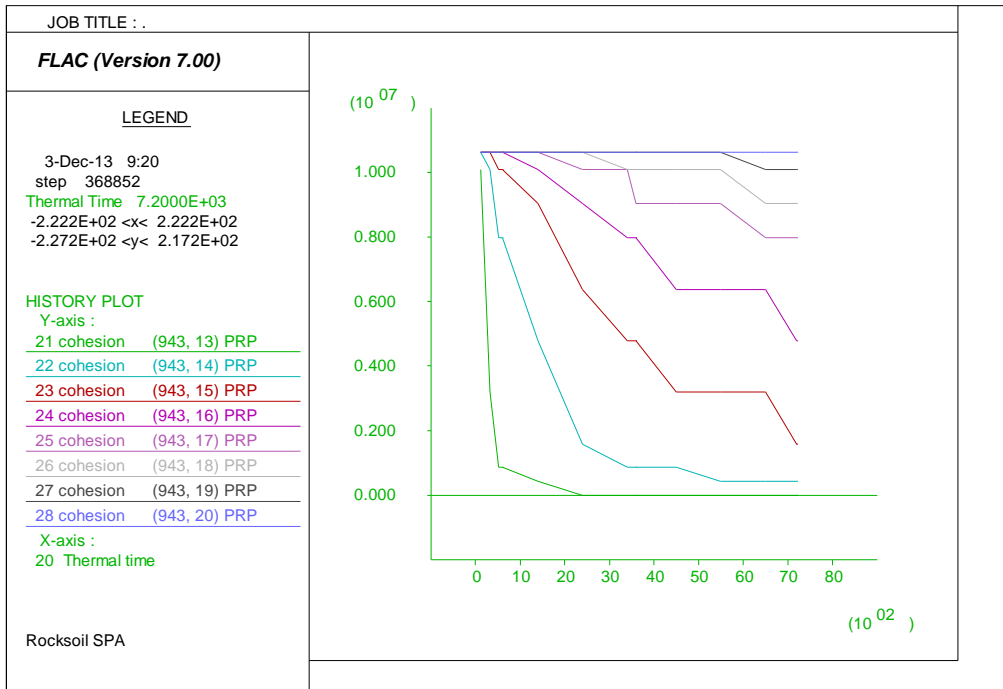
Figura 53 – Evoluzione del valore di coesione c'nel rivestimento – Curva UNI11076
