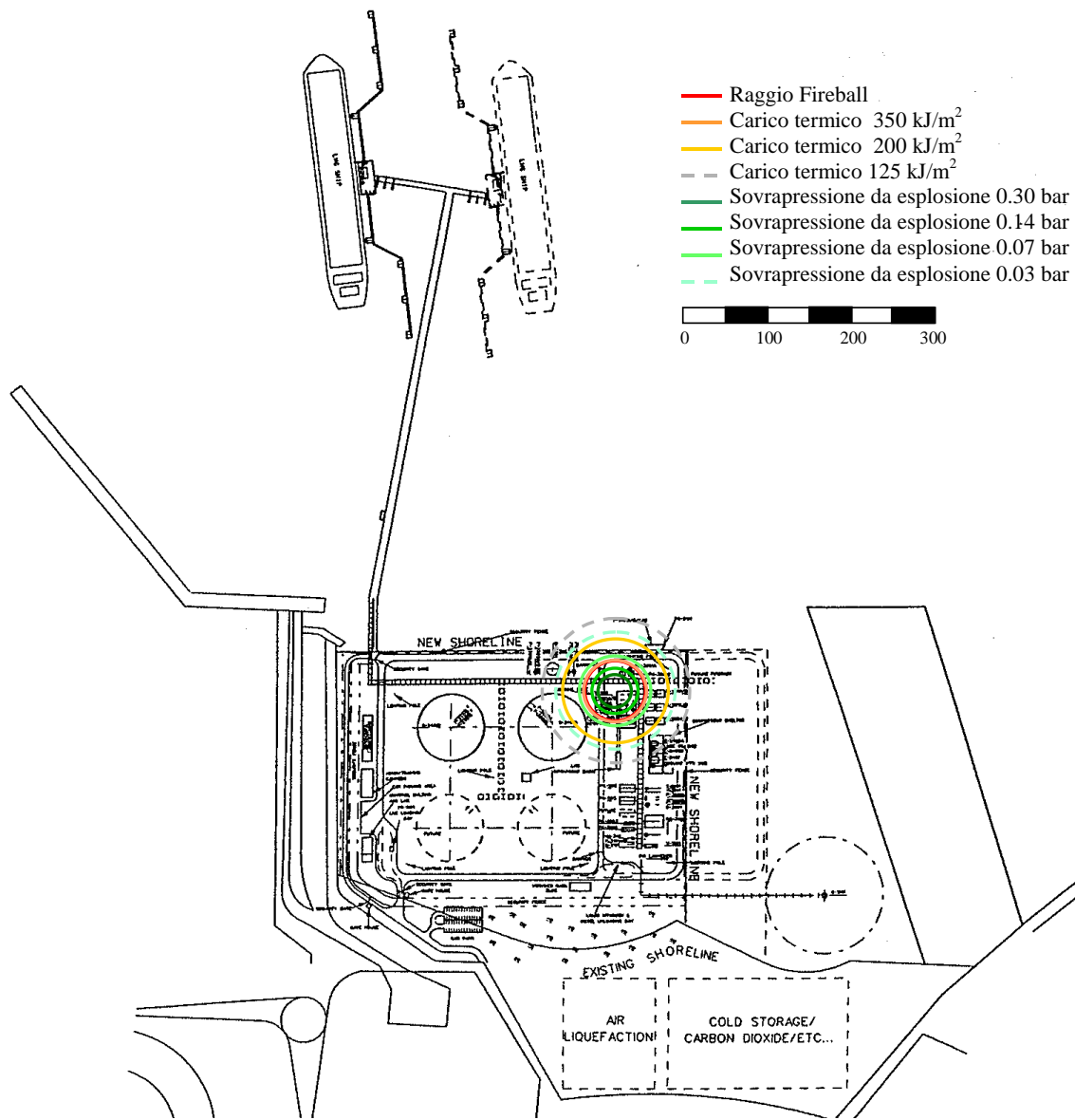
Allegato 1.C.13: Scenario 8 – BLEVE del Serbatoio del Condensatore
