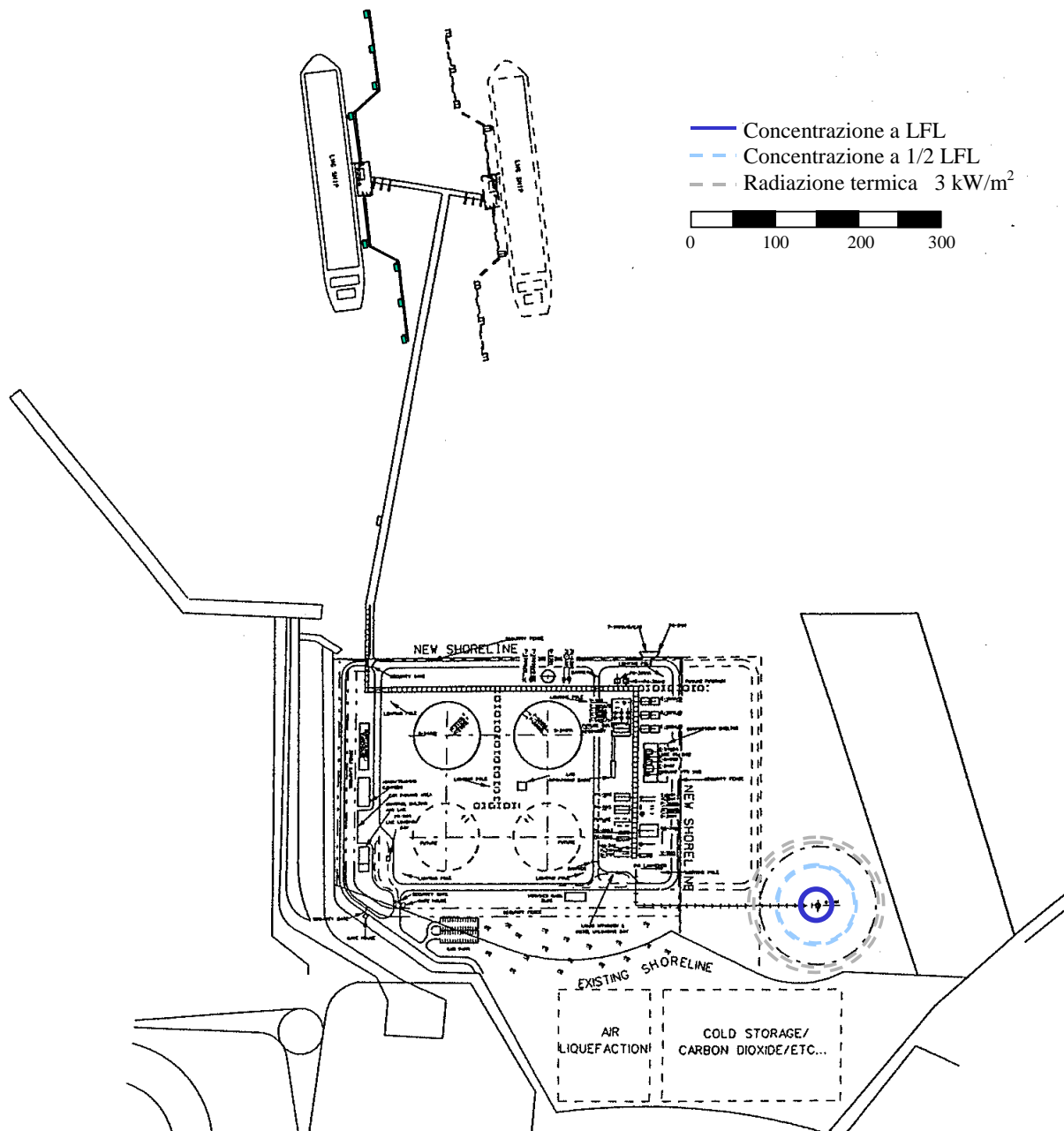
Allegato 1.C.14: Scenario 9 – Rilascio Attraverso la Fiaccola
