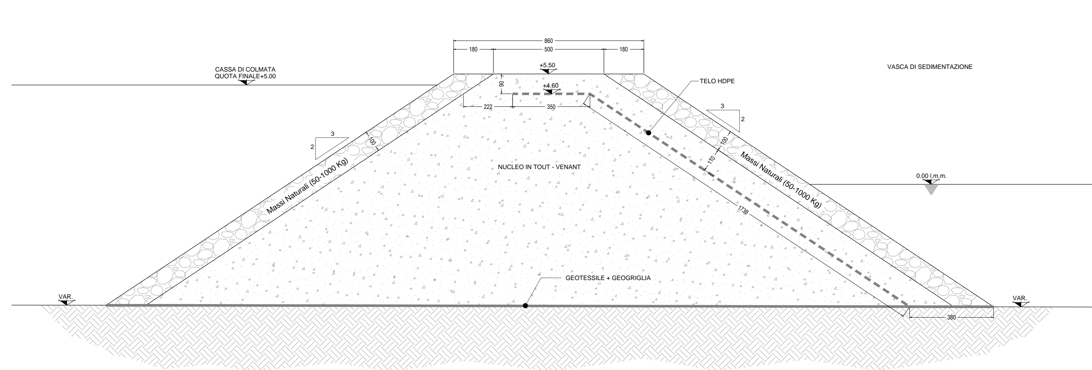
SEZIONE 3-3 - DIGA DI SFIORO SCALA 1:100
