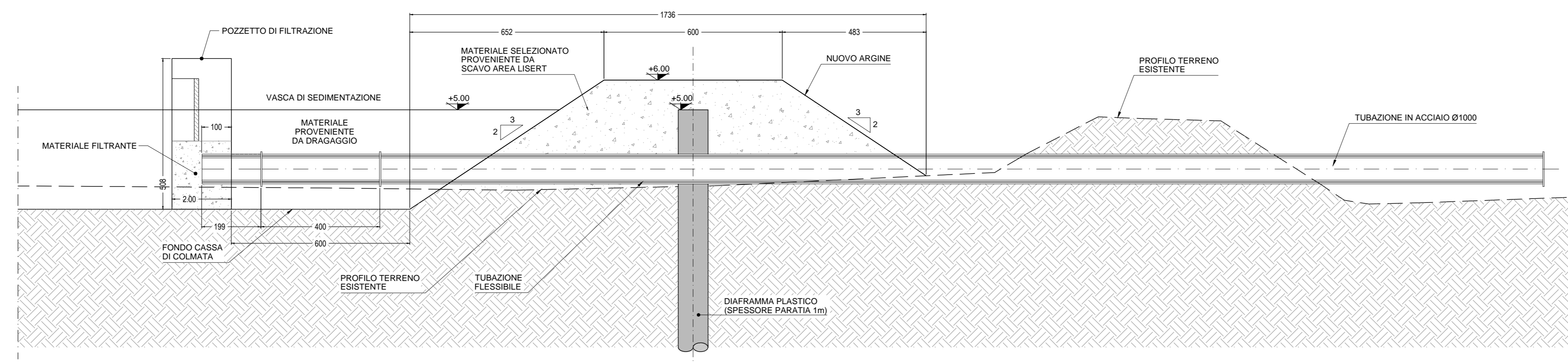
SEZIONE 1-1 - MANUFATTO DI SFIORO SCALA 1:100
