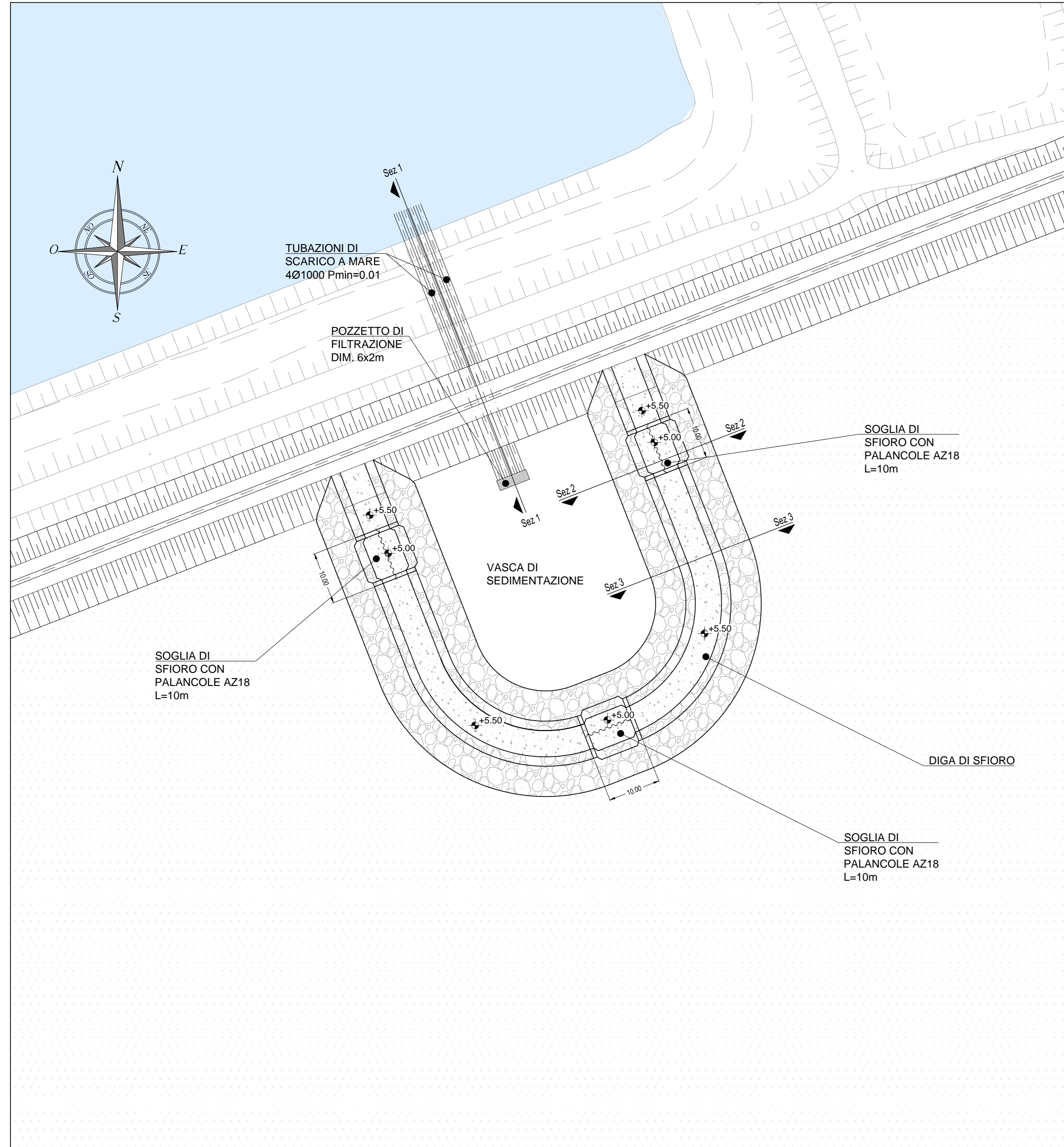
PLANIMETRIA DI PROGETTO SCALA 1:500
