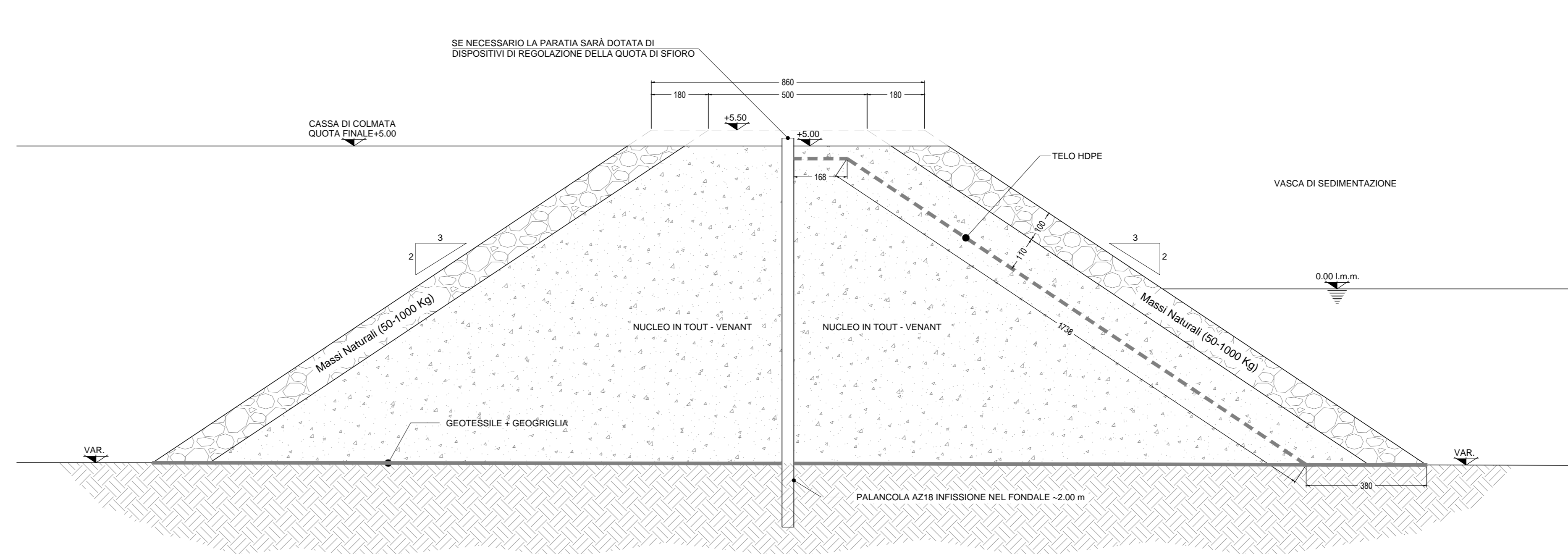
SEZIONE 2-2 - SFIORATORE SCALA 1:100
