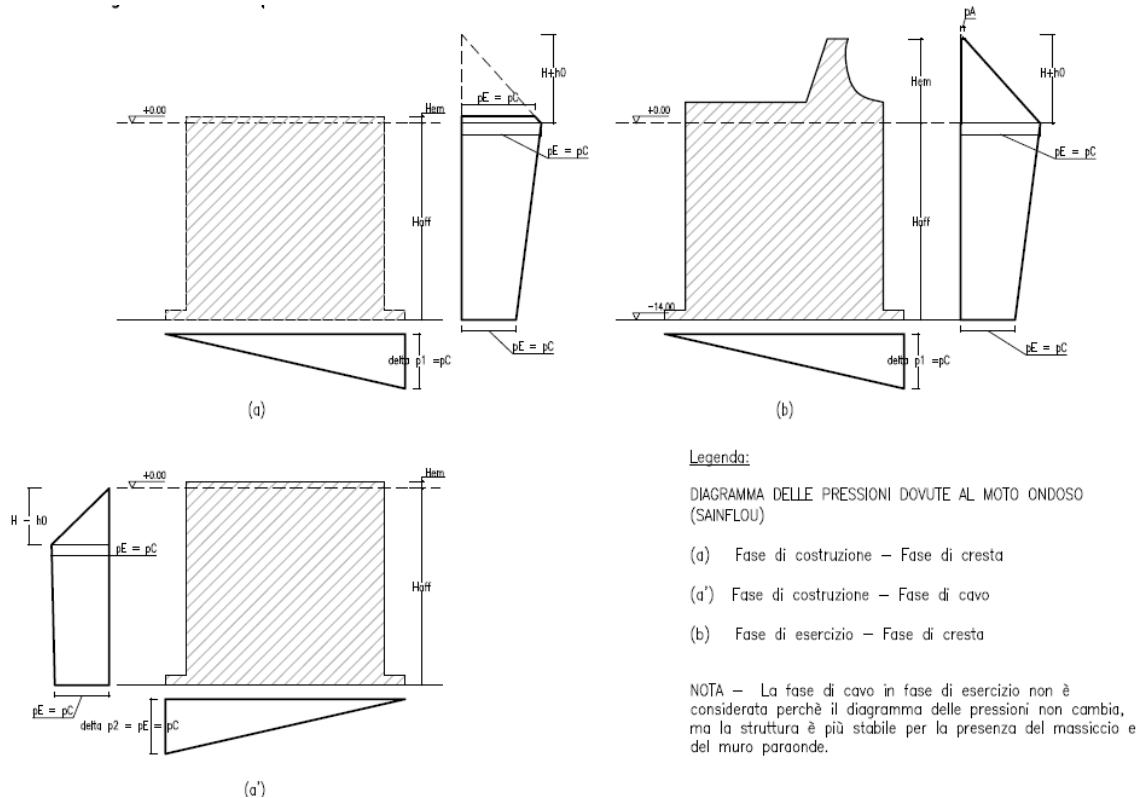
Figura 2- Schematizzazione della spinta secondo Sainflou
