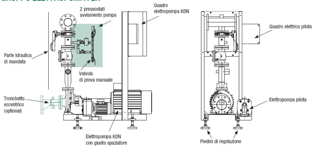
Figura 6 – Schema del gruppo antincendio
