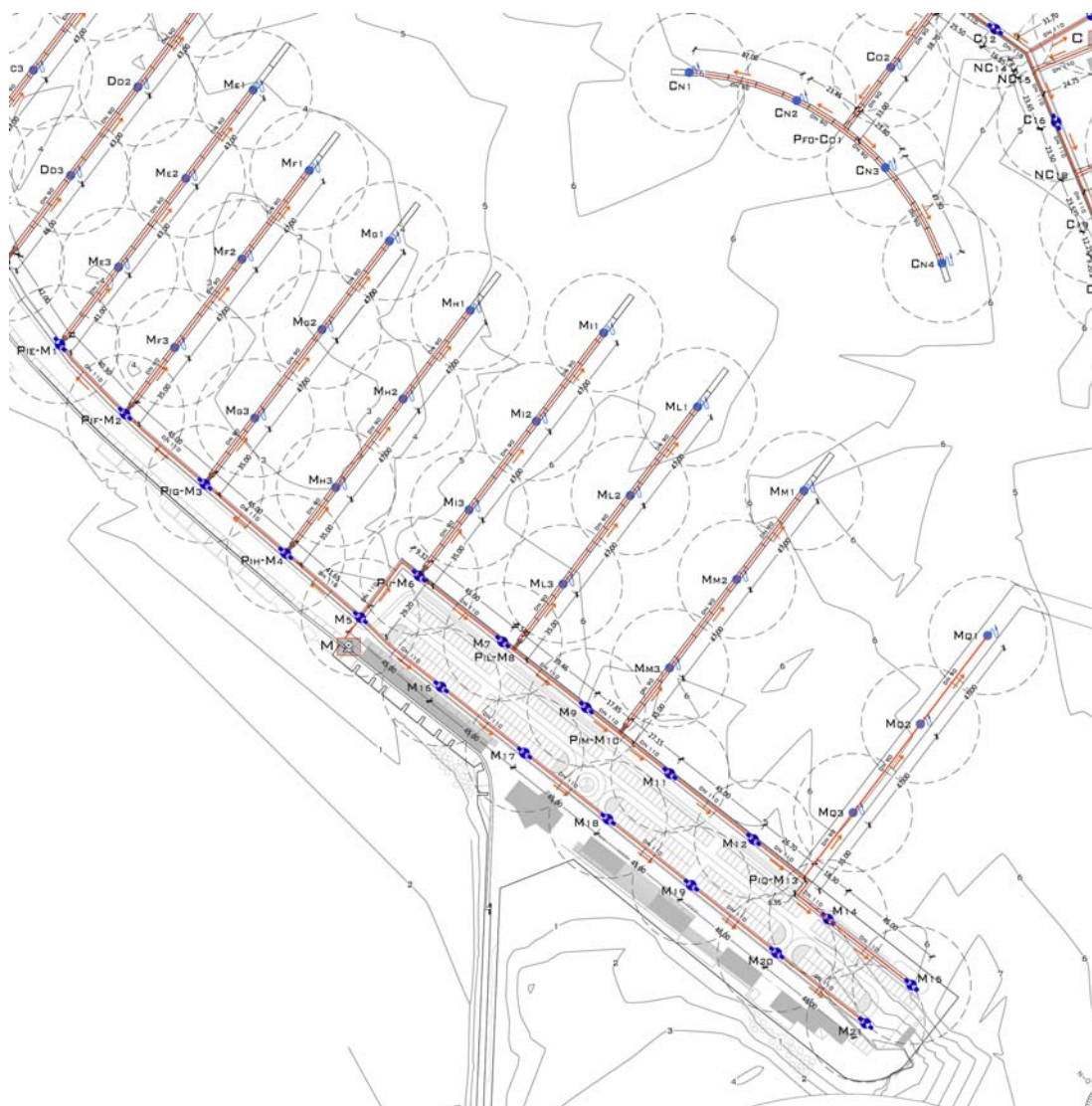
Figura 2 – Rete antincendio blocco M
