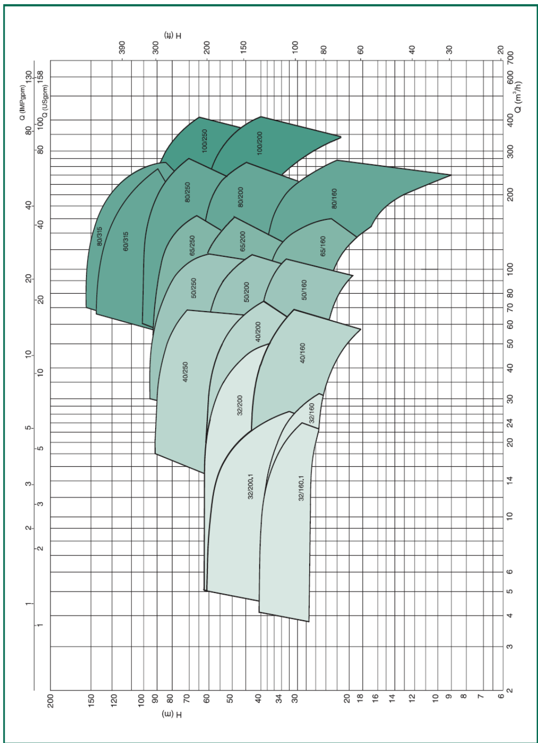
Figura 5 – Tabelle di selezione gruppi di pompe antincendio a NORMA UNI 12845.
