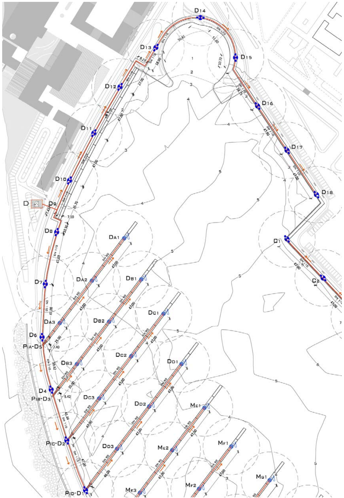
Figura 3 – Rete antincendio blocco D
