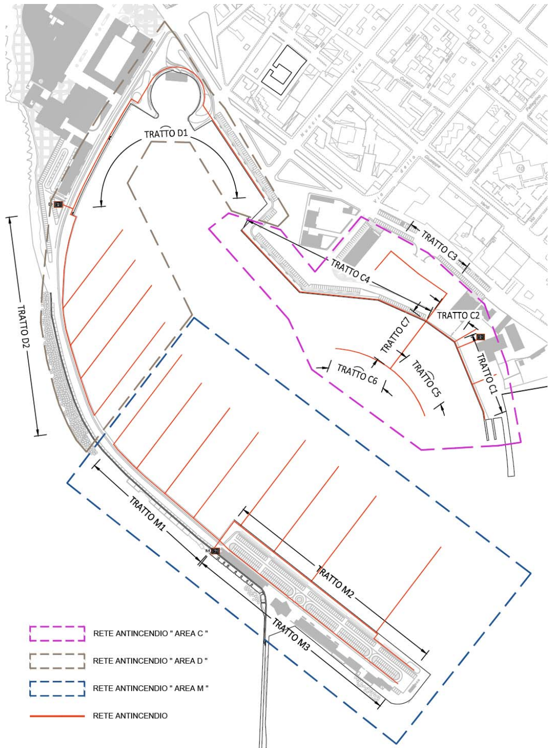
Figura 1 – Distribuzione di insieme rete antincendio
