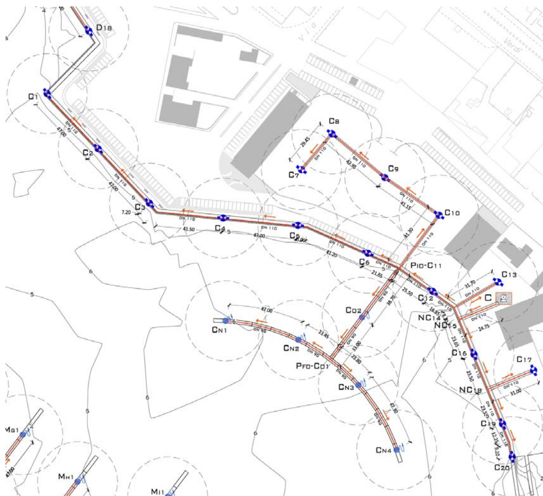
Figura 4 – Rete antincendio blocco C
