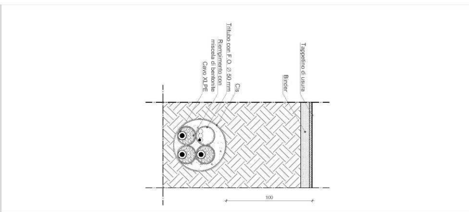
SEZIONE B-B
