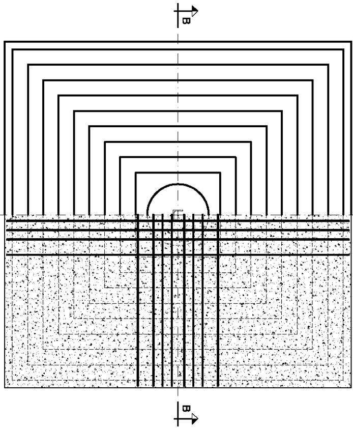
PIANTA - SEZIONE A-A PLINTO FONDAZIONE
