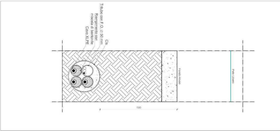
SEZIONE A-A
